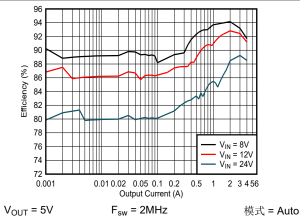
图 8-6. 效率
