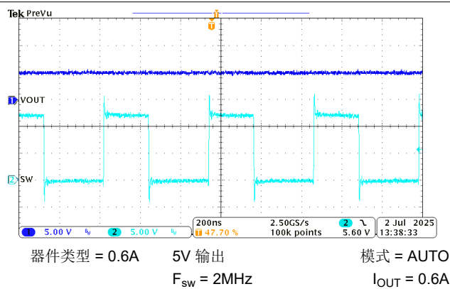
图 8-20. 稳态波形
