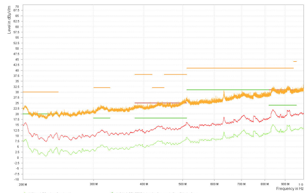
图 8-25. 辐射 EMI 与 CISPR25 限值 (黄色：峰值信号，红色：准峰值信号，绿色：平均信号)、水平双锥天线、LMR60410QEVM
