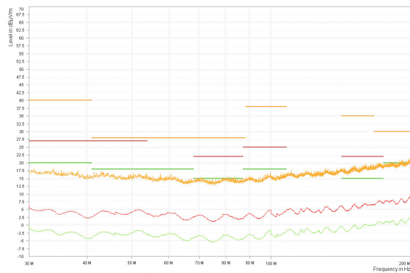
图 8-24. 辐射 EMI 与 CISPR25 限值 (黄色：峰值信号，红色：准峰值信号，绿色：平均信号)、单极天线、LMR60410QEVM
