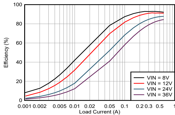
器件类型 = 0.6A 3.3V 输出 模式 = FPWM F_{sw} = 400\text{kHz}
