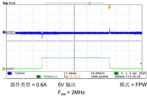
图 8-18. 0A 至 0.6A 负载瞬态
