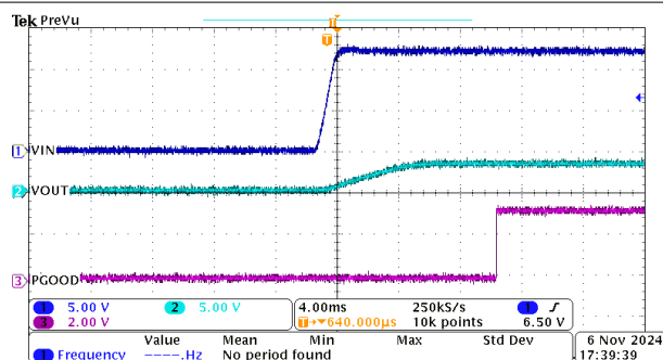
图 8-14. 启动
