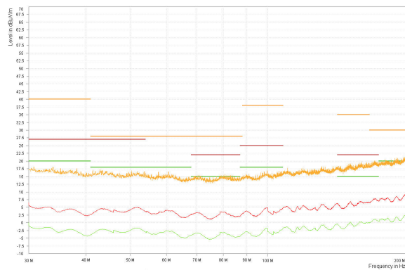
V_{OUT} = 3.3V F_{SW} = 2MHz I_{OUT} = 1A 频率跨度：30MHz 至 200MHz
