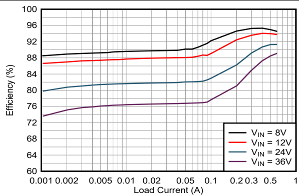
器件类型 = 0.6A 5V 输出 模式 = AUTO F_{sw} = 400kHz
