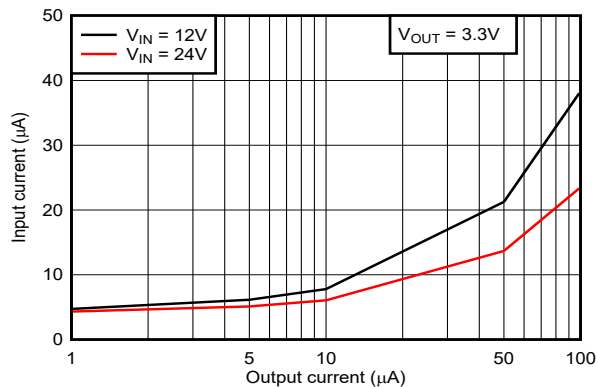
3.3V 固定输出 F_{sw} = 2\text{MHz} 模式 = AUTO
