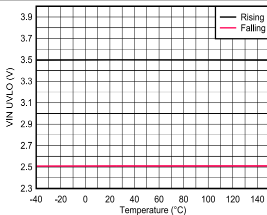
图 6-11. 输入电压 UVLO - B 型号
