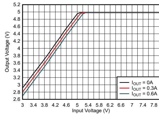
器件类型 = 0.6A 5V 输出 模式 = FPWM F_{sw} = 2\text{MHz}
