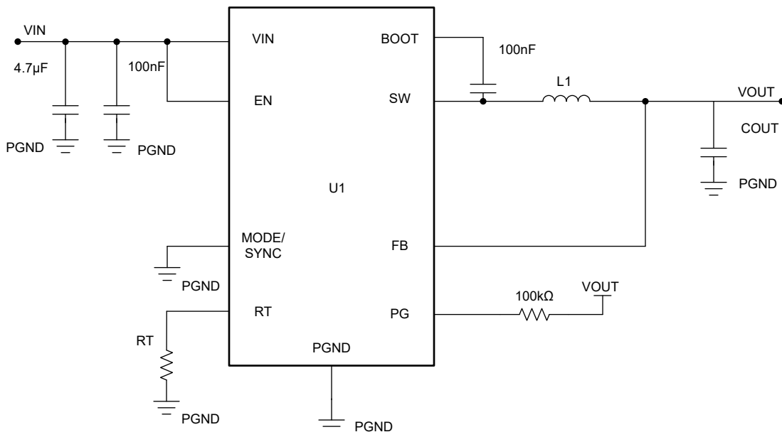
图 8-30. 应用电路示例
