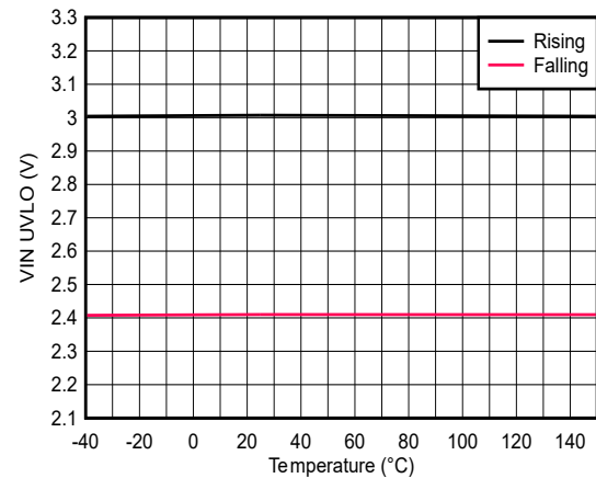
图 6-10. 输入电压 UVLO - A 型号
