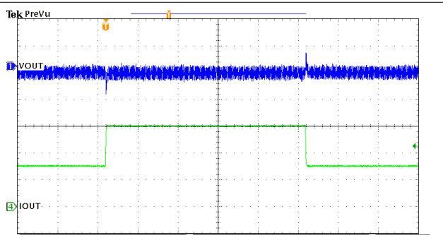
器件类型 = 0.6A 3.3V 输出 模式 = FPWM F_{sw} = 2\text{MHz}
