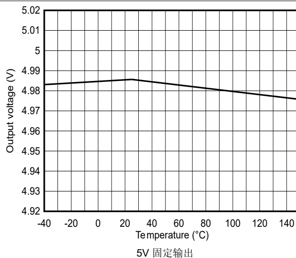
图 6-6. 输出电压精度
