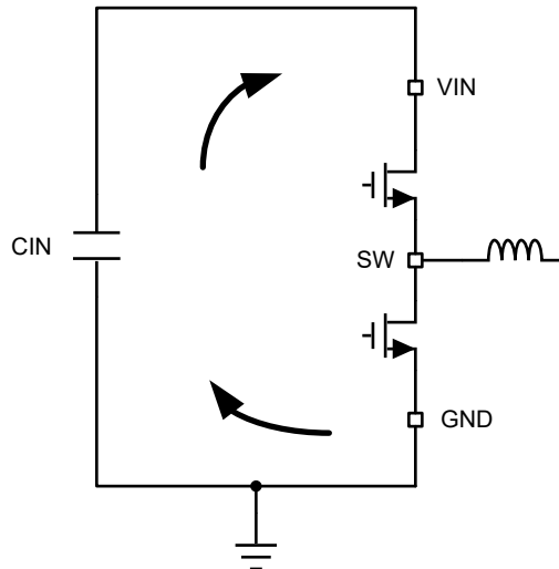
图 8-31. 具有快速瞬变的电流环路
