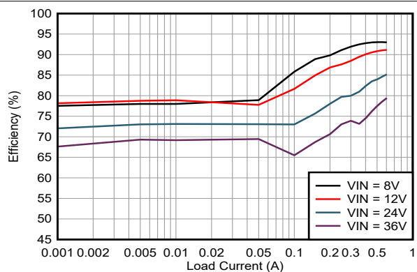
器件类型 = 0.6A 5V 输出 模式 = AUTO F_{sw} = 2MHz
