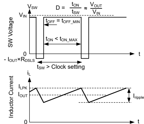
图 7-11. 压降波形
