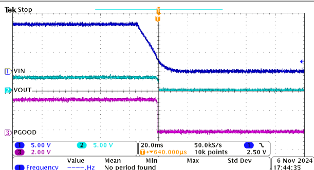
图 8-15. 关断
