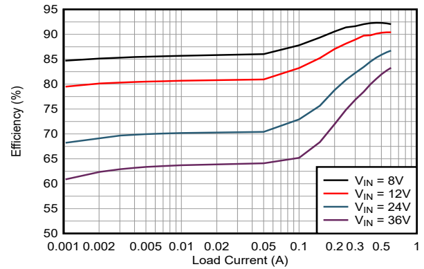
器件类型 = 0.6A 3.3V 输出 模式 = AUTO F_{sw} = 2\text{MHz}
