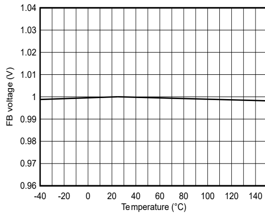
图 6-9. 反馈电压精度
