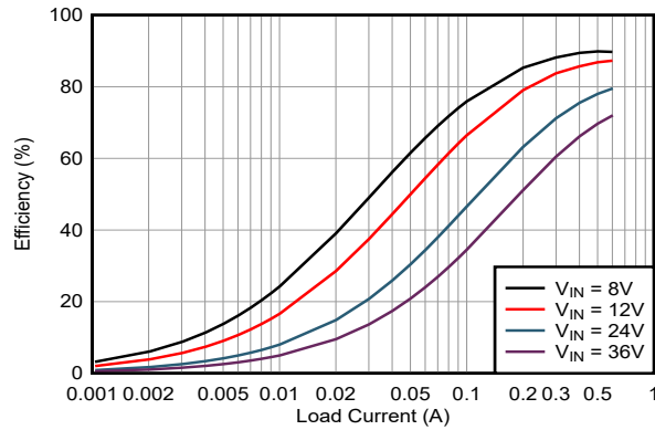
器件类型 = 0.6A 3.3V 输出 模式 = FPWM F_{sw} = 2\text{MHz}
