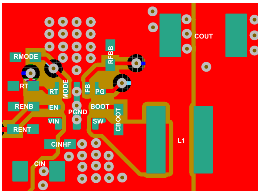
图 8-32. 示例布局
