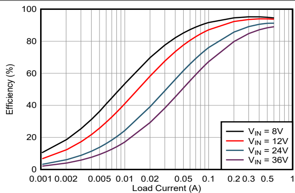
器件类型 = 0.6A 5V 输出 模式 = FPWM F_{sw} = 400kHz
