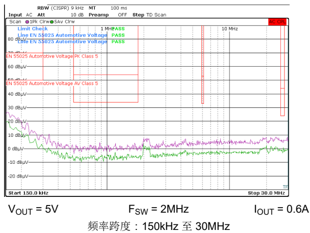
图 8-22. 传导 EMI 与 CISPR25 限值 (紫色: 峰值信号, 绿色: 平均信号), LMR60410QEVM
