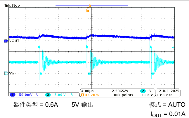
图 8-21. 稳态波形
