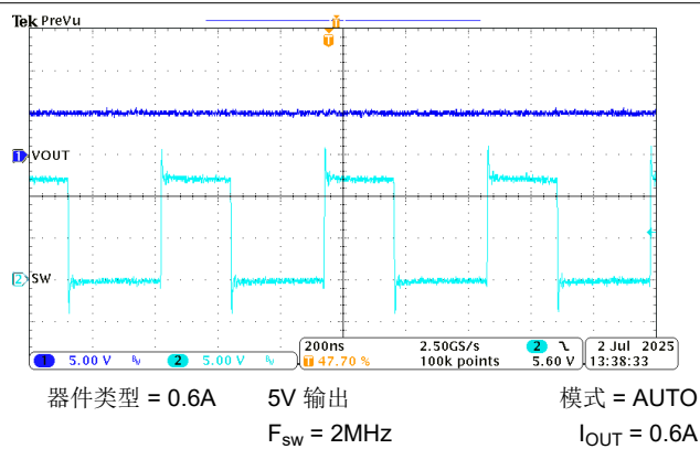
图 8-20. 稳态波形
