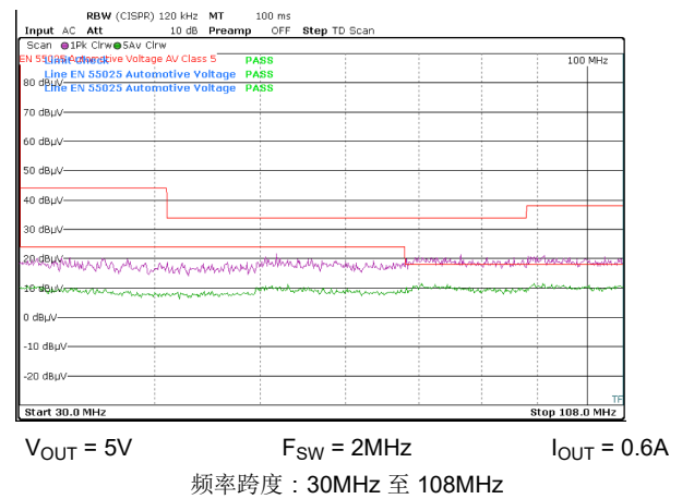
图 8-23. 传导 EMI 与 CISPR25 限值 (紫色: 峰值信号, 绿色: 平均信号), LMR60410QEVM
