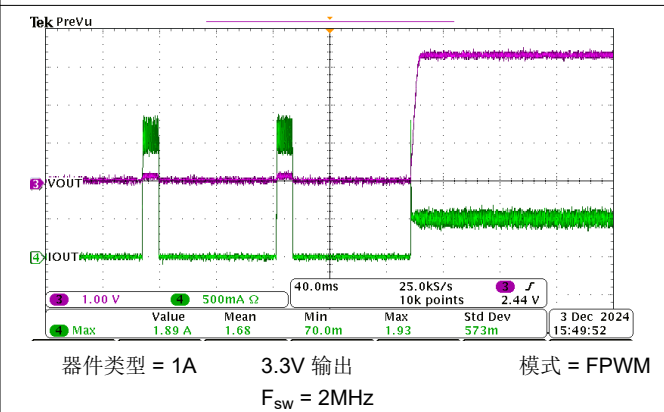
图 8-23. 短路恢复
