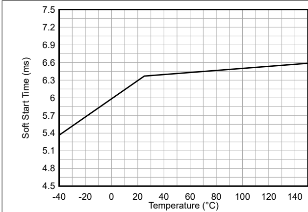
图 6-7. 软启动时间
