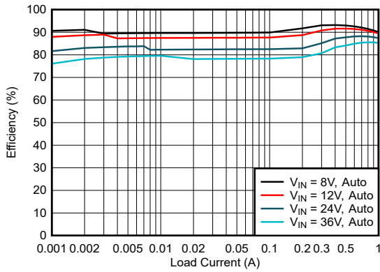
器件类型 = 1A 3.3V 输出 模式 = AUTO F sw = 400kHz
