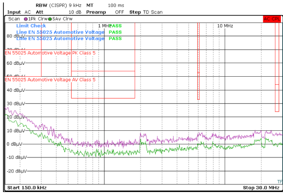
V_{OUT} = 5V F_{SW} = 2MHz I_{OUT} = 1A 频率跨度：150kHz 至 30MHz
