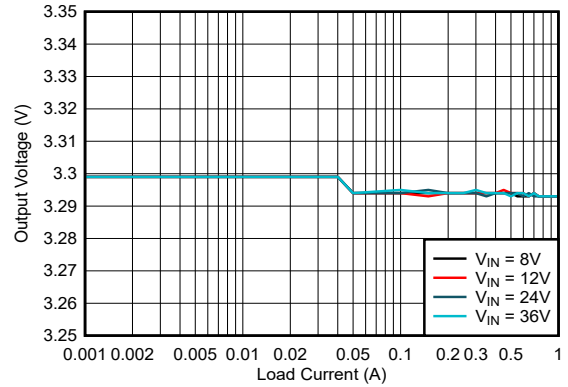
器件类型 = 1A 3.3V 输出 模式 = FPWM F sw = 2MHz
