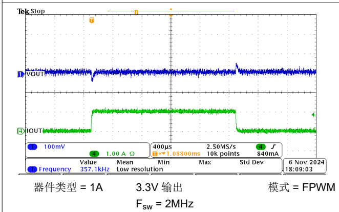
图 8-20. 0A 至 1A 负载瞬态
