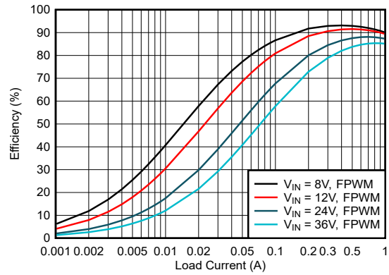
器件类型 = 1A 3.3V 输出 模式 = FPWM F sw = 400kHz
