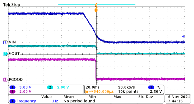
器件类型 = 1A 3.3V 输出 模式 = FPWM F sw = 2MHz
