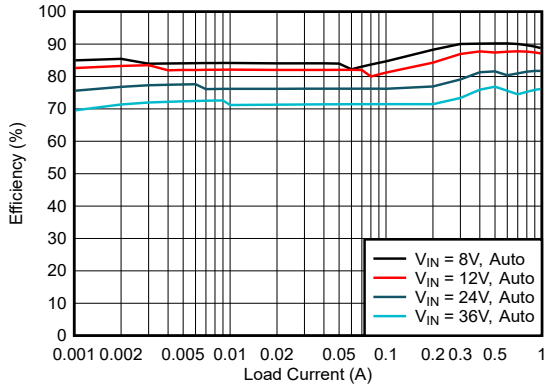
器件类型 = 1A 3.3V 输出 模式 = AUTO F sw = 2MHz
