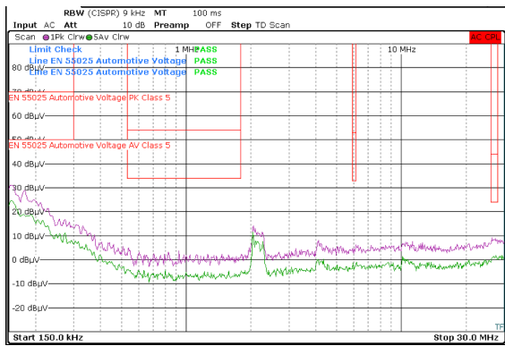
V_{OUT} = 3.3V F_{SW} = 2MHz I_{OUT} = 1A 频率跨度：150kHz 至 30MHz
