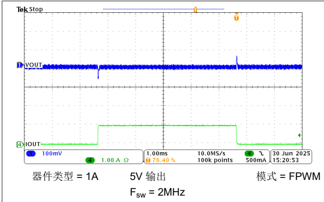
图 8-18. 0A 至 1A 负载瞬态
