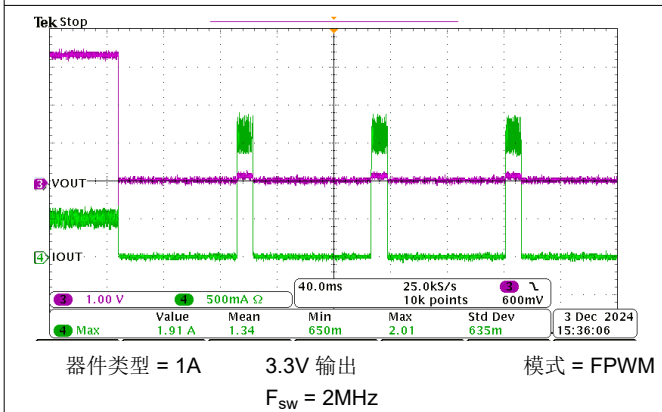
图 8-22. 应用短路
