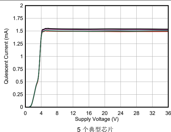
图 5-25. 静态电流与电源电压间的关系
