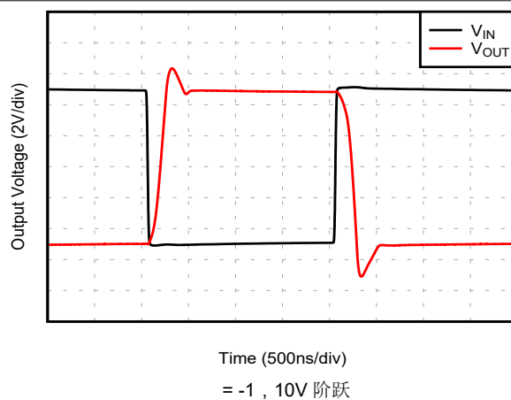
图 5-36. 大信号阶跃响应
