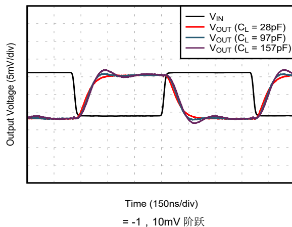
图 5-34. 小信号阶跃响应
