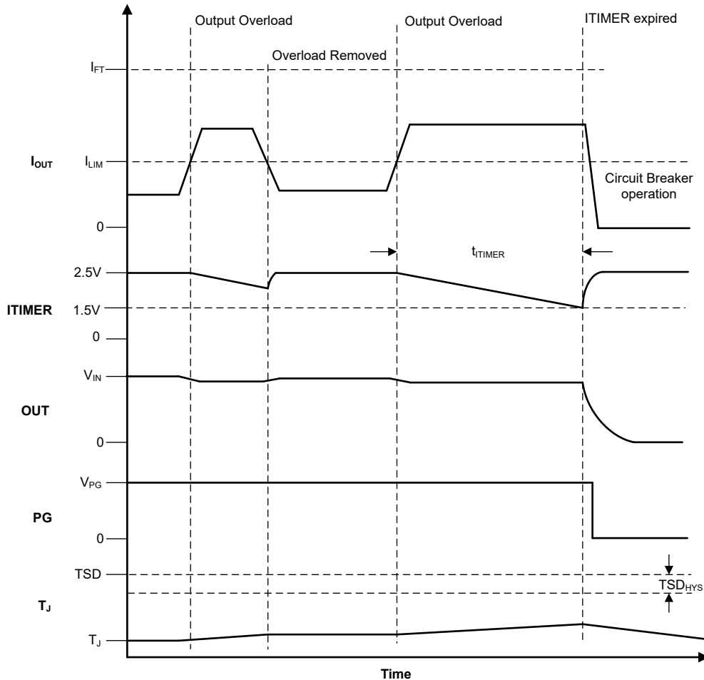
图 7-4. 断路器响应
