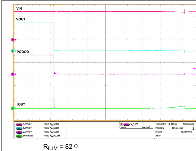
图 8-7. 导通时输出硬短路
