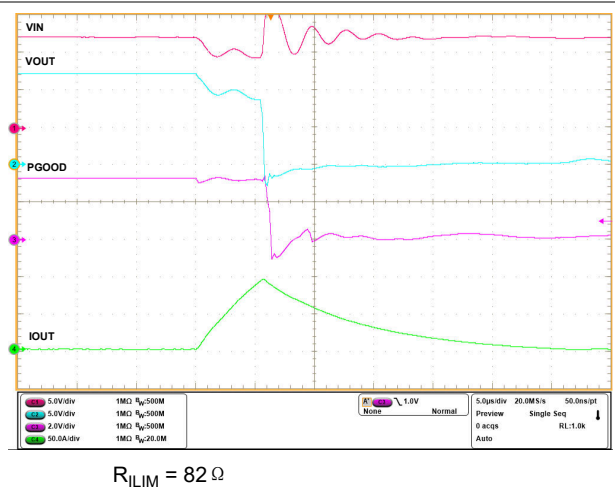
图 8-8. 导通时输出硬短路 (放大图)
