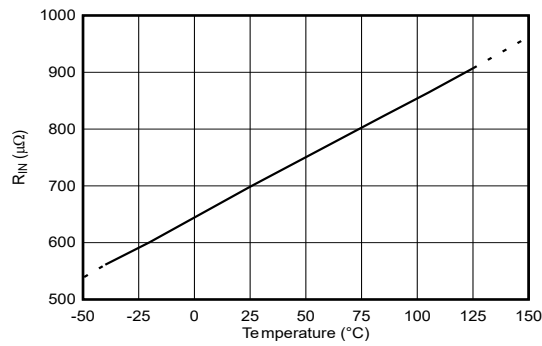
图 6-23. 输入导体电阻与温度间的关系
