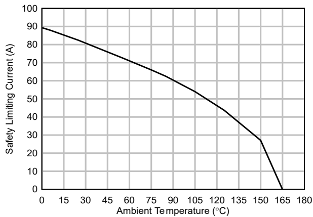
图 6-24. 安全限制电流的热降额曲线，侧 1
