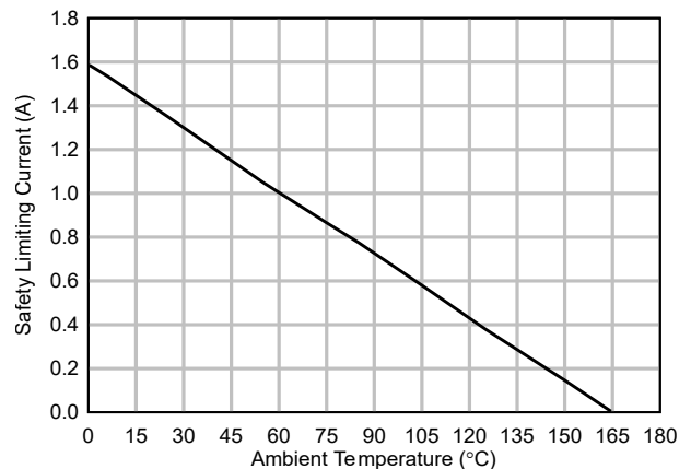
图 6-25. 安全限制电流的热降额曲线，侧 2
