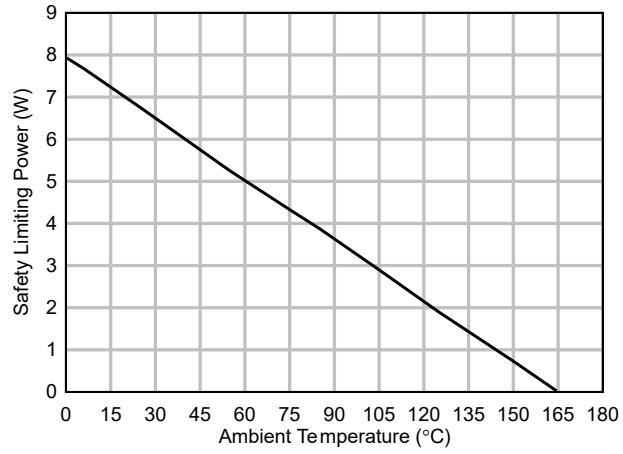
图 6-26. 安全限制功率的热降额曲线
