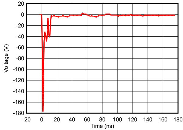
图 5-13. -8kV 钳位 IEC 波形 (DPY)
