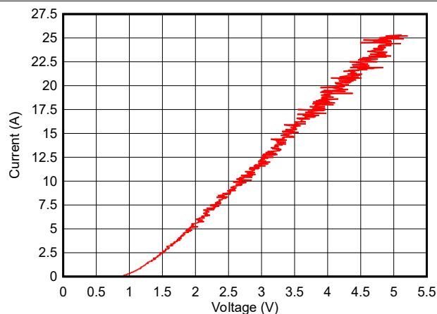
图 5-11. 负 TLP 曲线 (DPY)
