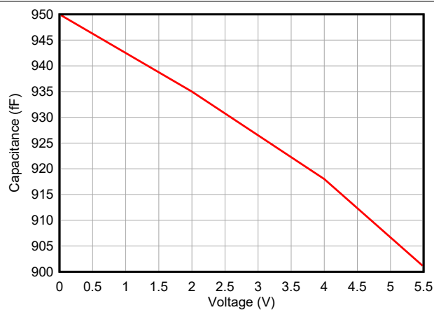
图 5-5. 偏置电压与电容间的关系 (DPL)
