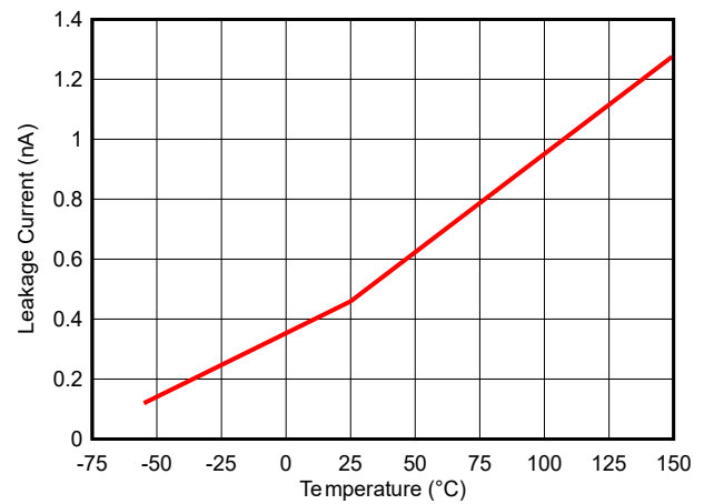
图 5-16. 温度与漏电流间的关系 (DPY)
