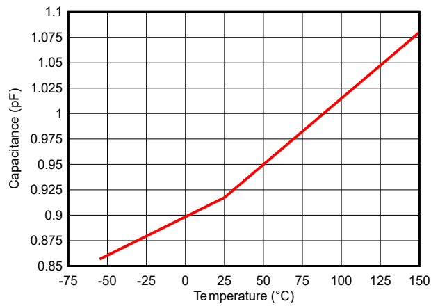
图 5-15. 温度与电容间的关系 (DPY)
