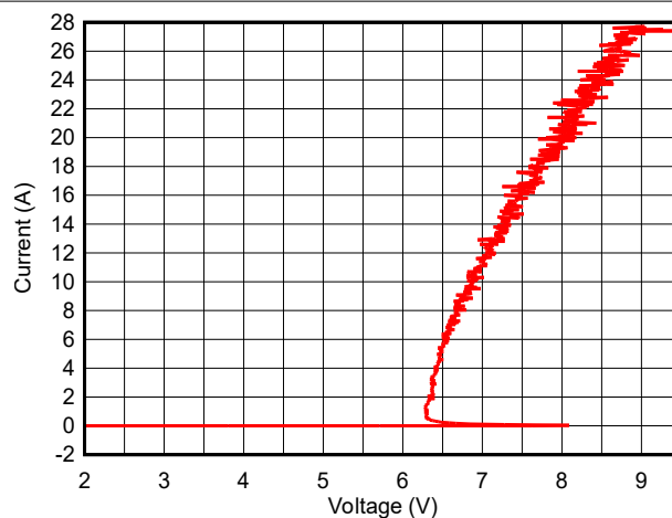
图 5-10. 正 TLP 曲线 (DPY)
