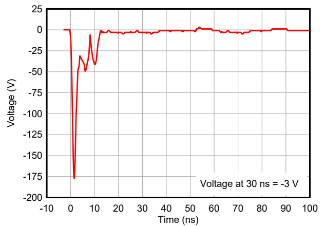
图 5-4. -8kV 钳位 IEC 波形 (DPL)
