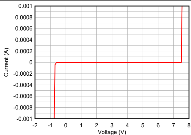
图 5-9. 直流 I-V 曲线 (DPL)
