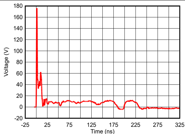
图 5-12. +8kV 钳位 IEC 波形 (DPY)
