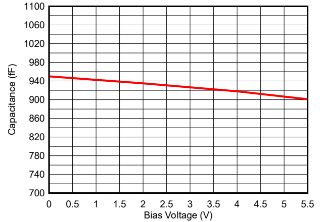
图 5-14. 偏置电压与电容间的关系 (DPY)
