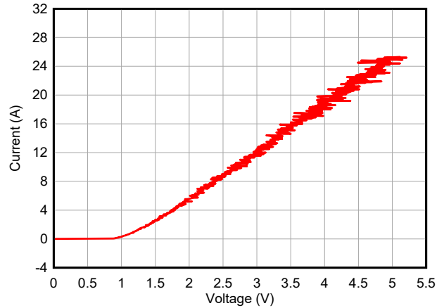
图 5-2. 负 TLP 曲线 (DPL)
