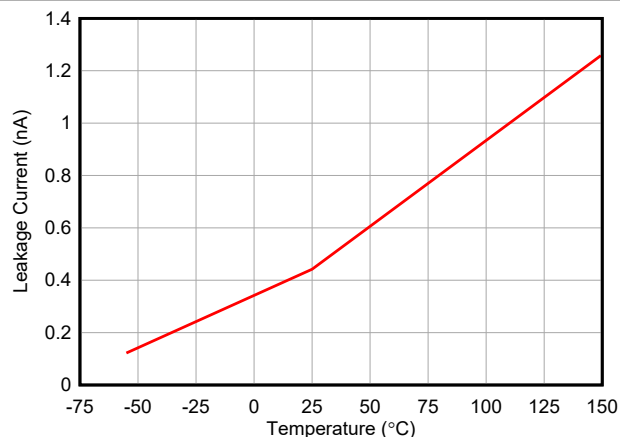
图 5-7. 温度与漏电流间的关系 (DPL)
