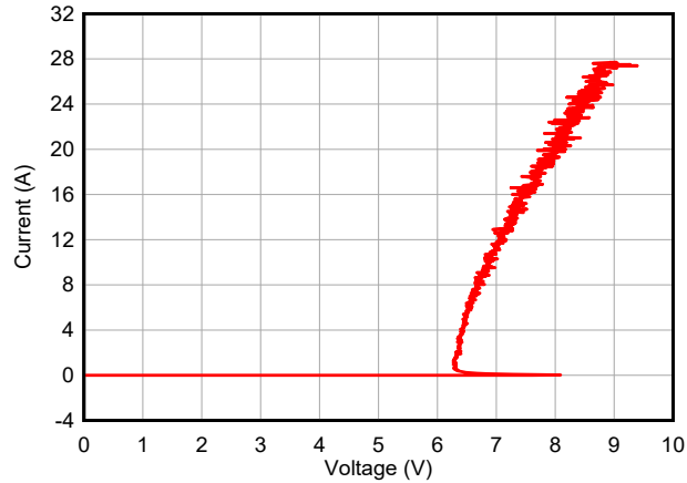
图 5-1. 正 TLP 曲线 (DPL)
