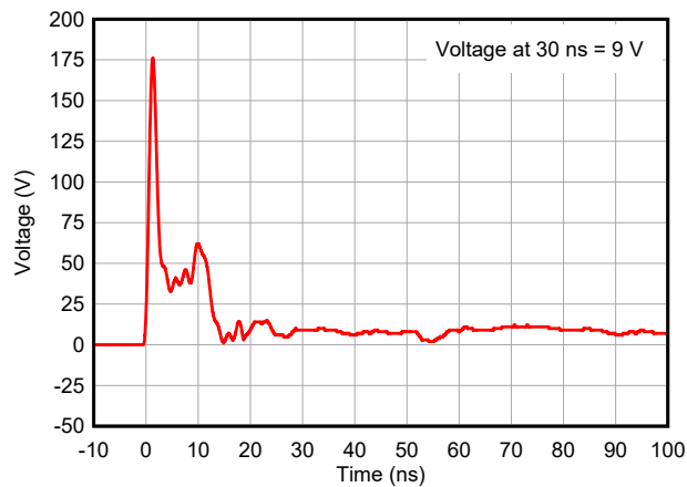
图 5-3. +8kV 钳位 IEC 波形 (DPL)
