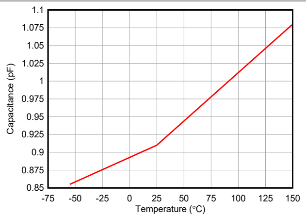
图 5-6. 温度与电容间的关系 (DPL)
