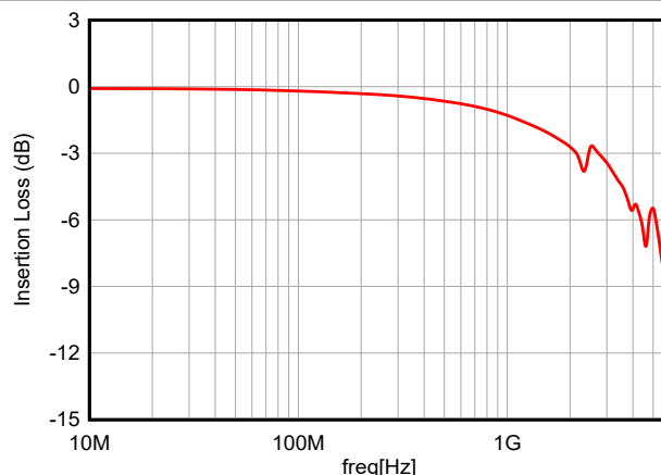
图 5-8. 插入损耗 (DPL)
