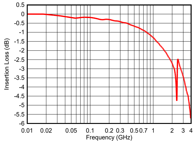
图 5-17. 插入损耗 (DPY)
