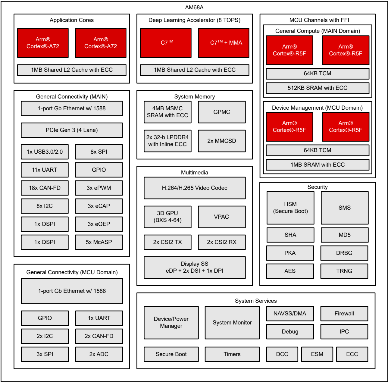
图 3-1. 功能方框图
