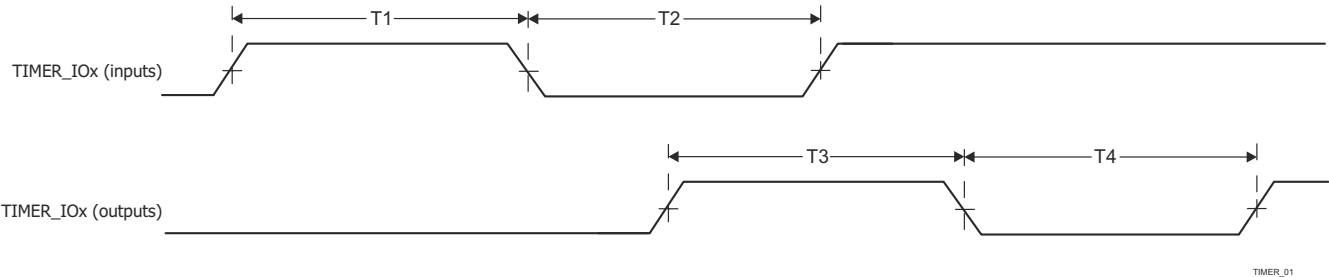
图 6-114. 计时器时序
