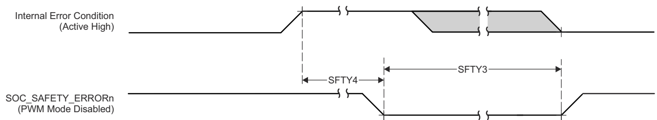
图 6-22. SOC_SAFETY_ERRORn 开关特性
