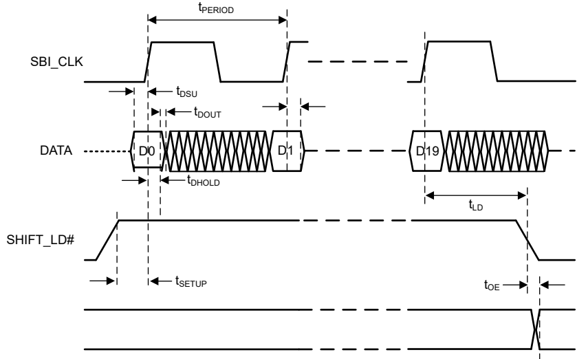
图 6-2. SBI 时序图
