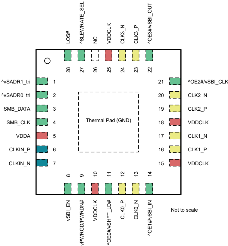
图 5-5. LMKDB1104 和 LMKDB1104FS 4mm x 4mm VQFN 封装 28 引脚 顶视图
