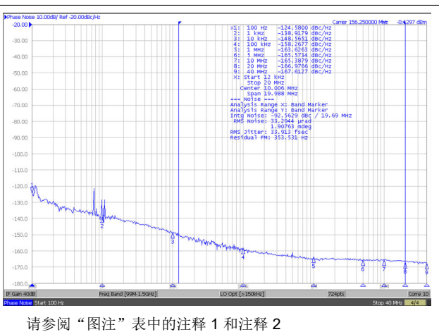
图 10-3. 156.25\text{MHz} 下的 LMKDB11xx/120x 相位噪声/输出抖动 ( 12\text{kHz} - 20\text{MHz} )
