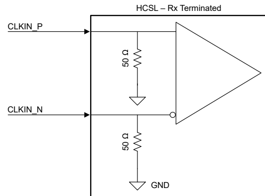
图 8-6. 接收器内部终端
