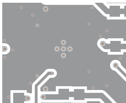
图 10-13. LMKDB1202 布局示例 - 底层
