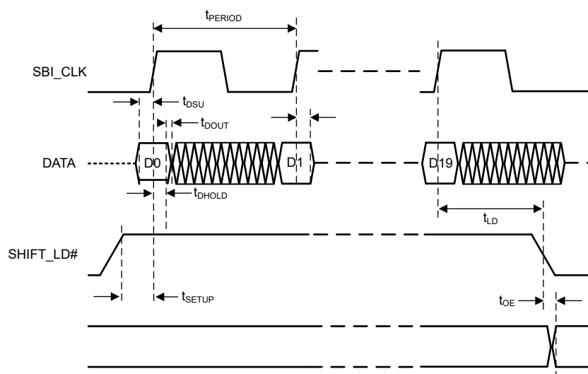
图 6-2. SBI 时序图
