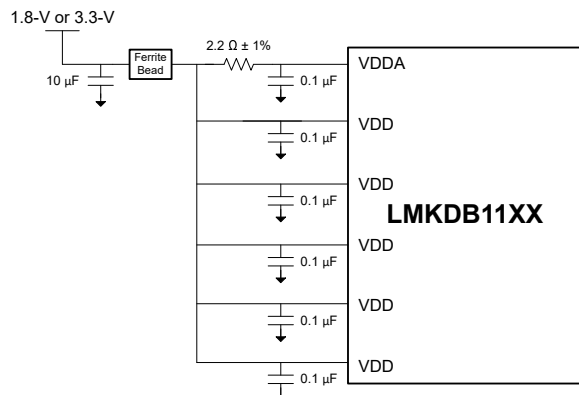
图 10-4. LMKDB11XX 缓冲器的电源建议
