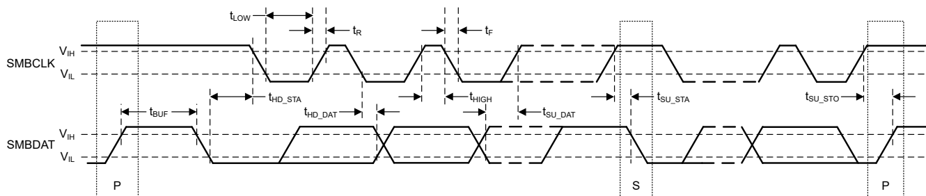
图 6-1. SMBus 时序图
