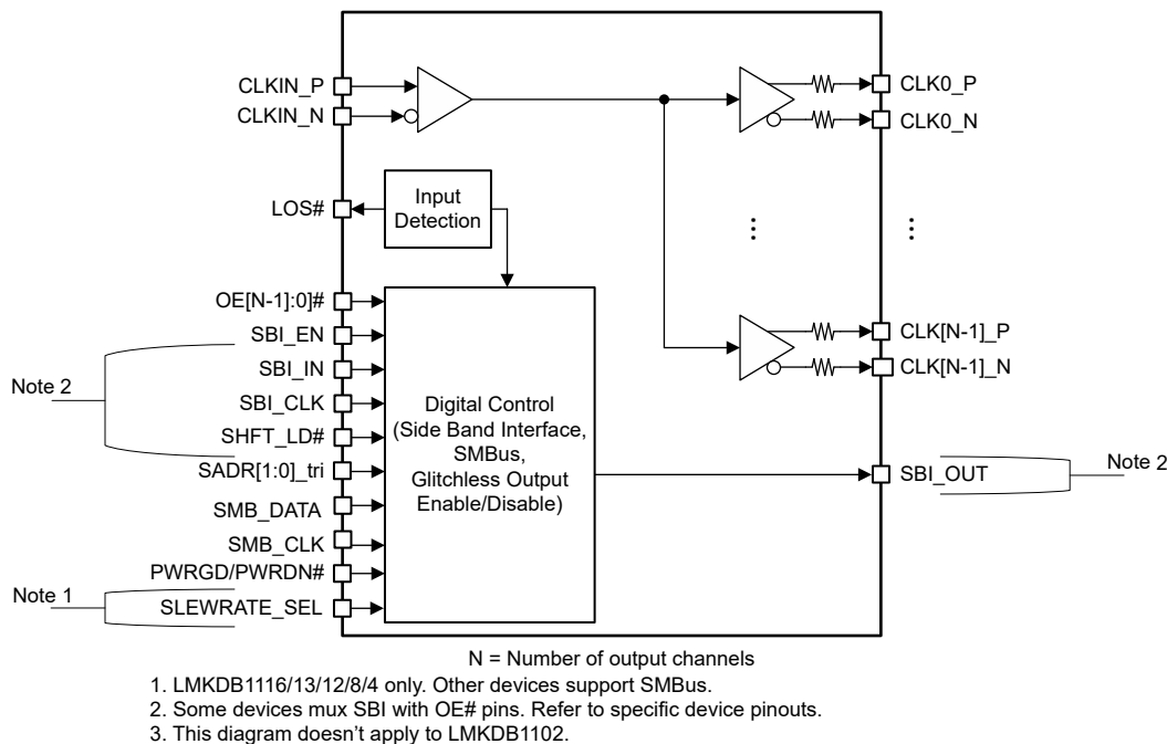
图 8-1. LMKDB11xx 功能方框图
