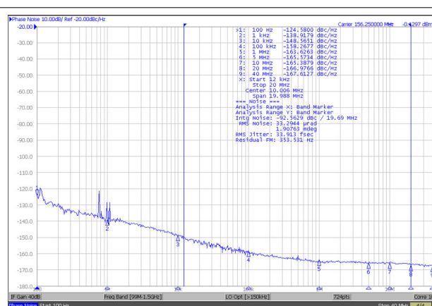
图 6-4. 156.25MHz 下的 LMKDB11xx 相位噪声/输出抖动 (12kHz - 20MHz)
