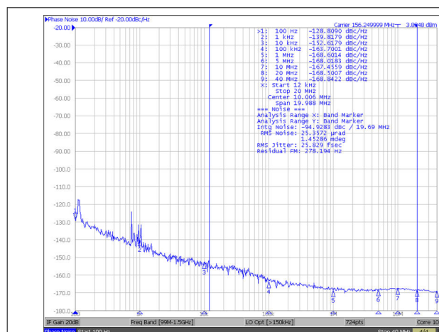
图 6-3. 156.25MHz 下的输入源 (12kHz - 20MHz)
