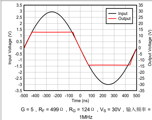
图 6-27. 过驱恢复
