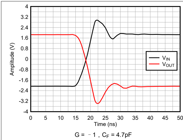
图 6-25. 趋稳时间
