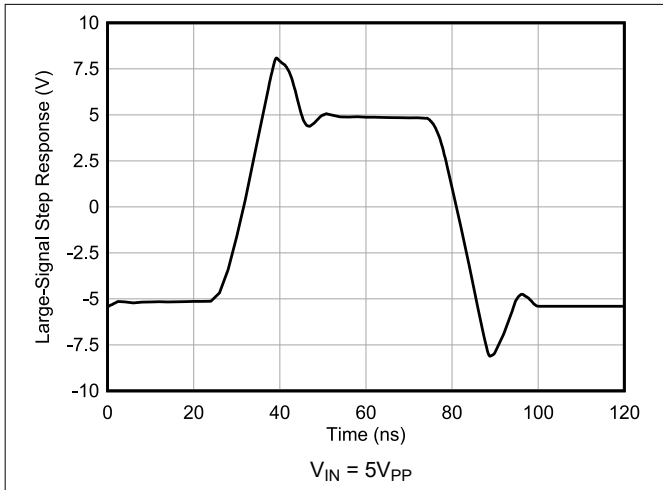
图 6-21. 大信号瞬态响应
