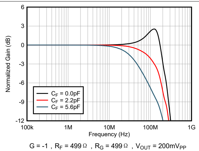
图 6-4. 小信号频率响应
