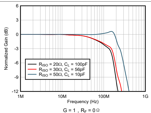
图 6-6. 频率响应与容性负载间的关系
