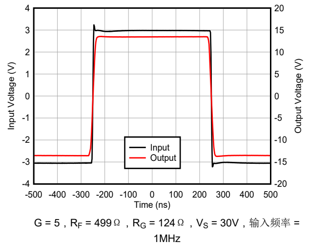
图 6-28. 过驱恢复
