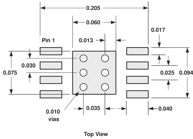
图 8-14. DGN PowerPAD™ 集成电路封装 PCB 蚀刻和过孔布局
