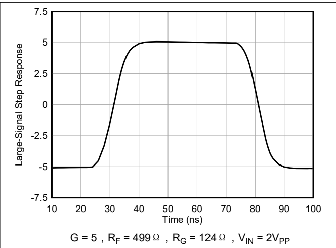
图 6-22. 大信号瞬态响应
