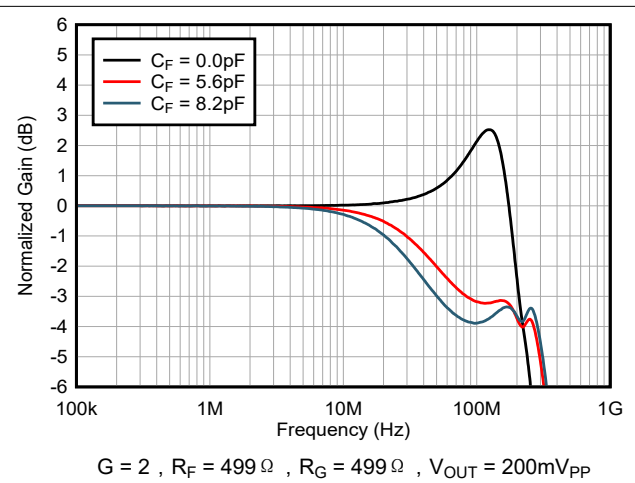
图 6-2. 小信号频率响应
