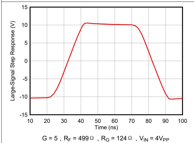
图 6-23. 大信号瞬态响应
