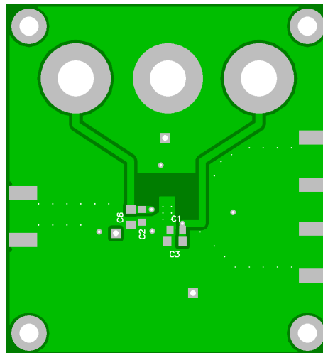
图 9-3. EVM 底层
