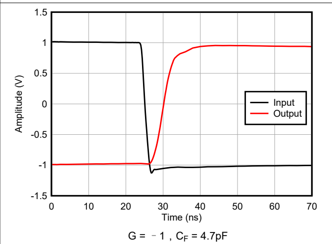
图 6-24. 趋稳时间
