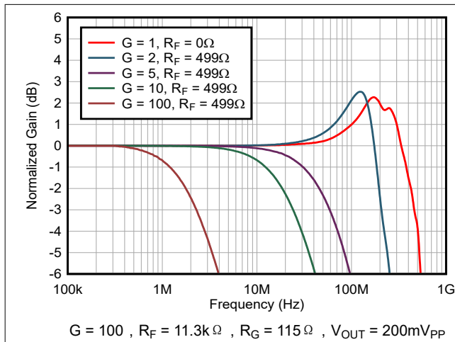
图 6-1. 小信号频率响应
