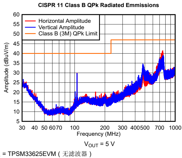
图 8-21. CISPR 11 RE, 3 米, 扫描 30MHz 至 1GHz
