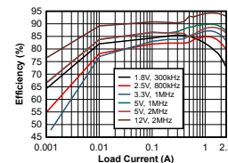
效率与输出电流间的关系 V_{IN} = 24V
