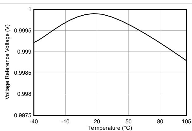
图 6-2. 反馈电压 ( V_{FB} ) 精度与温度间的关系
