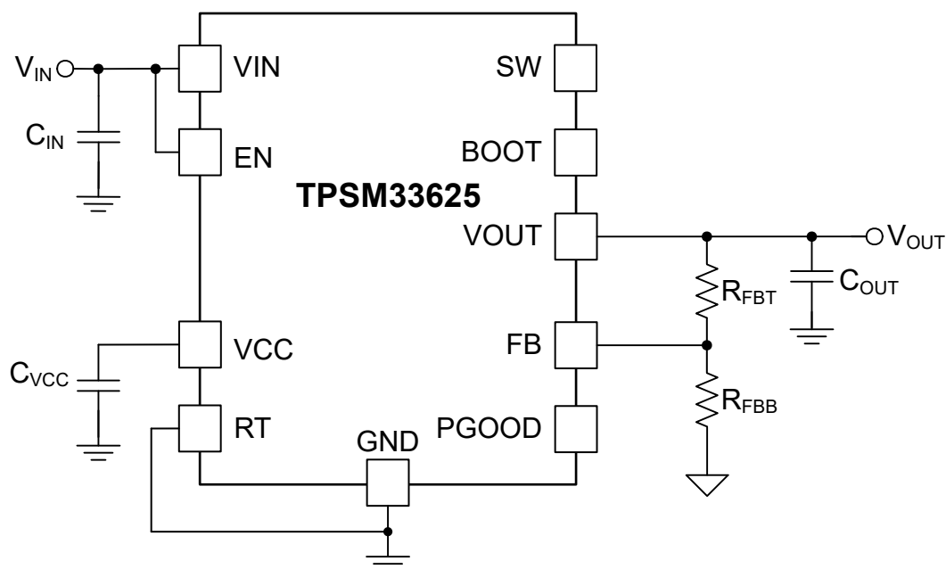
典型电路原理图
