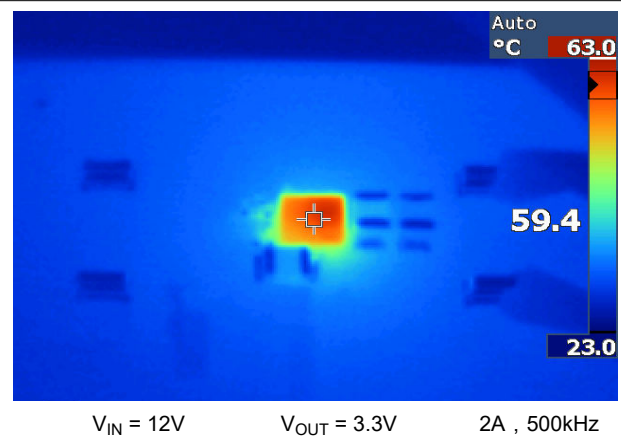
图 8-14. EVM 热性能
