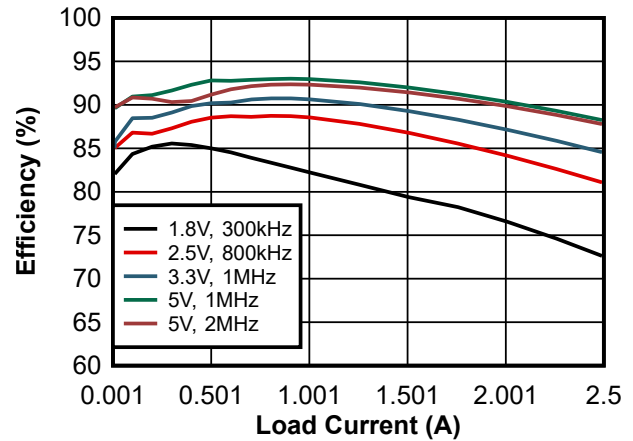
图 8-4. 12VIN 效率 (线性)
