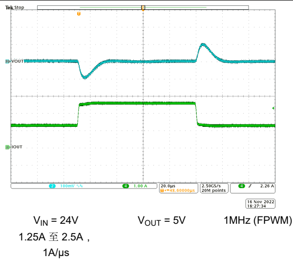
图 8-13. 负载瞬态
