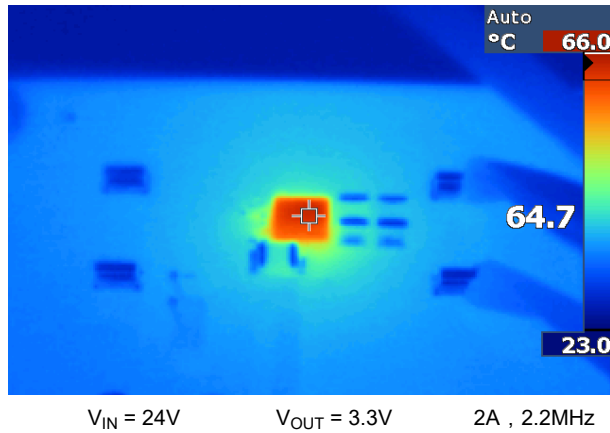
图 8-19. EVM 热性能
