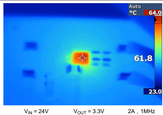
图 8-18. EVM 热性能
