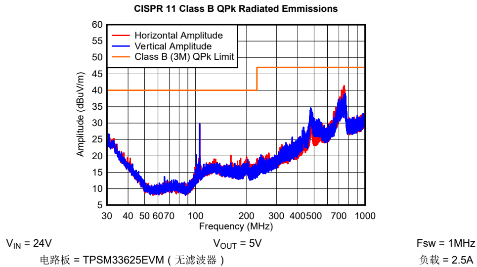
图 8-21. CISPR 11 RE, 3 米, 扫描 30MHz 至 1GHz
