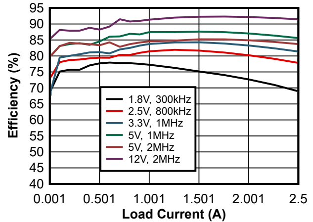
图 8-10. 36VIN 效率 (线性)
