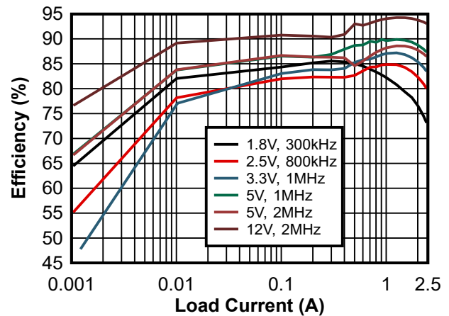
图 8-6. 24VIN 效率 (对数)
