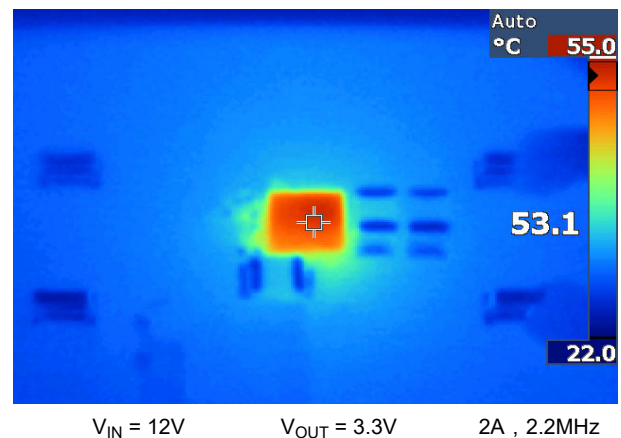
图 8-16. EVM 热性能
