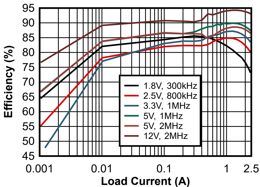
效率与输出电流间的关系 V_{IN} = 24V
