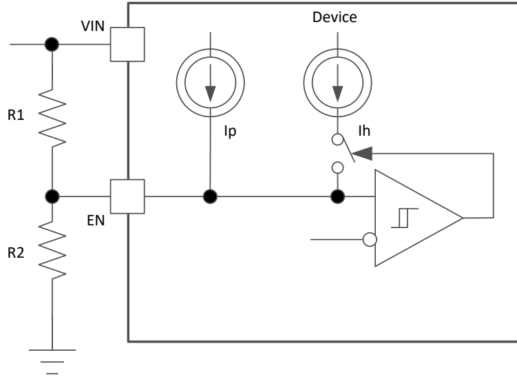
图 6-6. 可调节 V_{IN} 欠压锁定
