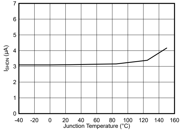
图 5-2. TPS54538 关断电流与结温间的关系
