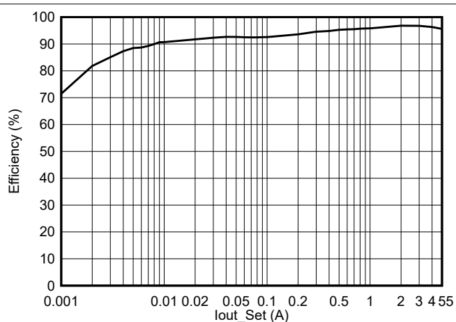
图 5-16. TPS54538 效率 (PFM), V_{IN} = 24\text{V} 、 V_{OUT} = 12\text{V} 、 f_{SW} = 500\text{kHz} 、 L = 5.6\mu\text{H}
