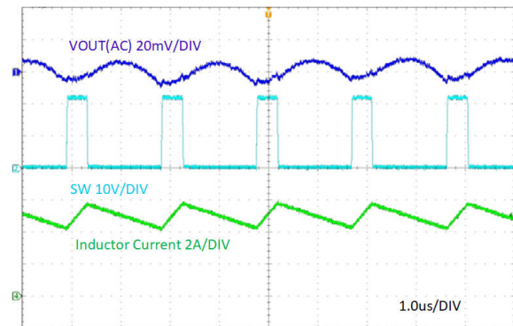
图 7-13. 稳态, I_{OUT} = 5A
