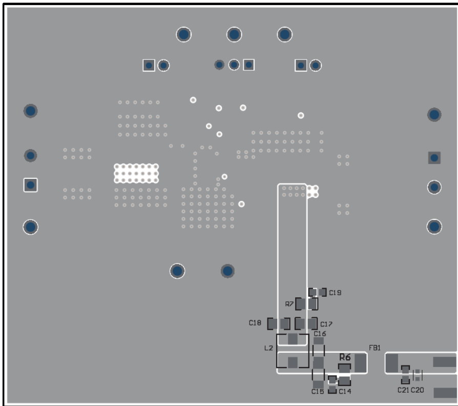
图 7-19. TPS54538 底层布局示例
