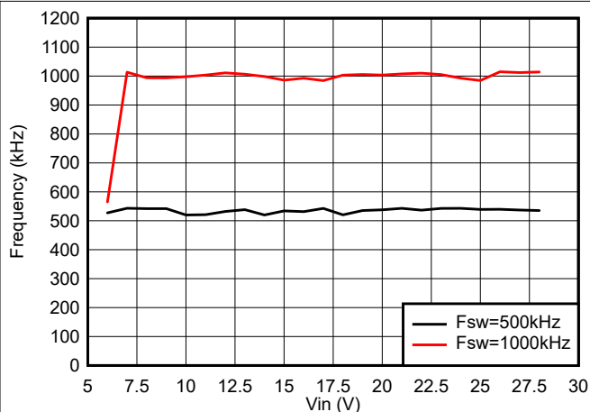
图 5-20. TPS54538 开关频率与 V_{IN} 间的关系, V_{OUT} = 5\text{V} , I_{OUT} = 5\text{A}
