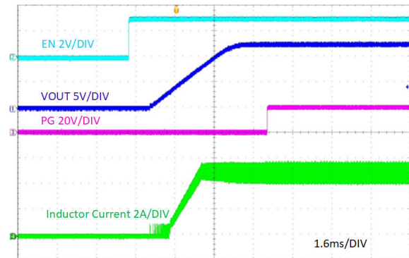
图 7-11. 通过 EN 的启动, I_{OUT} = 5A
