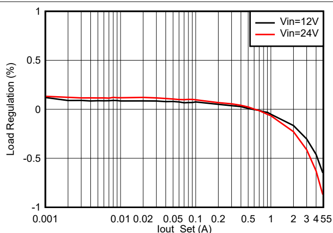
图 7-4. 负载调节 (PFM)
