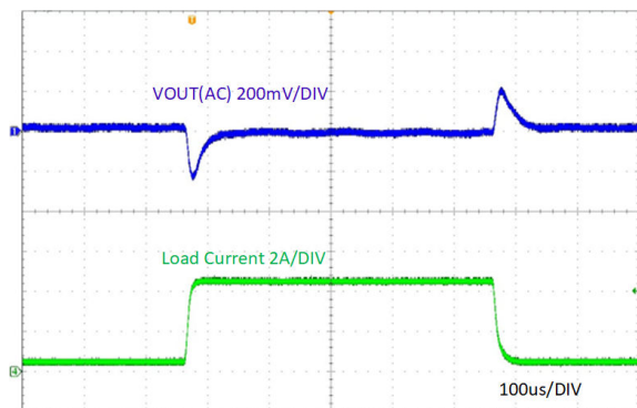
图 7-14. 负载瞬态响应，0.5A 至 4.5A，压摆率 = 0.8A/ μS
