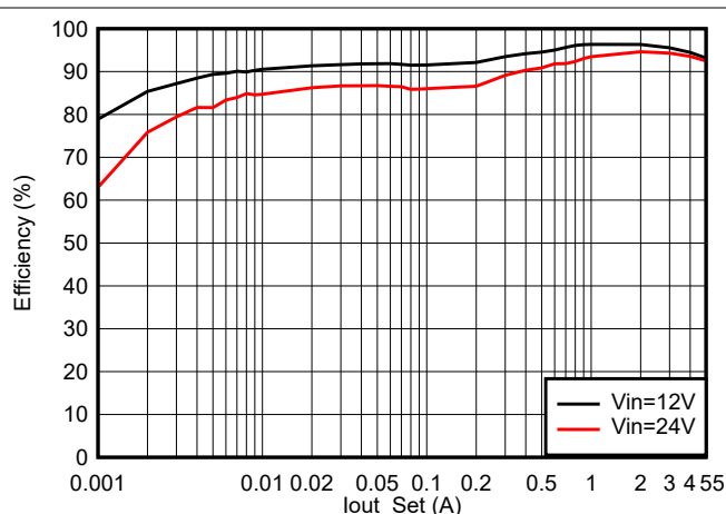
图 7-2. 效率 (PFM)
