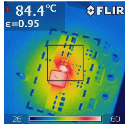
图 7-9. 外壳温度, V_{IN} = 24V , I_{OUT} = 5A , f_{sw} = 500kHz
