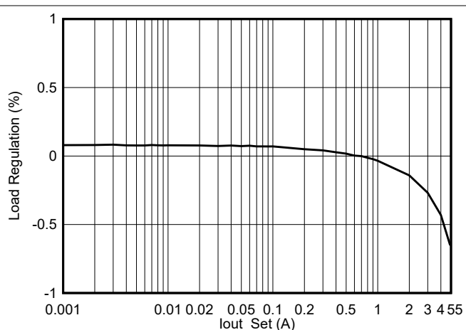
图 5-18. TPS54538 负载调节 (PFM), V_{IN} = 24\text{V} 、 V_{OUT} = 12\text{V} 、 f_{SW} = 500\text{kHz}
