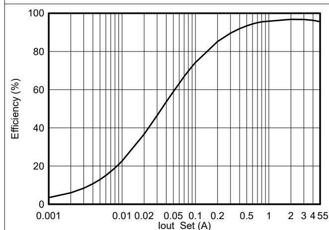
图 5-17. TPS54538 效率(FCCM), V_{IN} = 24\text{V} 、 V_{OUT} = 12\text{V} 、 f_{SW} = 500\text{kHz} 、 L = 5.6\mu\text{H}
