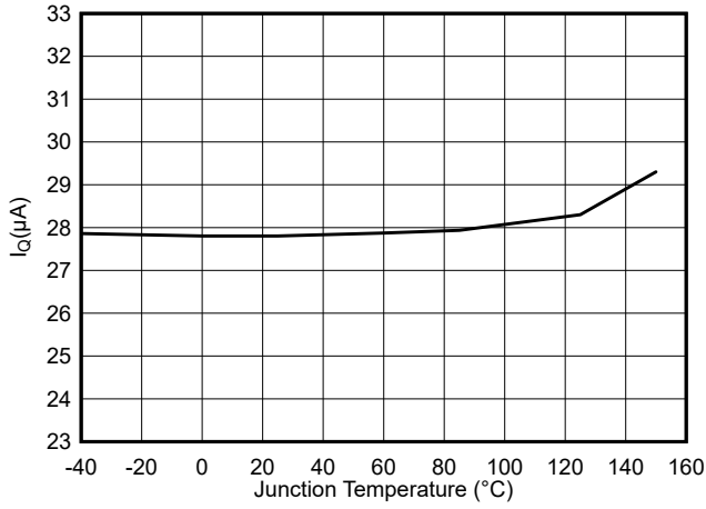
图 5-1. TPS54538 静态电流 (PFM) 与结温间的关系
