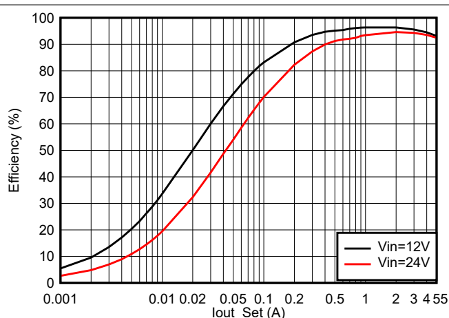
图 7-3. 效率 (FCCM)
