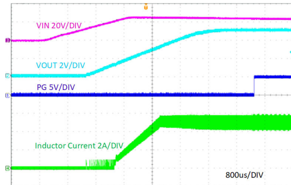
图 7-10. 相对于 V_{IN} 、 I_{OUT} = 5A 的启动
