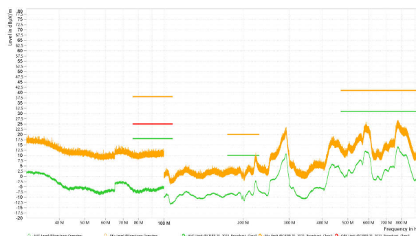
图 5-22. TPS54538 CISPR 25 5 类辐射发射, V_{IN} = 24\text{V} 、 V_{OUT} = 5\text{V} 、 I_{OUT} = 5\text{A} , 启用展频
