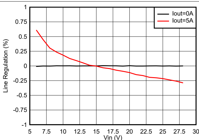
图 7-7. 线路调整率 (FCCM)
