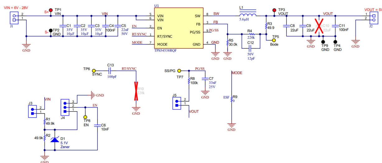
图 7-1. TPS54538 5V 输出、5A 参考设计
