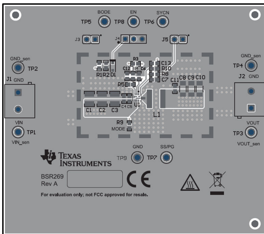
图 7-18. TPS54538 顶层布局示例
