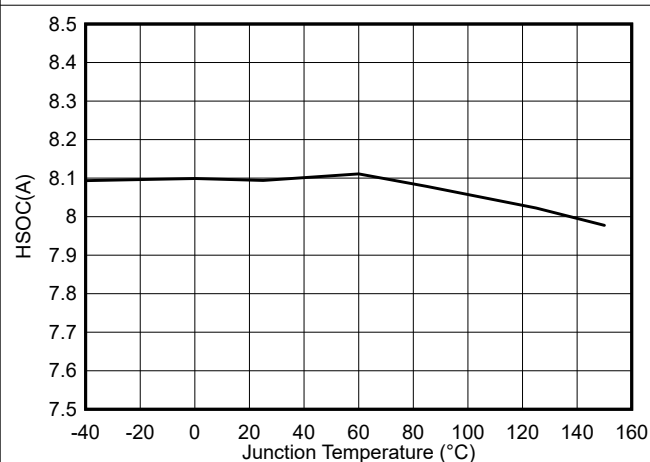
图 5-11. TPS54538 高侧电流限值与结温间的关系
