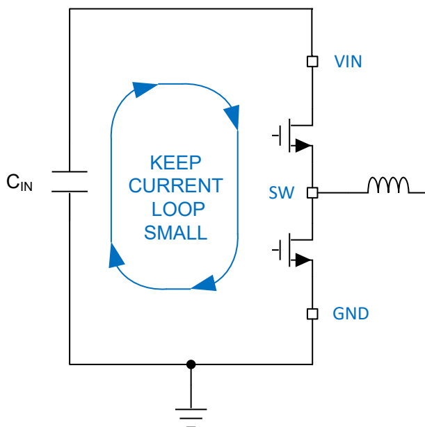
图 7-17. 具有快速边沿的电流环路
