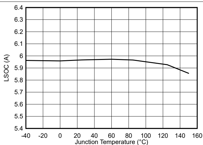
图 5-12. TPS54538 低侧电流限值与结温间的关系
