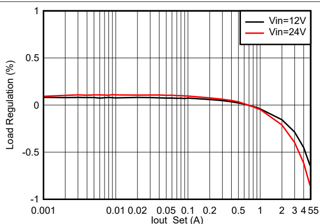
图 7-5. 负载调节 (FCCM)
