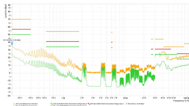
图 5-21. TPS54538 CISPR 25 5 类传导发射, V_{IN} = 24\text{V} 、 V_{OUT} = 5\text{V} 、 I_{OUT} = 5\text{A} , 启用展频
