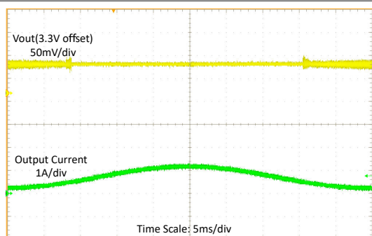
图 8-14. 输入电压为 2.7V 时的负载扫描
