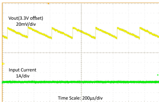
图 8-10. 负载为 1mA 时的稳定状态波形
