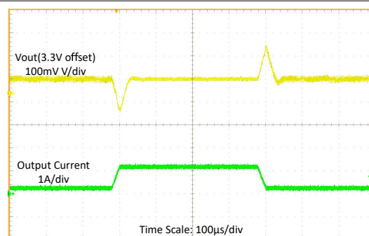
图 8-15. 输入电压为 3.6V 时的负载瞬态
