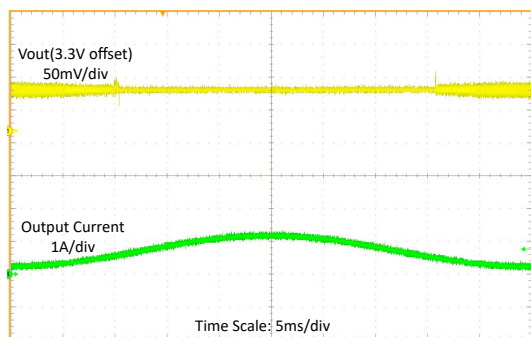
图 8-18. 输入电压为 4.3V 时的负载扫描
