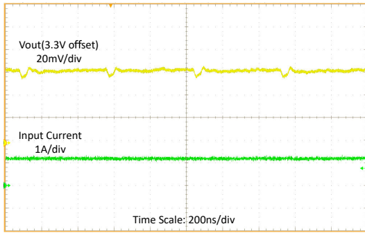
图 8-8. 负载为 1A 并采用降压/升压时的稳定状态波形
