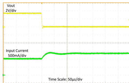
图 8-21. 输出短路保护 ( 进入 )
