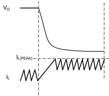
图 7-3. 短路保护期间的典型器件行为
