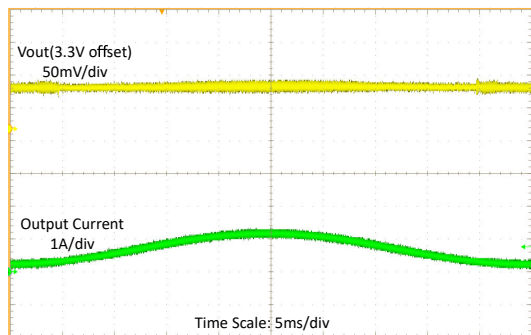
图 8-14. 输入电压为 2.7V 时的负载扫描
