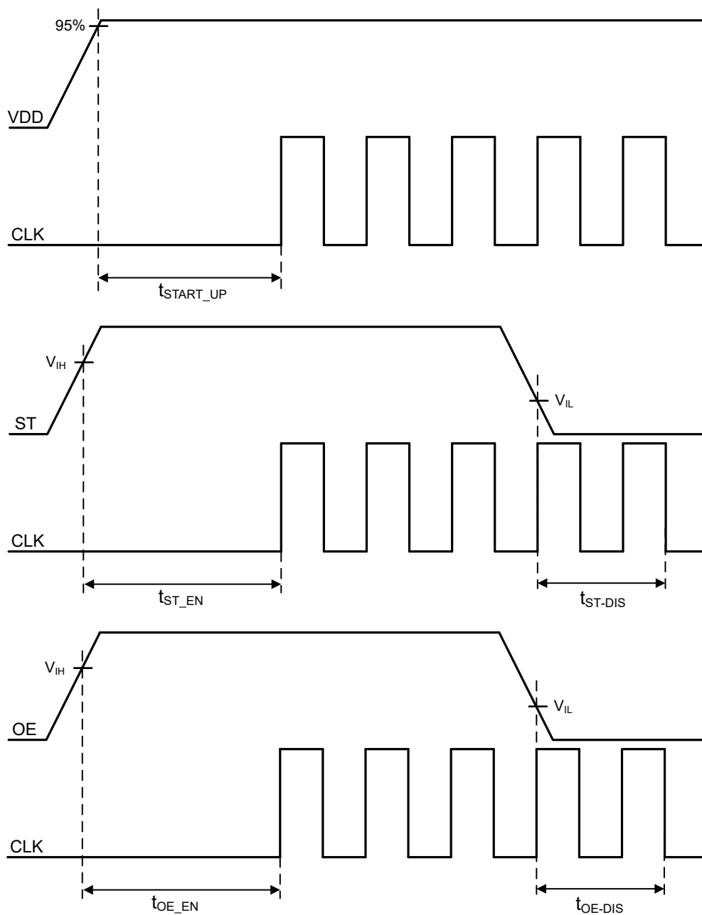
图 6-2. 上电特性
