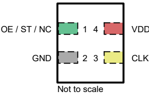
图 5-1. CDC6Cx 4 引脚 VSON ( 顶视图 )
