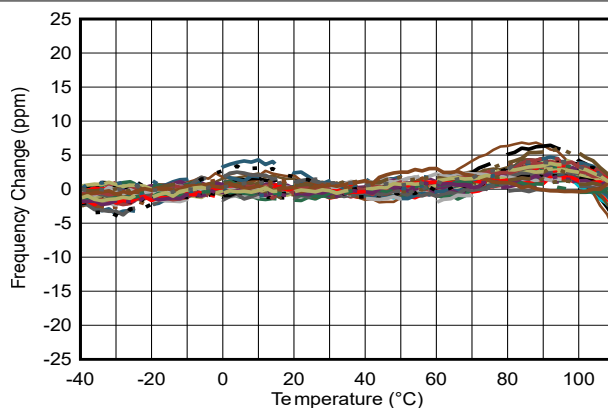
图 6-14. 频率变化与温度间的关系 (25MHz、3.3V 电源电压、80 个器件)
