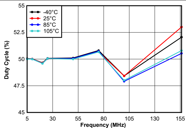
图 6-13. 占空比与频率和温度间的关系 (1.8V 电源电压, 无容性负载, 正常模式器件)
