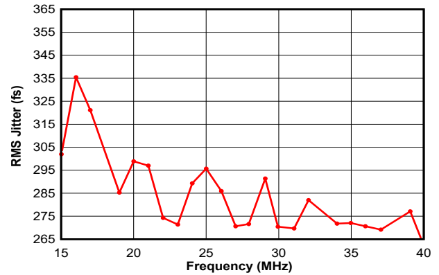
图 6-8. 典型 RMS 抖动与频率的关系 ( 3.3V 电源电压, 25°C, 带宽 12kHz 至 5MHz )
