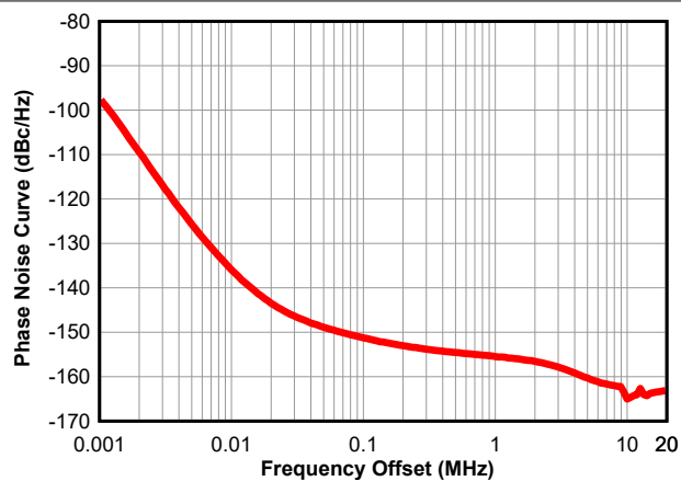
图 6-10. 相位噪声曲线 (25MHz、25°C 和 3.3V 电源电压)
