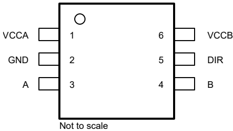
图 4-3. DRL 封装，6 引脚 SOT-5X3 ( 顶视图 )
