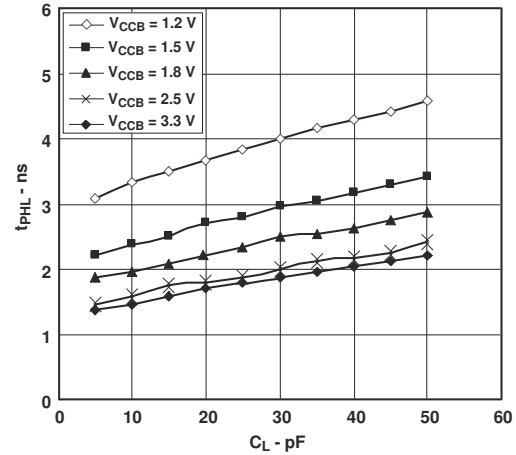
图 5-10. 低电平到高电平 (A 到 B) 的典型传播延迟与负载电容间的关系 T A = 25°C、V CCA = 3.3V
