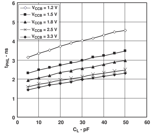
图 5-8. 低电平到高电平 (A 到 B) 的典型传播延迟与负载电容间的关系 T A = 25°C、V CCA = 2.5V
