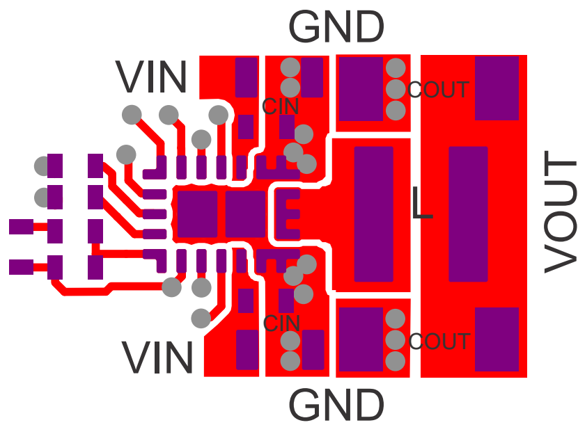
图 9-25. 布局示例
