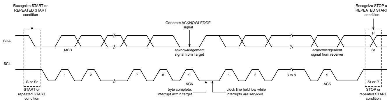
图 7-19. 总线协议
