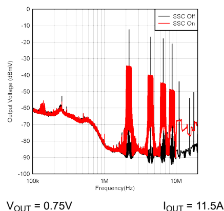
图 9-19. 扩频运行
