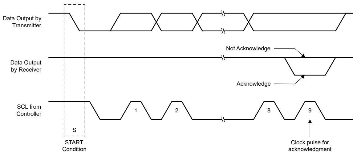
图 7-18. I²C 总线上的确认
