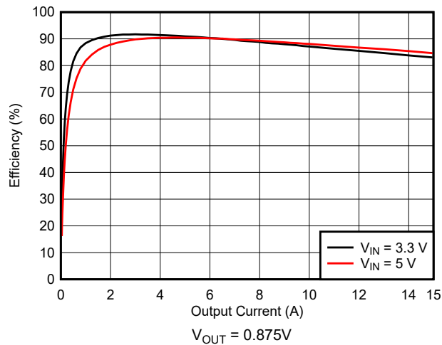
图 9-8. 效率
