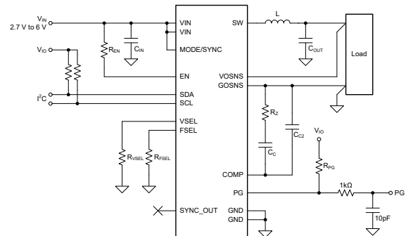
TPS6287x-Q1 简化原理图
