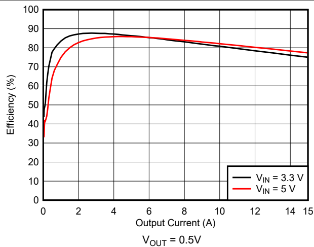
图 9-4. 效率
