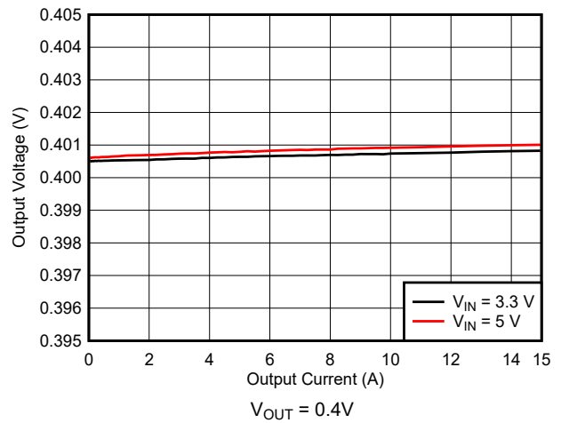
图 9-3. 负载调整率
