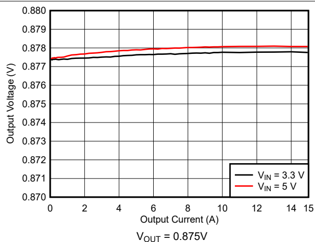
图 9-9. 负载调整率
