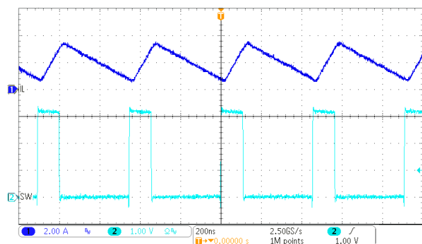
图 9-16. PWM-CCM 运行
