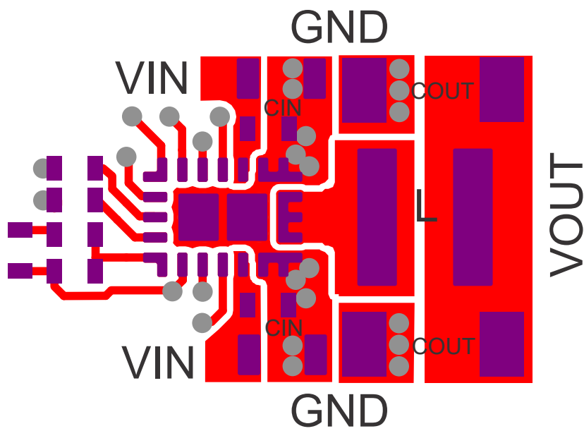
图 9-25. 布局示例
