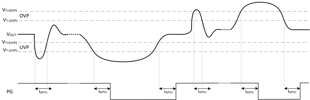
图 7-12. PG 时序
