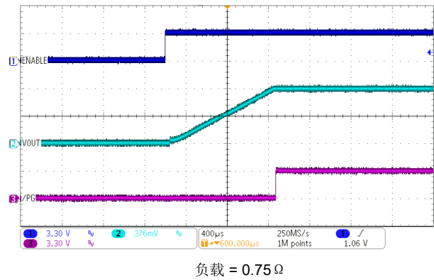
图 9-21. 通过 EN 引脚启动
