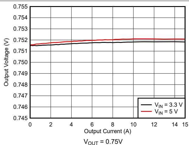
图 9-7. 负载调整率
