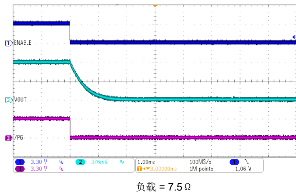
图 9-22. 通过 EN 引脚关断 (启用放电)
