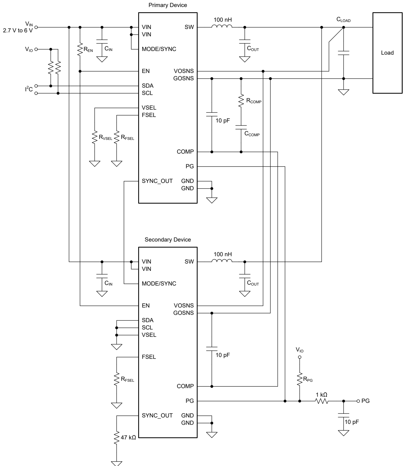
图 7-15. 堆叠配置中的两个 TPS6287x-Q1 器件
