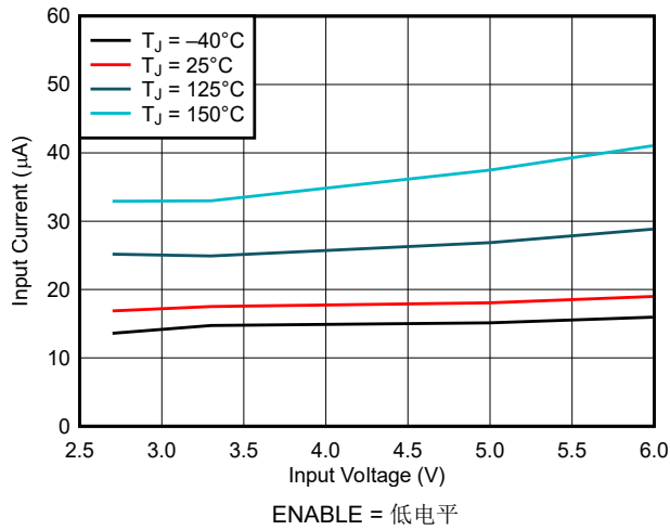
图 6-3. 静态电源电流
