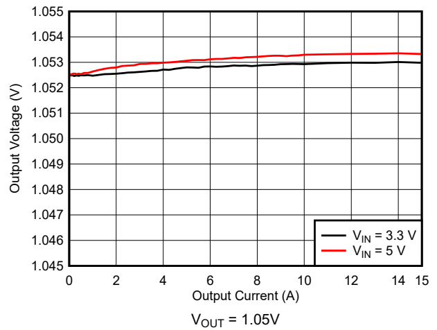
图 9-11. 负载调整率
