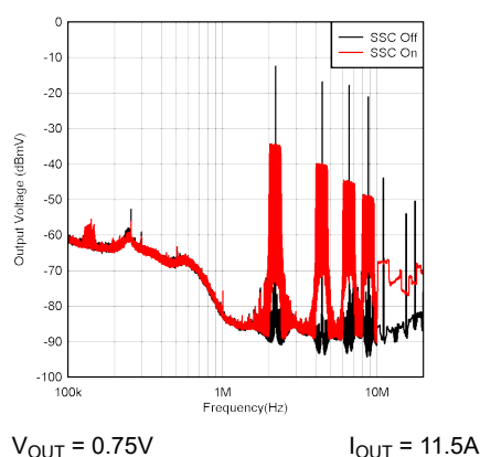
图 9-19. 扩频运行
