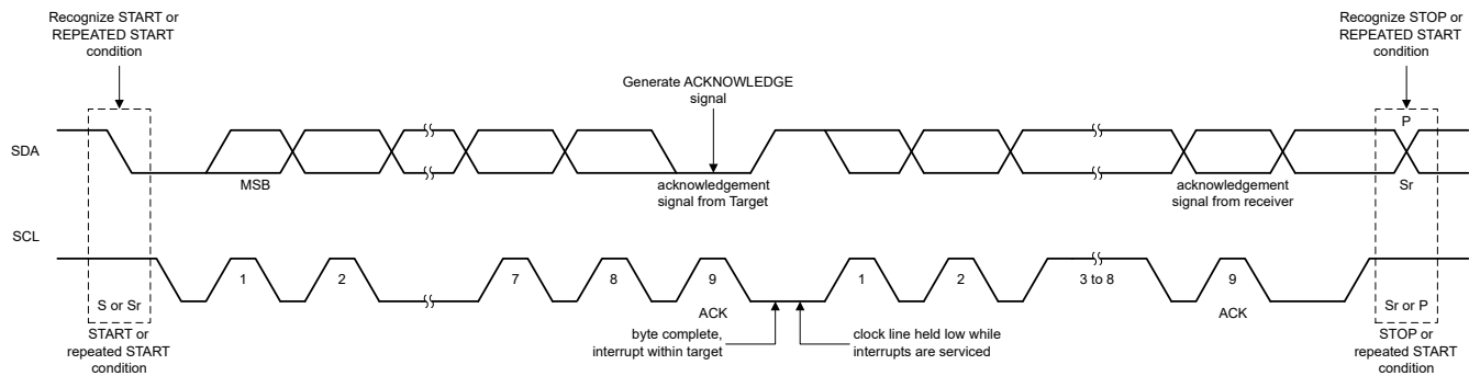
图 7-19. 总线协议
