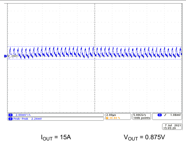
图 9-13. 输出电压纹波
