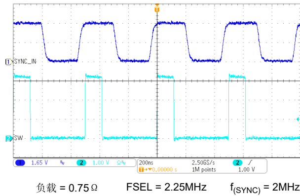
图 9-20. 可与外部时钟保持同步
