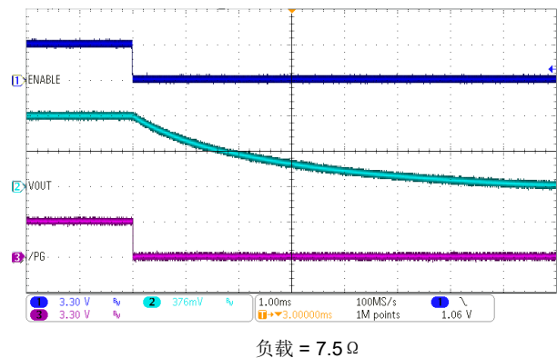
图 9-23. 关断 (禁用放电)
