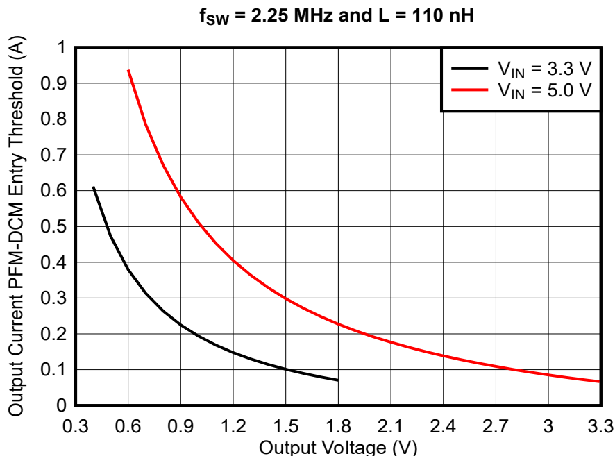
图 7-5. 输出电流 PFM-DCM 进入阈值
