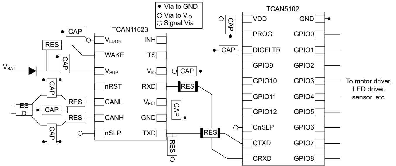
图 8-2. 布局示例
