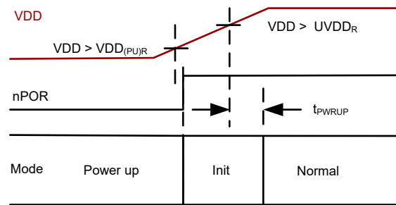
图 6-1. 上电时序
