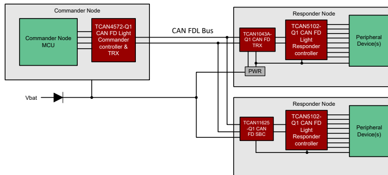
CAN FD 光命令器/响应器应用
