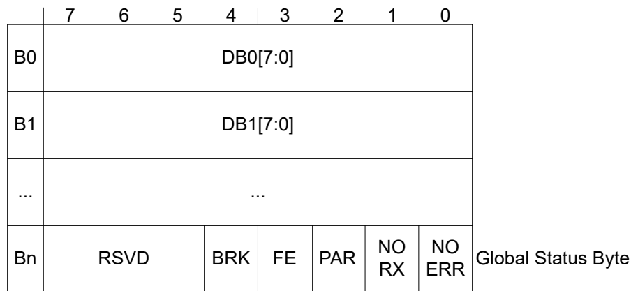
图 7-98. UART 接收 FIFO 突发读取
