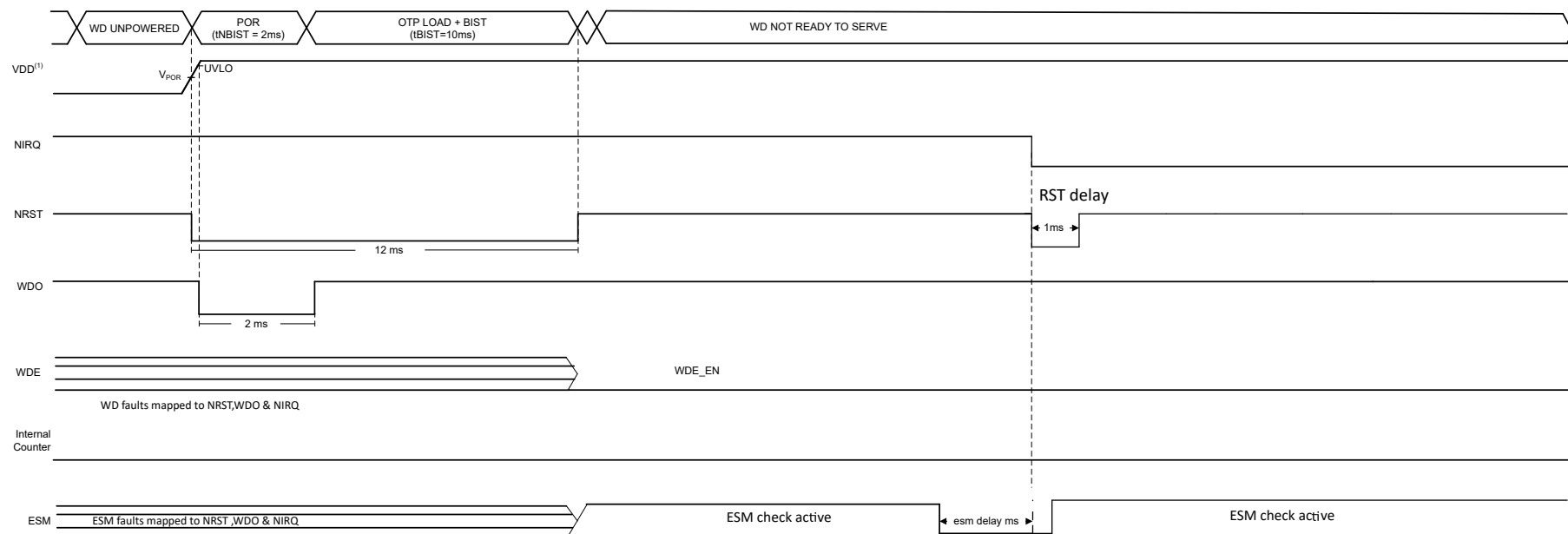
图 7-28. 瞬态 ESM 故障 (WD 禁用)
