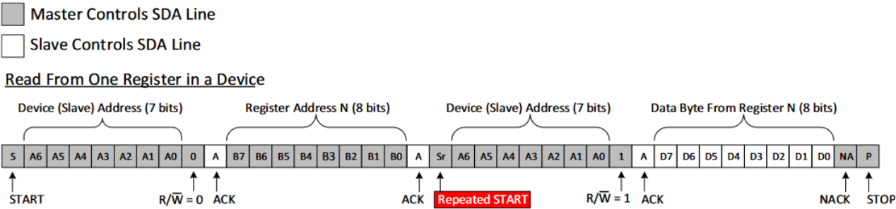
图 7-4. I 2 C 读取协议
