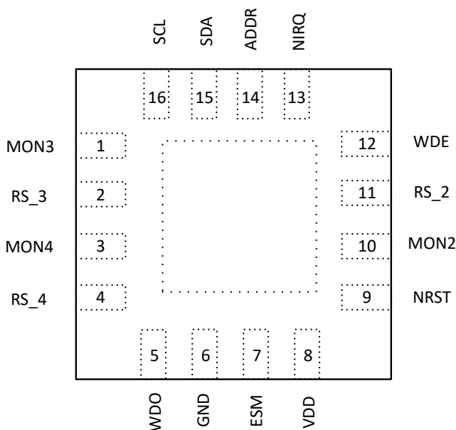
图 5-1. RTE 封装 16 引脚 WQFN TPS389C03-Q1 ( 顶视图 )
