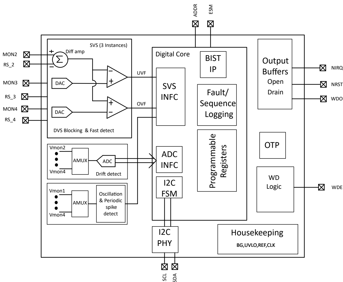
图 7-1. TPS389C03-Q1 方框图
