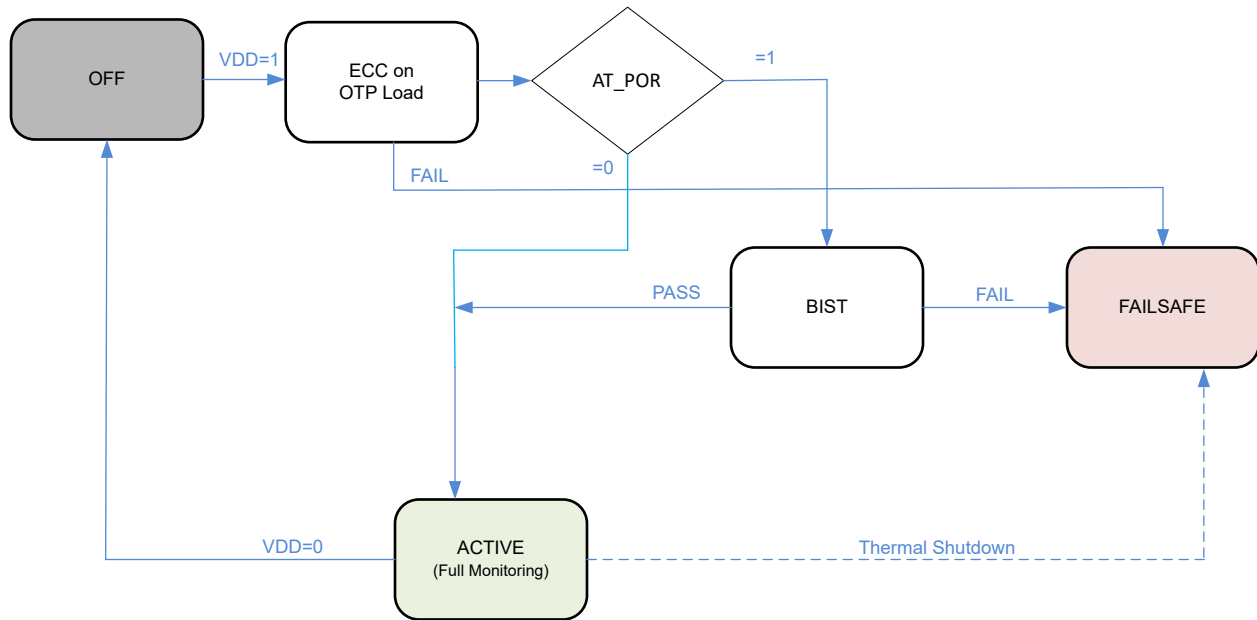
图 7-30. TPS389C03-Q1 状态图
