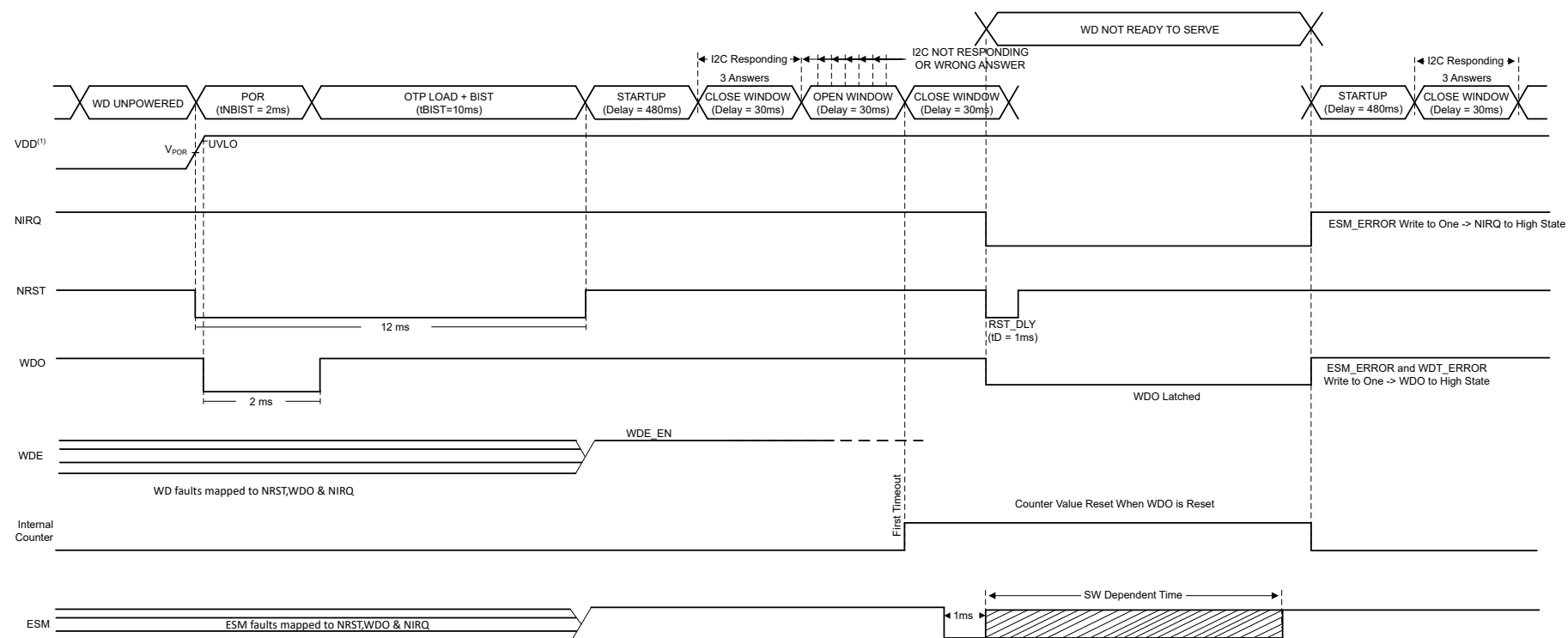
图 7-19. WD 超时后的 TPS389C03 ESM 错误
