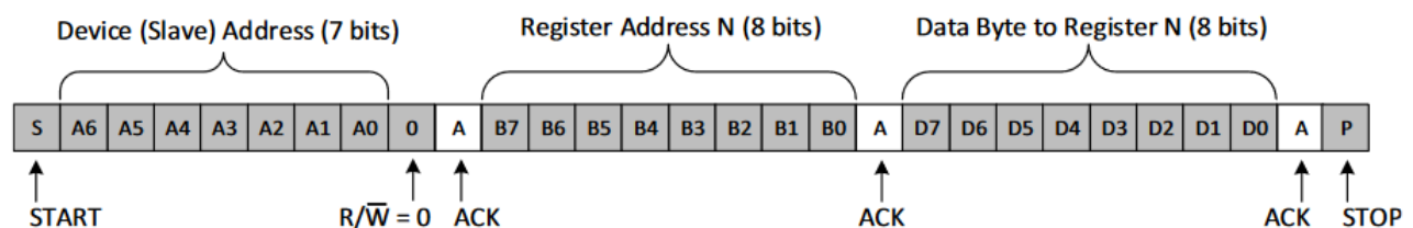
图 7-3. I 2 C 写入协议
