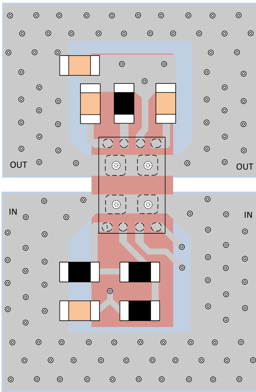
图 8-26. 布局示例
