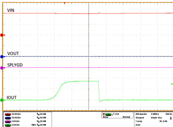
图 8-11. 唤醒至短路保护
