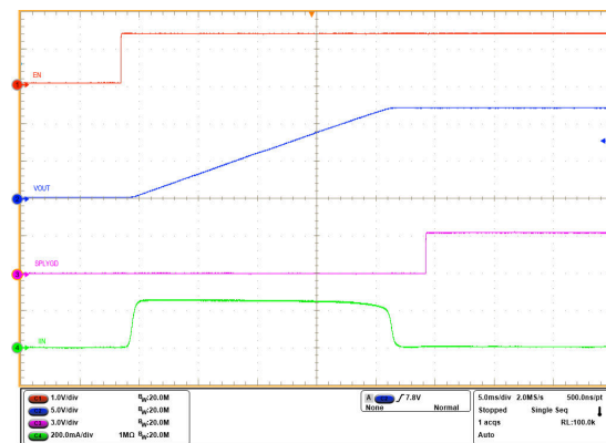
图 6-28. 通过电源启动
