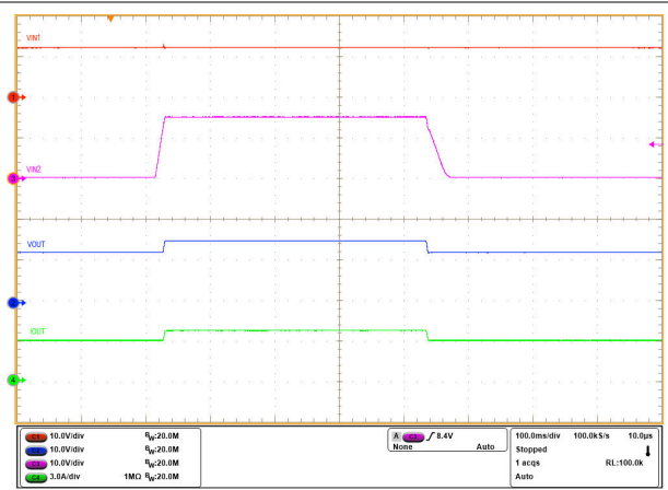
图 8-15. 有源 ORing 响应
