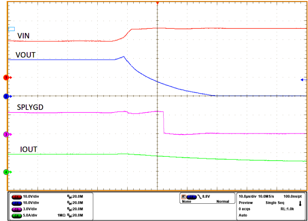
图 8-8. 过压保护
