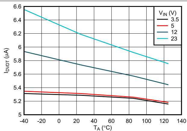
图 6-24. DVDVT 充电电流与温度间的关系
