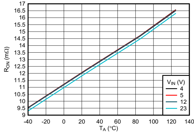
图 6-1. 导通电阻与温度间的关系
