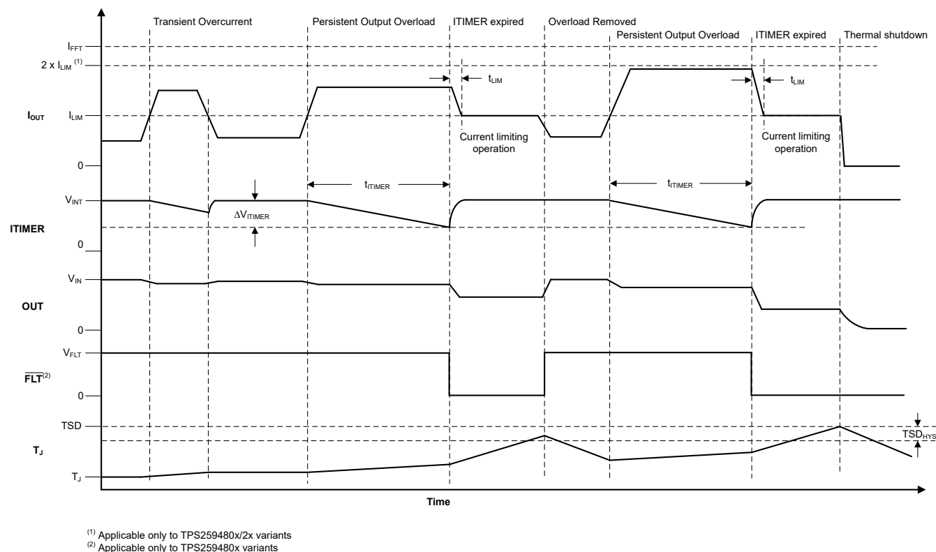
图 7-8. TPS25948xx 主动电流限制响应
