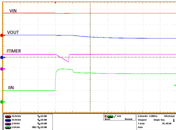
图 8-9. 过流保护
