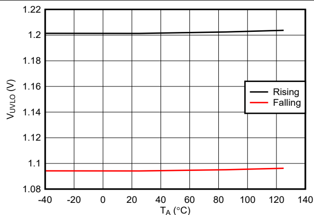
图 6-10. EN/UVLO FET 关断阈值与温度间的关系
