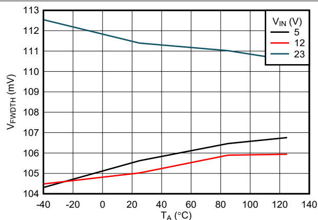
图 6-19. RCB — 正向比较器阈值与温度间的关系
