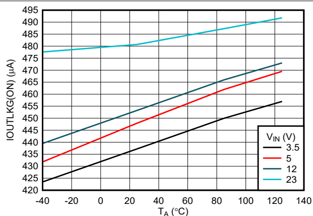
图 6-20. 导通状态反向电流阻断期间的输出漏电流
