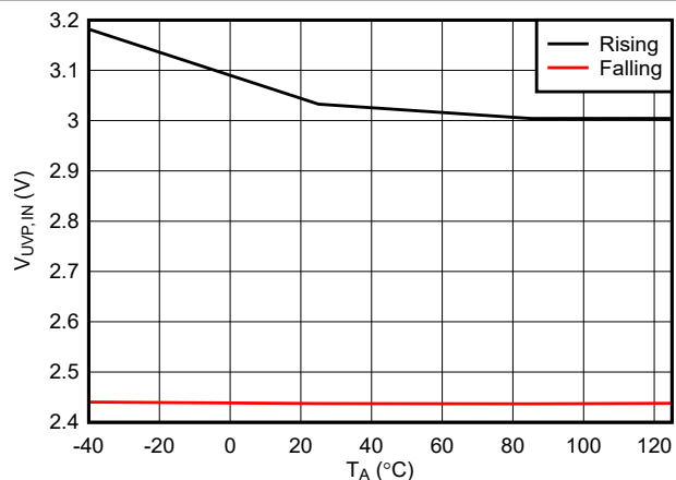
图 6-8. 输入欠压保护阈值与温度间的关系
