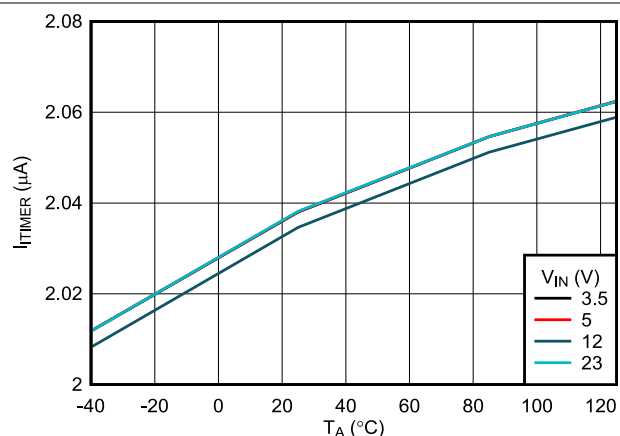
图 6-23. ITIMER 放电电流与温度间的关系
