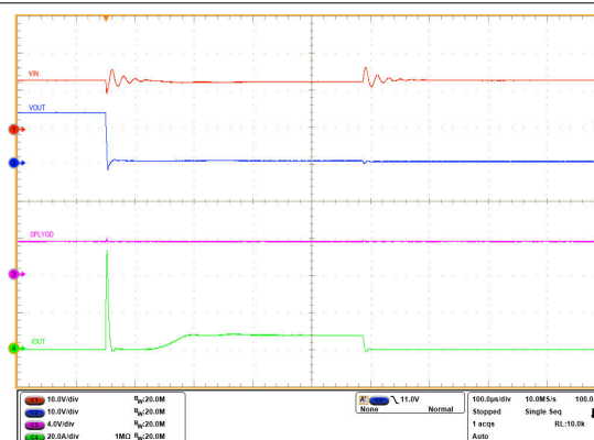
图 6-34. 瞬态过流消隐计时器响应
