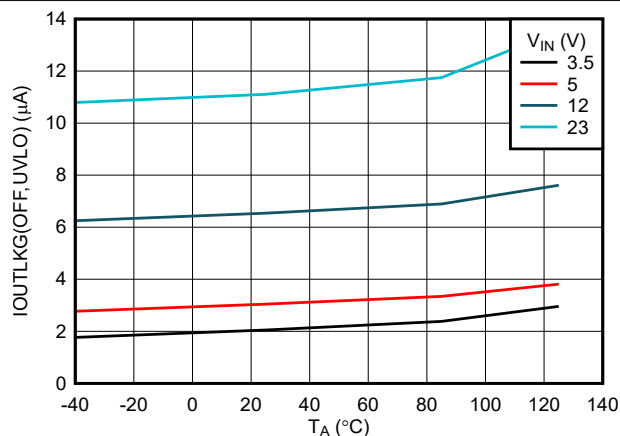
图 6-21. 关断状态期间的反向漏电流
