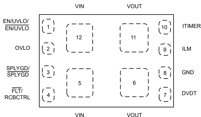
图 5-1. YWP 封装，12 焊球 PWCSP ( 顶视图 )
