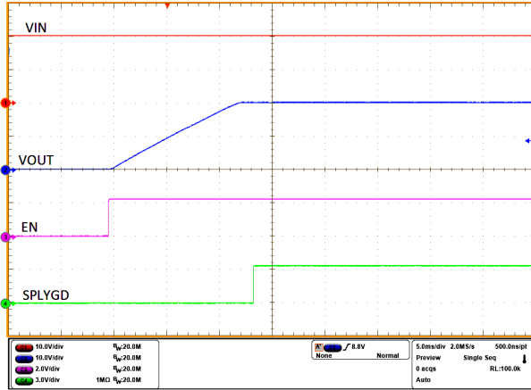
图 8-7. 上电
