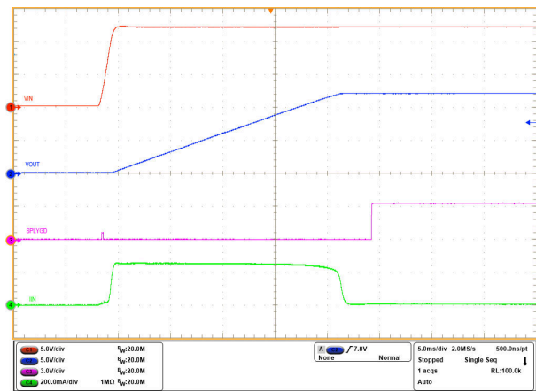
图 6-26. 浪涌状态期间的热关断时间
