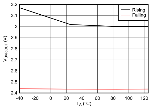
图 6-9. 输出欠压保护阈值与温度间的关系
