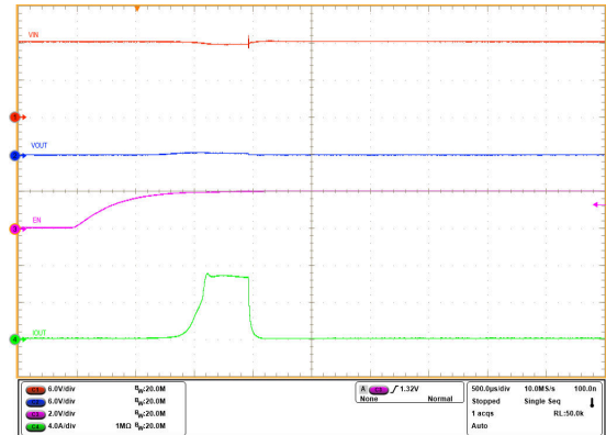
V_{IN} = 12V , OUT 短路至 GND, I_{LIM} 设置为 4.5A , V_{EN/UVLO} 从 0V 升至 2V
