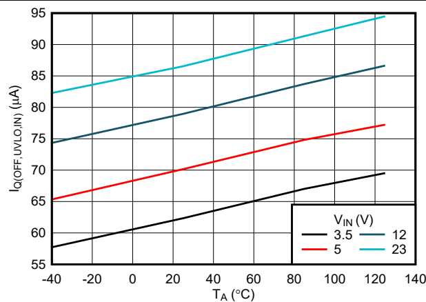
图 6-3. 输入关断状态 (UVLO) 电流与温度间的关系
