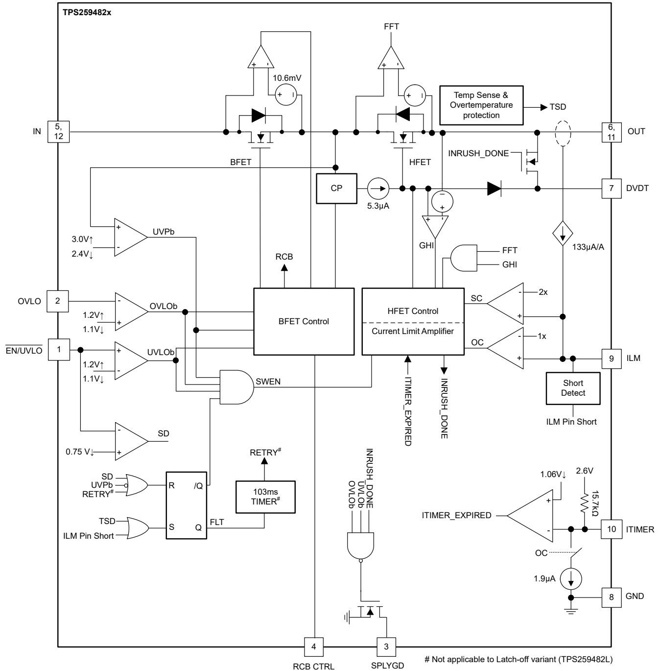
图 7-3. TPS25948x 方框图
