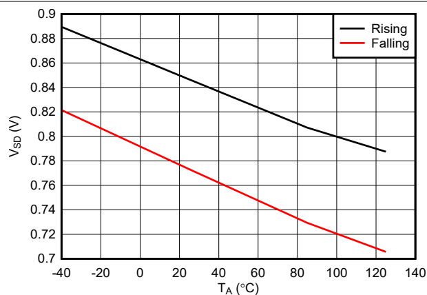
图 6-11. EN/UVLO 关断阈值与温度间的关系
