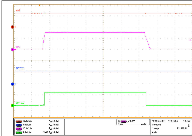
图 8-14. 有源 ORing 响应
