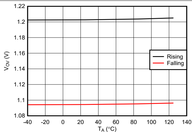
图 6-12. OVLO 阈值与温度间的关系
