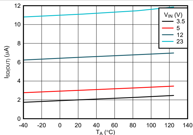
图 6-7. OUT 关断电流与温度间的关系
