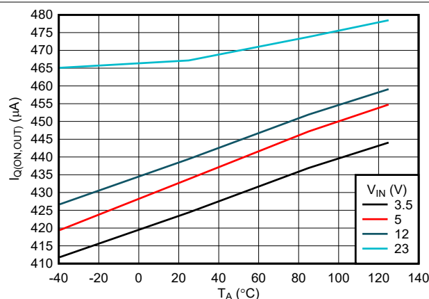
图 6-5. OUT 静态电流与温度间的关系
