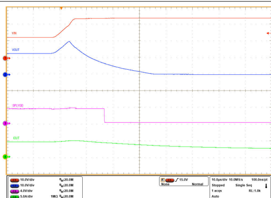
图 6-31. 具有阻止性和容性负载时的浪涌电流
