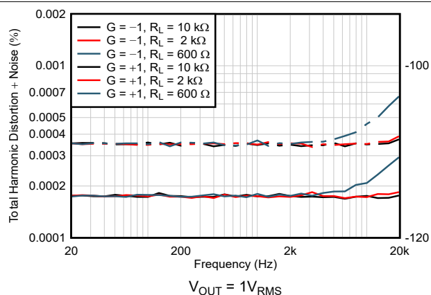
图 5-30. THD+N 与频率间的关系
