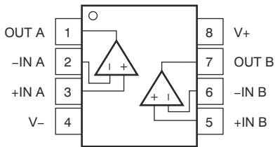
图 4-3. OPA2328 D 和 DGK 封装 8 引脚 SOIC 和 VSSOP ( 顶视图 )
