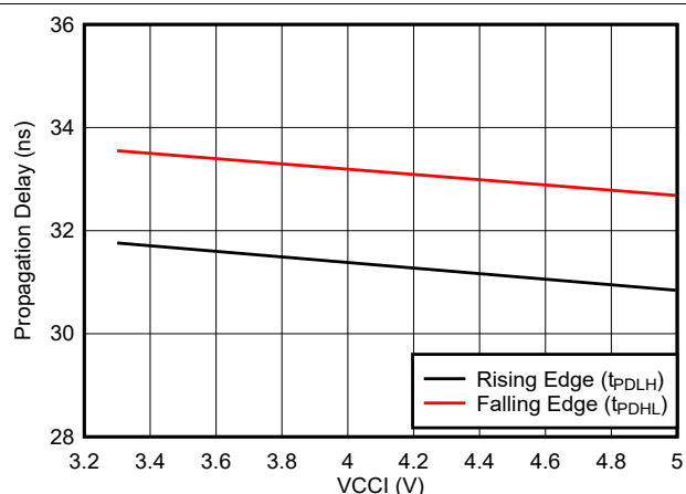
图 5-17. 传播延迟与 VCCI 之间的关系
