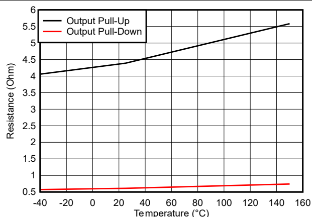
图 5-15. 输出电阻与温度之间的关系
