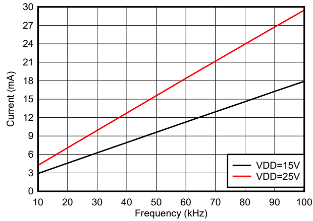
图 5-10. 每通道电流消耗 ( I_{VDDA/B} ) 与频率之间的关系 (10nF 负载, V_{DD} = 15V 或 25V )
