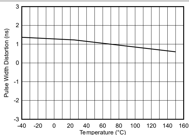
图 5-18. 脉宽失真度与温度之间的关系
