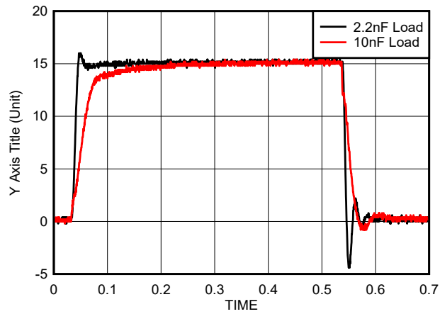
图 5-34. 典型输出波形
