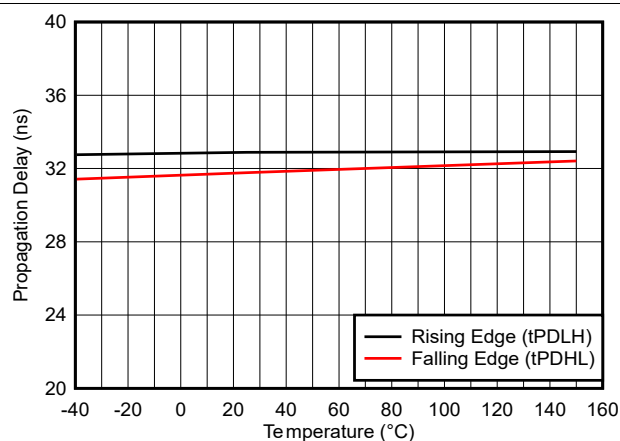
图 5-16. 传播延迟与温度间的关系
