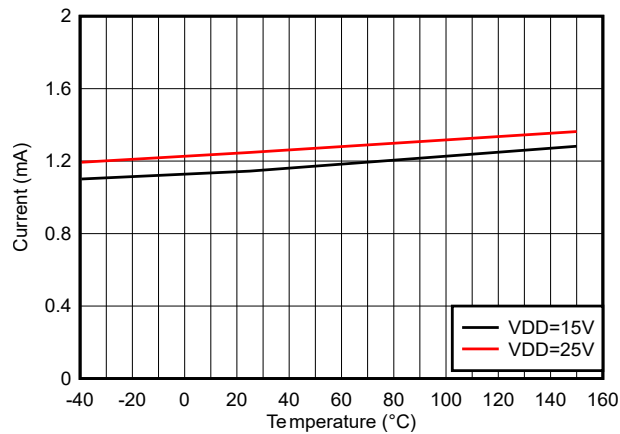
图 5-12. 每通道 ( I_{VDDA/B} ) 静态电源电流与温度之间的关系 (无负载, 低电平输入, 无开关)
