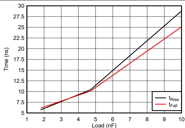
图 5-14. 上升和下降时间与负载间的关系 (VDD = 15V)
