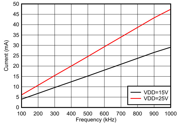
图 5-9. 每通道电流消耗 ( I_{VDDA/B} ) 与频率之间的关系 (1nF 负载, V_{DD} = 15V 或 25V )
