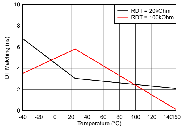
图 5-33. 死区时间匹配与温度之间的关系 ( R_{DT} = 20\text{k}\Omega 和 100\text{k}\Omega )
