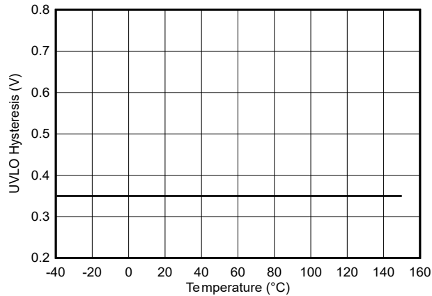
图 5-22. VDD 5V UVLO 迟滞与温度间的关系
