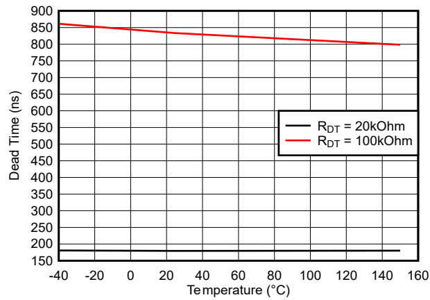
图 5-32. 死区时间与温度之间的关系 ( R_{DT} = 20\text{k}\Omega 和 100\text{k}\Omega )
