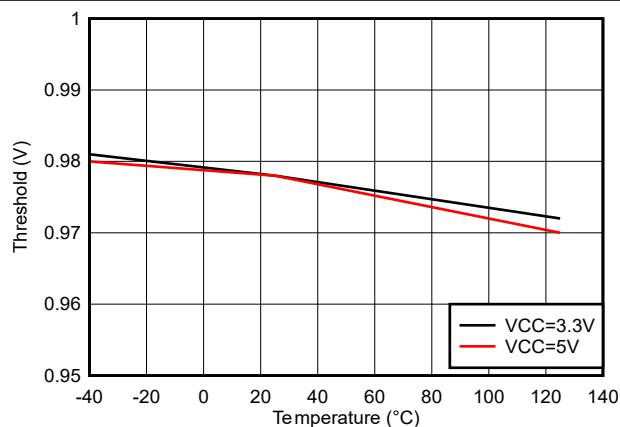
图 5-30. IN/EN 低阈值
