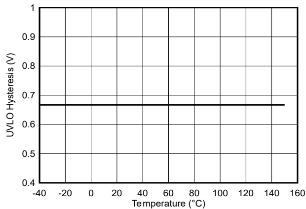
图 5-24. VDD 8V UVLO 迟滞与温度间的关系
