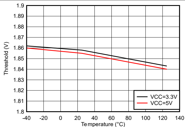
图 5-31. IN/EN 高阈值
