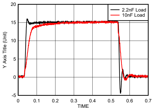
图 5-34. 典型输出波形
