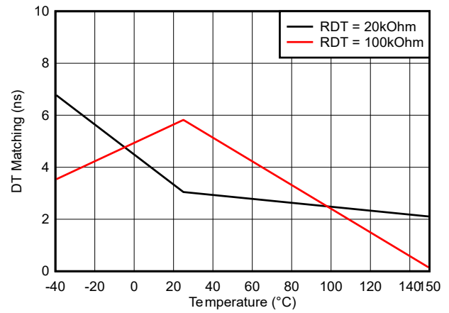
图 5-33. 死区时间匹配与温度之间的关系 ( R_{DT} = 20k\Omega 和 100k\Omega )
