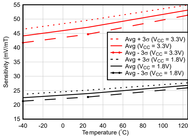
图 6-23. TMAG5253UA5 灵敏度与温度间的关系
