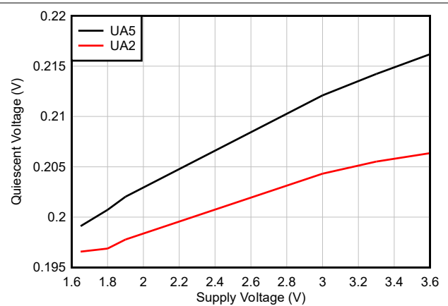
图 6-18. 静态电压与电源电压之间的关系
