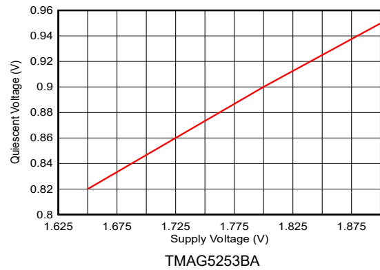
图 6-6. TMAG5253BA 静态电压与电源电压间的关系
