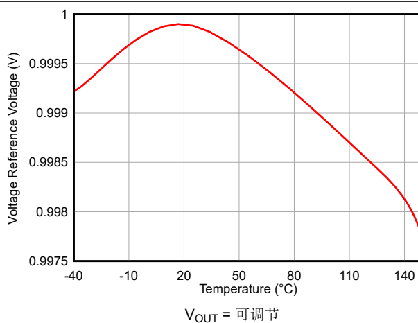
图 6-4. 反馈电压精度与温度间的关系
