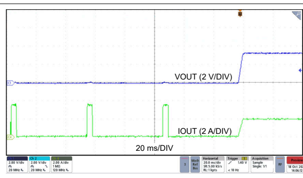
图 7-12. 退出断续
