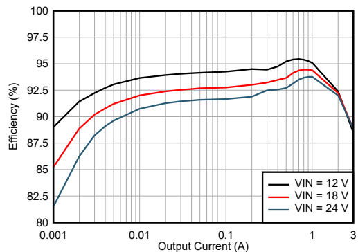
LMQ66430R5R V_{OUT} = 5V 400kHz (自动) 固定式
