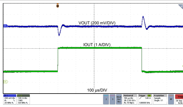
LMQ66430R5R V_{OUT} = 5V 400kHz (自动) 1A 至 3A, 1A/ \mu s 固定式
