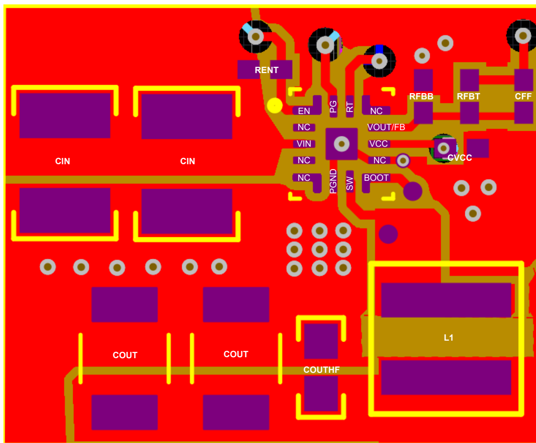
图 8-13. 布局示例
