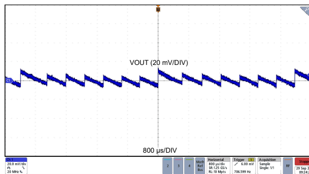
LMQ66430R5R V_{OUT} = 5V 0A 负载 固定式
