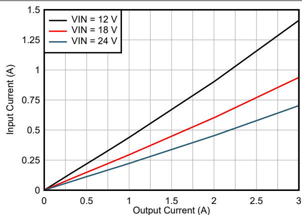
LMQ66430R5R V_{OUT} = 5V 400kHz (自动) 固定式
