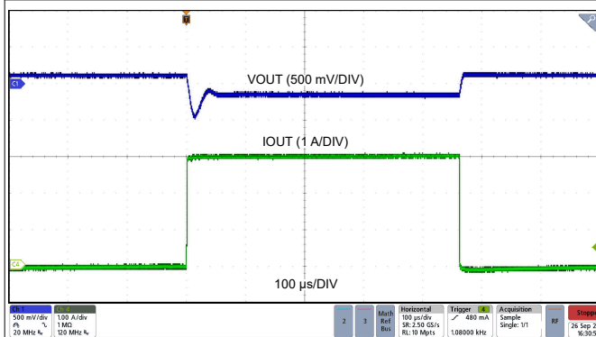
LMQ66430R5R V_{OUT} = 5V 400kHz (自动) 0A 至 3A, 1A/ \mu s 固定式
