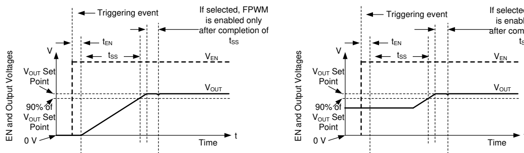
图 7-7. 带和不带预偏置电压的软启动
