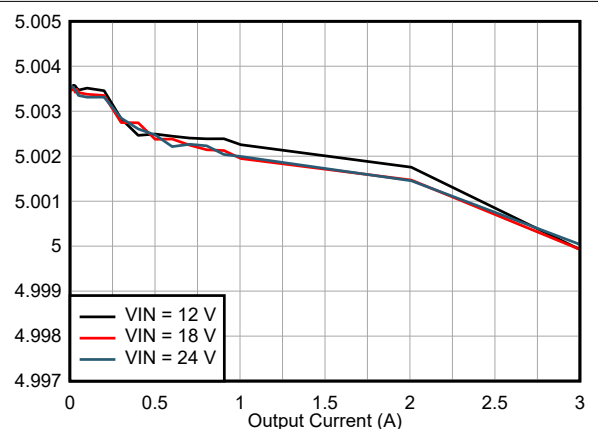
LMQ66430R5R V_{OUT} = 5V 400kHz (自动) 固定式
