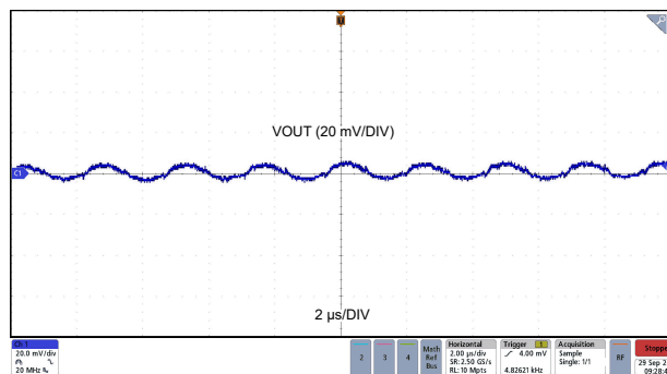
LMQ66430R5R V_{OUT} = 5V 3A 负载 固定式
