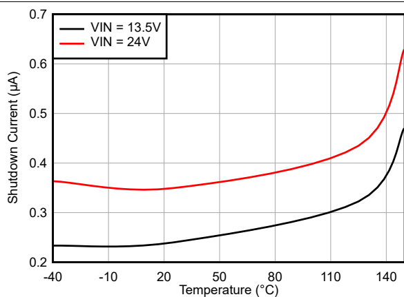
图 6-1. 关断电流与温度之间的关系
