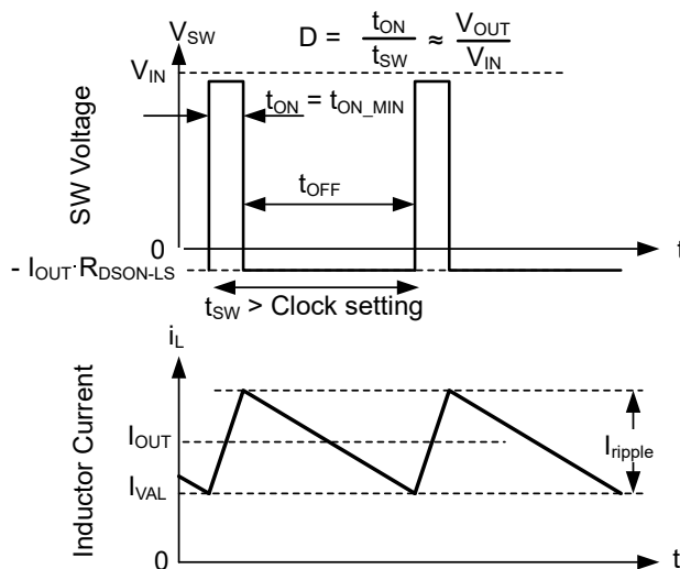
图 7-17. 谷值电流模式运行
