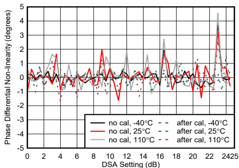
图 4-453. 9.6GHz 条件下 RX 相位微分非线性
