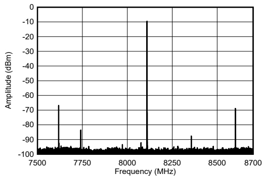
图 4-204. 8.1GHz 条件下 TX 单音输出频谱
