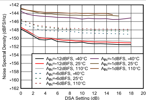
图 4-434. 8.1GHz 条件下 RX NSD 与 DSA 设置间的关系
