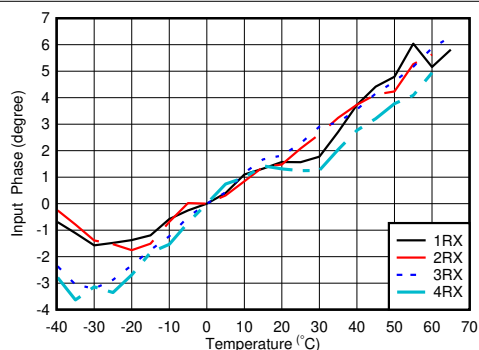
图 4-287. f_{\text{OUT}} = 0.8\text{GHz} 时 RX 输入相位与温度和 DSA 间的关系
