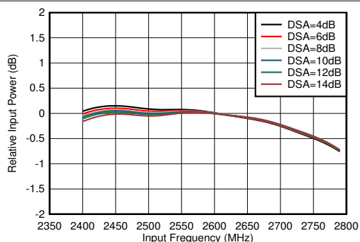
图 4-346. RX 带内增益平坦度， f_{\text{IN}} = 2600\text{MHz}
