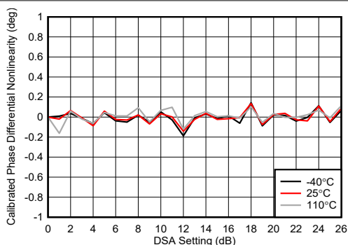
图 4-249. TX DSA 已校准相位积分非线性
