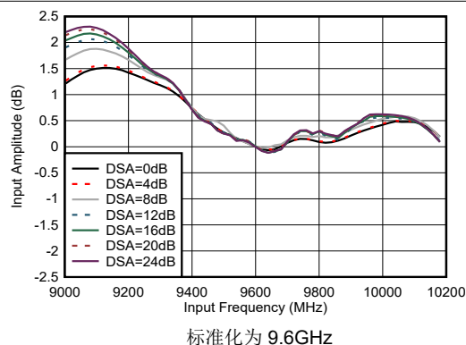
图 4-450. 9.6GHz 条件下 RX 输入振幅与频率间的关系
