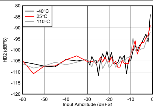
图 4-436. 8.1GHz 条件下 RX HD2 与数字振幅间的关系
