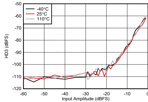
图 4-464. 9.6GHz 条件下 RX HD3 与数字电平间的关系
