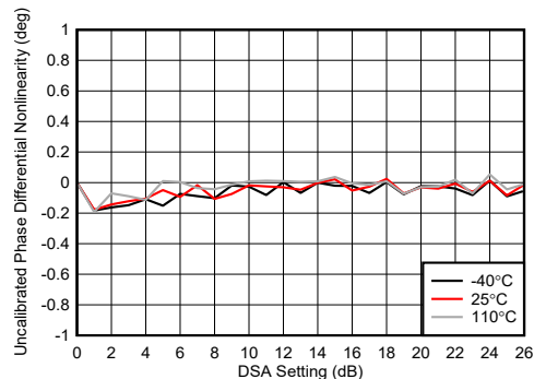
图 4-246. TX DSA 未校准相位微分非线性
