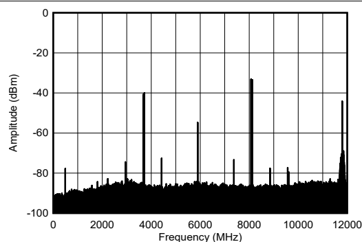
图 4-211. 8.1GHz 条件下 TX 双音输出频谱
