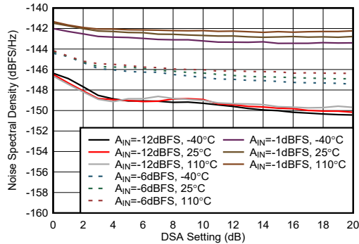
图 4-461. 9.6 GHz 条件下 RX NSD 与 DSA 设置间的关系
