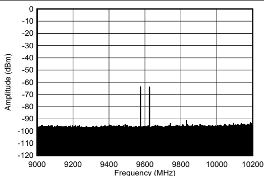
图 4-277. 9.61GHz 和单频 -30dBFS (1.2GHz 带宽) 条件下的 TX 双音频谱
