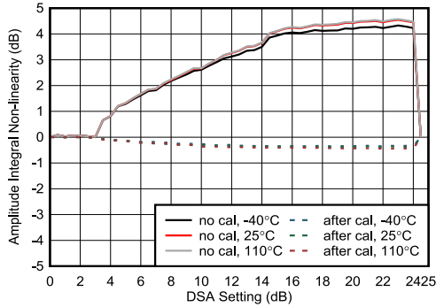
图 4-426. 8.1GHz 条件下 RX 振幅积分非线性
