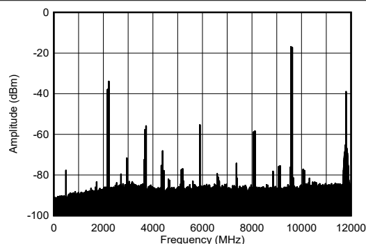
图 4-274. 9.61GHz 和 -13dBFS (宽带) 条件下的 TX 双音频谱
