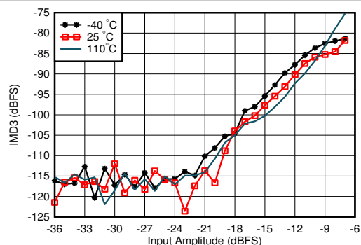
图 4-410. 4.9GHz 条件下 RX IMD3 与输入电平和温度间的关系
