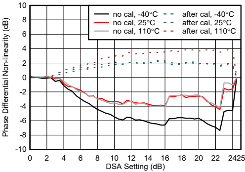
图 4-428. 8.1GHz 条件下 RX 相位微分非线性
