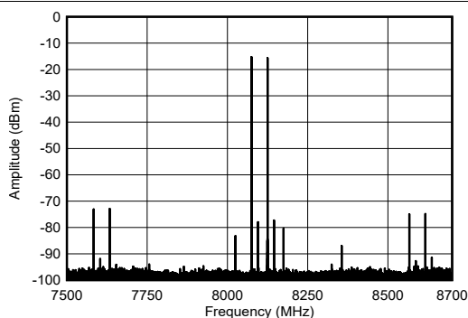
图 4-210. 8.1GHz 条件下 TX 双音输出频谱
