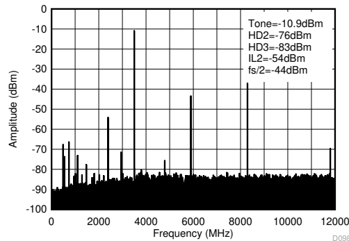
图 4-146. 3.5GHz (0 - f_{\text{DAC}} ) 条件下的 TX 单音 (-1dBFS) 输出频谱
