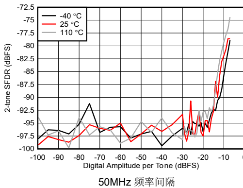
图 4-440. 8.11GHz 条件下 RX 双音 SFDR 与数字振幅间的关系
