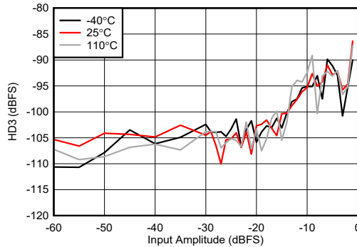
图 4-438. 8.11GHz 条件下 RX HD3 与数字振幅间的关系
