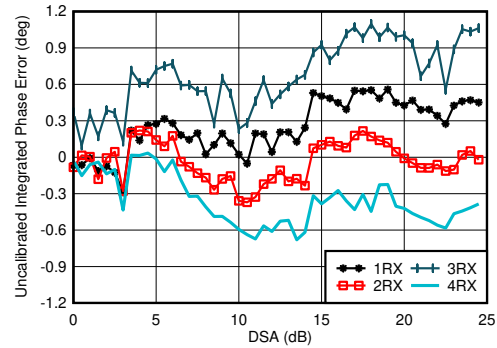
图 4-292. 0.8GHz 条件下 RX 未校准差分相位误差与 DSA 设置间的关系
