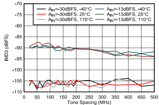
图 4-431. 8.11 GHz 条件下 RX IMD3 与频率间隔间的关系
