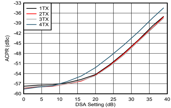
图 4-227. 8.1GHz 条件下 TX NR100MHz alt-ACPR 与 DSA 设置间的关系
