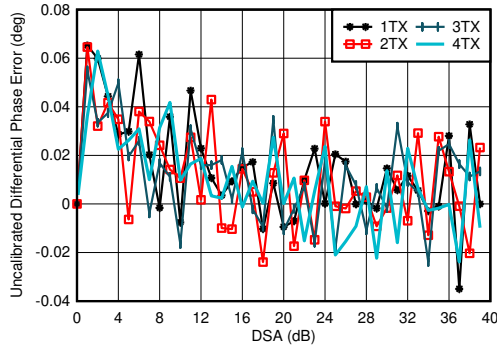
图 4-124. 3.5GHz 条件下 TX 未校准差分相位误差与 DSA 设置和通道间的关系
