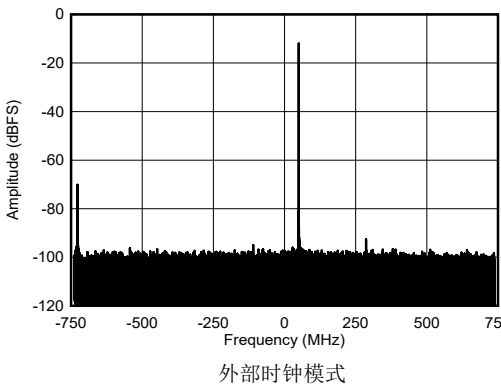
图 4-442. 8.11GHz 条件下 RX 单频输出 FFT, -12dBFS
