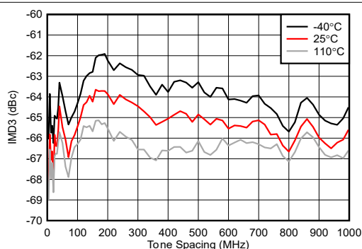
图 4-259. 9.61 GHz 条件下 TX IMD3 与频率间隔间的关系
