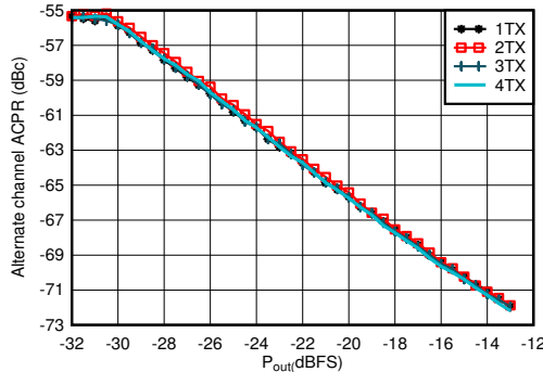
图 4-70. 1.8425GHz 条件下 TX 20MHz LTE alt-ACPR 与数字电平间的关系
