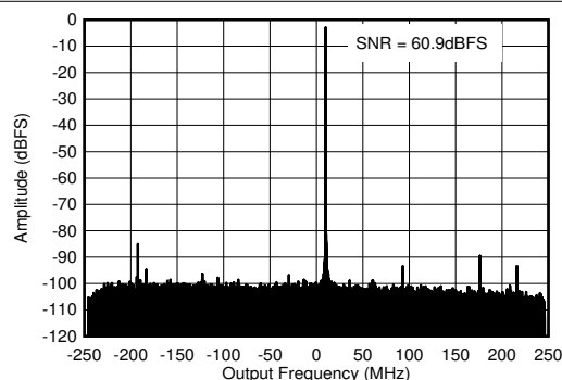
图 4-327. 1.75GHz 条件下的 RX 输出 FFT
