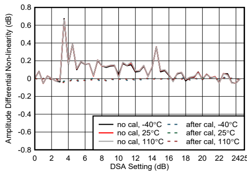
图 4-425. 8.11GHz 条件下 RX 振幅微分非线性
