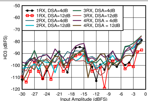
图 4-338. 1.9GHz 条件下 RX HD3 与 DSA 设置和通道间的关系
