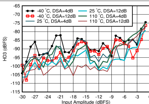
图 4-339. 1.9GHz 条件下 RX HD3 与 DSA 设置和温度间的关系
