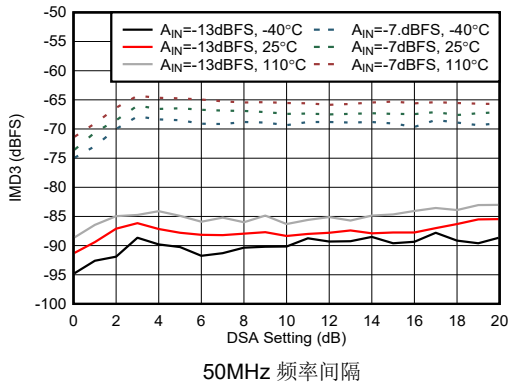
图 4-430. 8.11GHz 条件下 RX IMD3 与 DSA 设置间的关系
