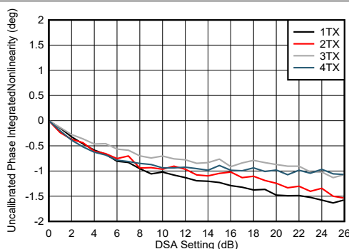
图 4-248. TX DSA 未校准相位积分非线性
