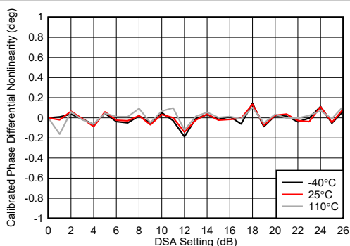
图 4-247. TX DSA 已校准相位微分非线性
