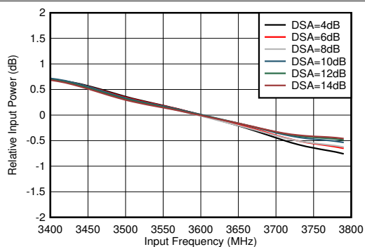
图 4-366. RX 带内增益平坦度， f_{\text{IN}} = 3600\text{MHz}
