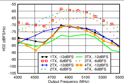
在 4.9 GHz 条件下匹配, f_{\text{DAC}} = 11.79648\text{GSPS} , 交错模式, 标准化为谐波频率下的输出功率
