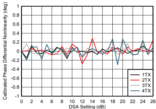
图 4-245. TX DSA 已校准相位微分非线性
