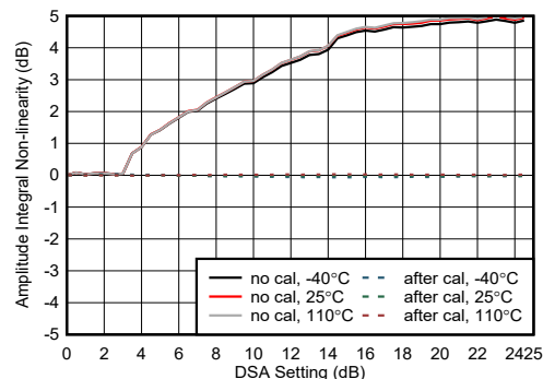
图 4-452. 9.6GHz 条件下 RX 振幅积分非线性
