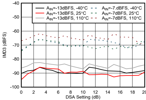
图 4-457. 9.6GHz 条件下 RX IMD3 与 DSA 设置间的关系
