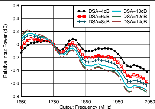
图 4-316. RX 带内增益平坦度， f_{\text{IN}} = 1750\text{MHz}
