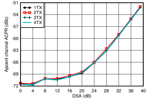
图 4-71. 1.8GHz 条件下 TX 20MHz LTE ACPR 与 DSA 间的关系
