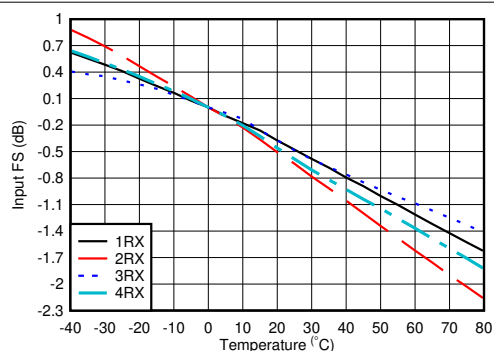
图 4-394. 4.9GHz 条件下 RX 输入满量程与温度和通道间的关系
