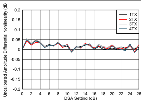
图 4-236. TX DSA 未校准振幅微分非线性
