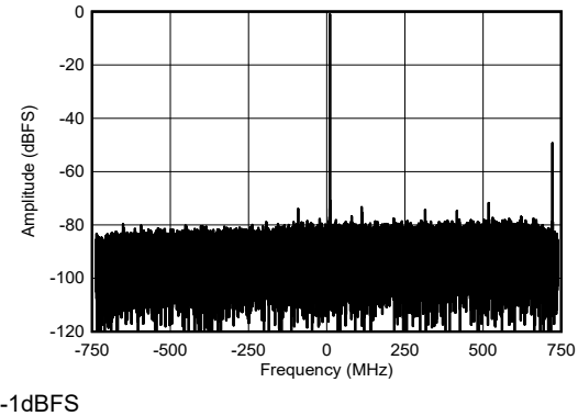
图 4-466. 9.61GHz 条件下 RX 单音输出 FFT
