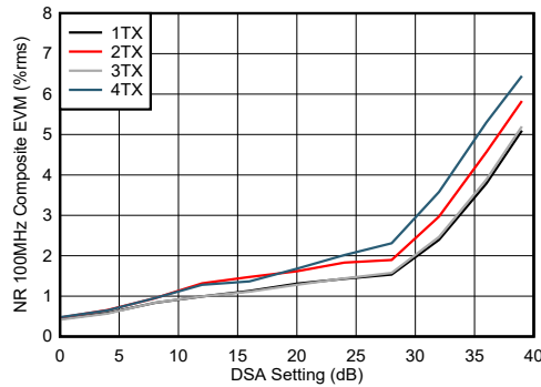
图 4-228. 8.1GHz 条件下 TX NR100MHz EVM 与 DSA 设置间的关系
