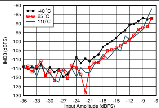
图 4-409. 4.9GHz 条件下 RX IMD3 与输入电平和温度间的关系
