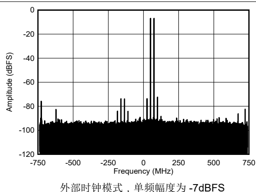
图 4-445. 8.1GHz 条件下 RX 双音输出 FFT
