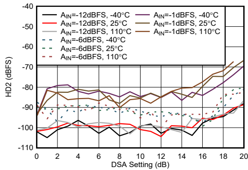
图 4-463. 9.6GHz 条件下 RX HD2 与 DSA 设置间的关系
