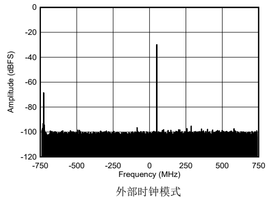
图 4-443. 8.11GHz 条件下 RX 单频输出 FFT, -30dBFS
