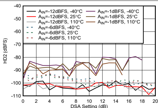
图 4-437. 8.1GHz 条件下 RX HD2 与 DSA 设置间的关系
