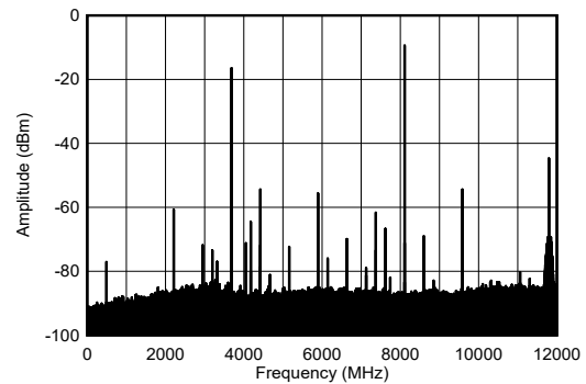
图 4-203. 8.1GHz 条件下 TX 单音输出频谱
