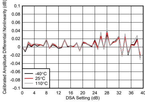
图 4-190. 8.1GHz 条件下 TX DSA 已校准振幅微分非线性
