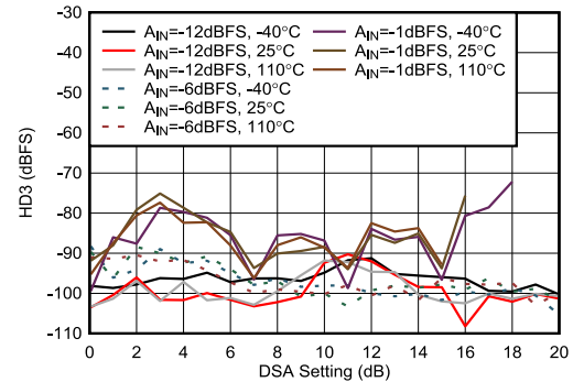
图 4-439. 8.11GHz 条件下 RX HD3 与 DSA 设置间的关系
