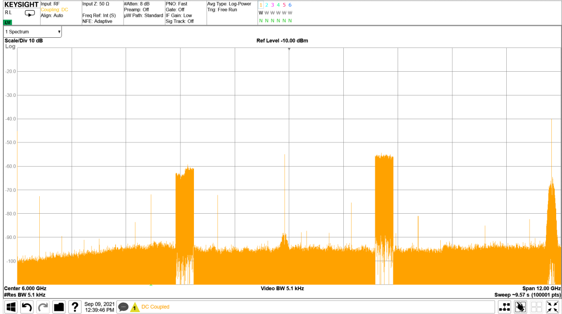
图 4-232. 8.1GHz 条件下 TX 4x100MHz NR 输出频谱
