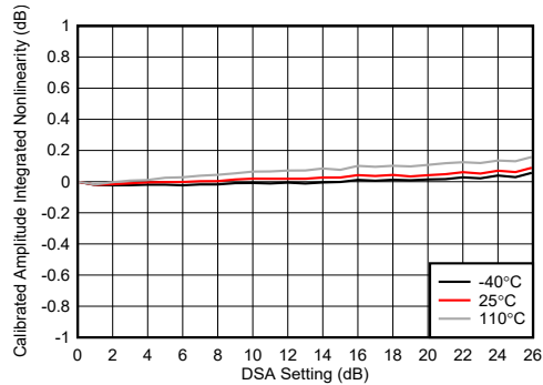
图 4-243. TX DSA 已校准振幅积分非线性
