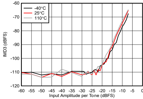
图 4-455. 9.6GHz 条件下 RX IMD3 与数字振幅间的关系
