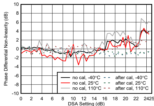
图 4-454. 9.6GHz 条件下 RX 相位微分非线性
