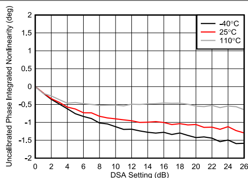
图 4-250. TX DSA 未校准相位积分非线性
