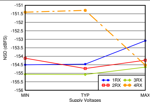
图 4-421. 4.9GHz 条件下 RX 噪声频谱密度与电源和通道间的关系
