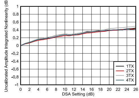
图 4-240. TX DSA 未校准振幅积分非线性
