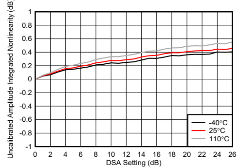
图 4-242. TX DSA 未校准振幅积分非线性
