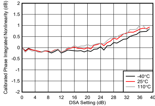
图 4-202. 8.1GHz 条件下 TX DSA 已校准相位积分非线性
