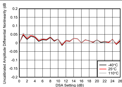
图 4-238. TX DSA 未校准振幅微分非线性
