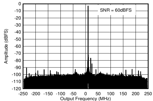
图 4-404. 4.9GHz 条件下的 RX 输出 FFT
