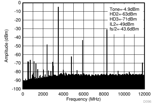
图 4-147. 3.5GHz (0 - f_{\text{DAC}} ) 条件下的 TX 单频 (-6dBFS) 输出频谱
