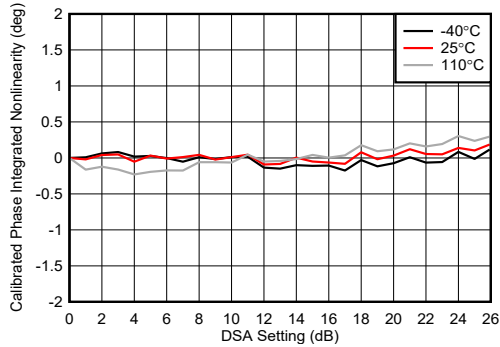
图 4-251. TX DSA 已校准振幅积分非线性
