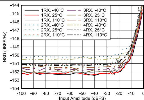
图 4-432. 8.1GHz 条件下 RX NSD 与数字振幅间的关系
