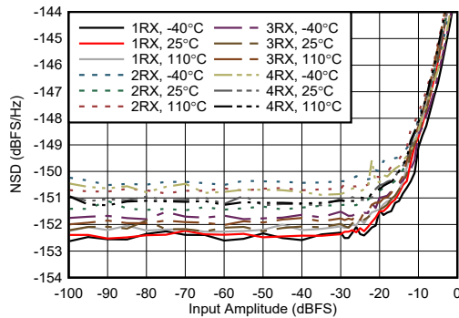
图 4-459. 9.6GHz 条件下 RX NSD 与数字振幅间的关系
