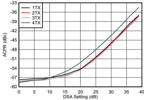
图 4-226. 8.1GHz 条件下 TX NR100MHz ACPR 与 DSA 设置间的关系
