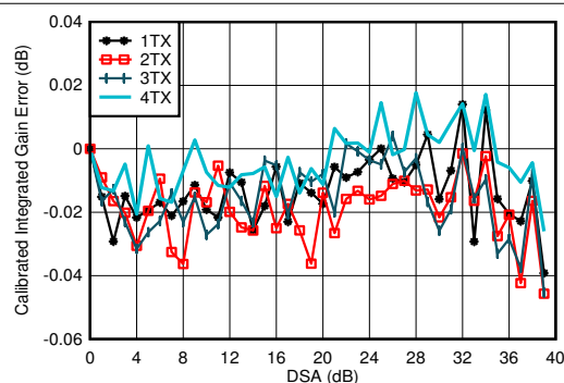
图 4-121. 3.5GHz 条件下 TX 校准差分增益误差与 DSA 设置和通道间的关系
