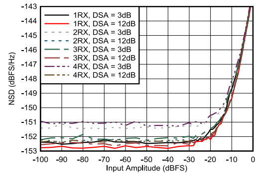
图 4-460. 9.6GHz 条件下 RX NSD 与数字振幅间的关系
