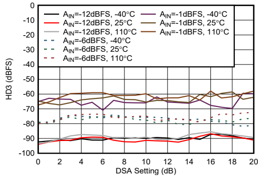
图 4-465. 9.6GHz 条件下 RX HD3 与 DSA 设置间的关系
