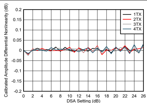
图 4-237. TX DSA 已校准振幅微分非线性
