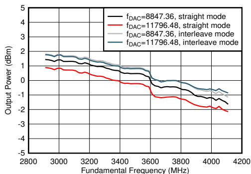
图 4-118. TX 输出功率与频率间的关系
