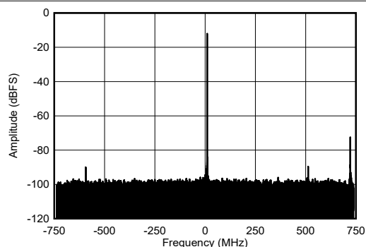
图 4-468. 9.61GHz 条件下 RX 单音输出 FFT
