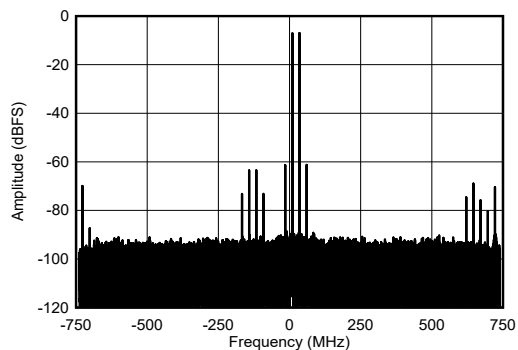
图 4-469. 9.61GHz 条件下 RX 单音输出 FFT
