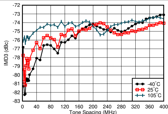
图 4-25. 0.85GHz 条件下 TX IMD3 与频率间隔和温度间的关系
