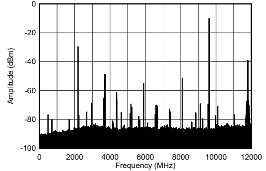
图 4-266. 9.61GHz 和 -1dBFS (宽带) 条件下的 TX 单音频谱
