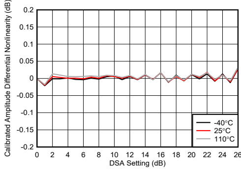
图 4-239. TX DSA 已校准振幅微分非线性
