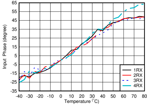
图 4-395. f_{\text{OUT}} = 4.9\text{GHz} 时 RX 输入相位与温度和 DSA 间的关系
