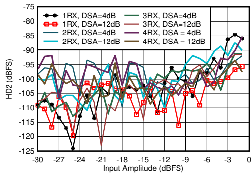
图 4-334. 1.9GHz 条件下 RX HD2 与 DSA 设置和通道间的关系
