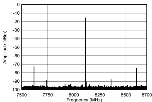
图 4-208. 8.1GHz 条件下 TX 单音输出频谱
