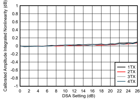
图 4-241. TX DSA 已校准振幅积分非线性
