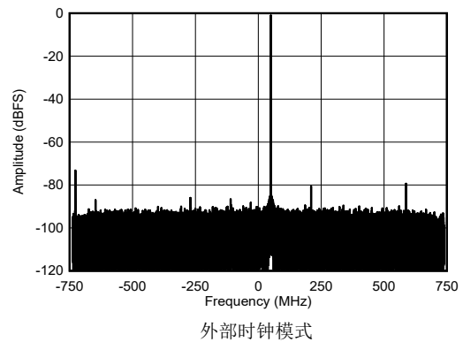
图 4-441. 8.11GHz 条件下 RX 单频输出 FFT, -1dBFS
