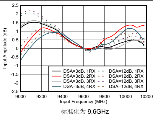
图 4-449. RX 输入振幅与频率间的关系
