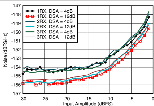
图 4-299. 0.8GHz 条件下 RX 噪声频谱密度与输入振幅和通道间的关系
