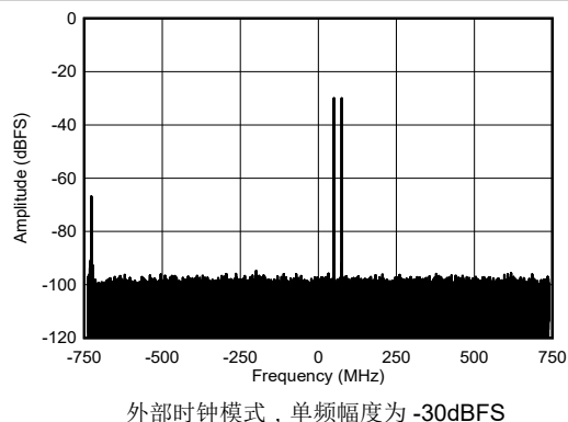
图 4-447. 8.1GHz 条件下 RX 双音输出 FFT
