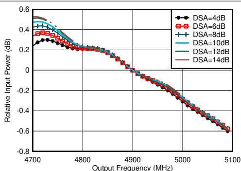
图 4-393. RX 带内增益平坦度， f_{\text{IN}} = 4900\text{MHz}
