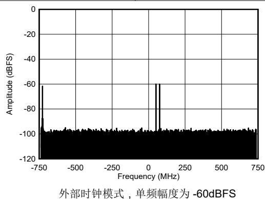
图 4-448. 8.1GHz 条件下 RX 双音输出 FFT
