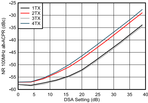
图 4-281. 9.61GHz 条件下 TX NR 100MHz ACPR 与 DSA 设置间的关系 9.61GHz 条件下 TX NR 100MHz alt-ACPR 与 DSA 设置间的关系
