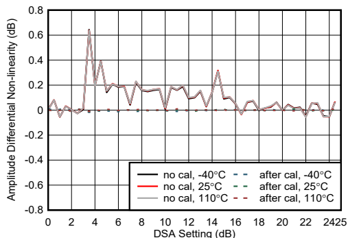
图 4-451. 9.6GHz 条件下 RX 振幅微分非线性
