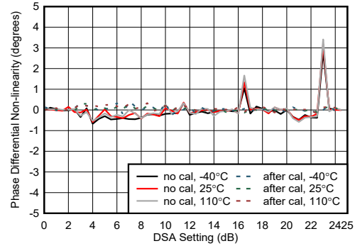
图 4-427. 8.1GHz 条件下 RX 相位微分非线性
