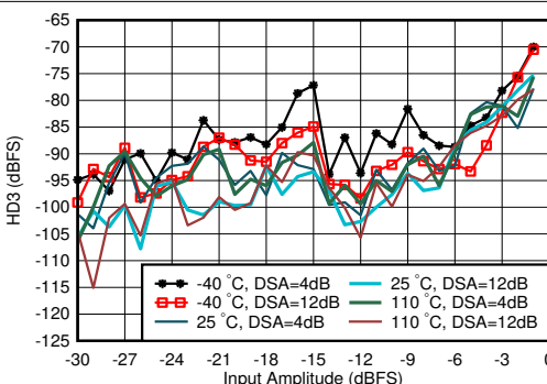
图 4-309. 0.8GHz 条件下 RX HD3 与 DSA 设置和温度间的关系
