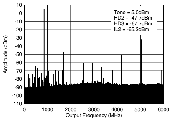
图 4-43. 0.85GHz ( 0-f_{\text{DAC}} ) 条件下的 TX 单频 (-1dBFS) 输出频谱
