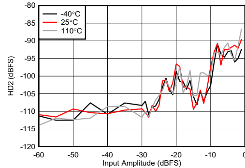
图 4-462. 9.6GHz 条件下 RX HD2 与数字电平间的关系
