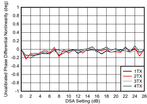
图 4-244. TX DSA 未校准相位微分非线性
