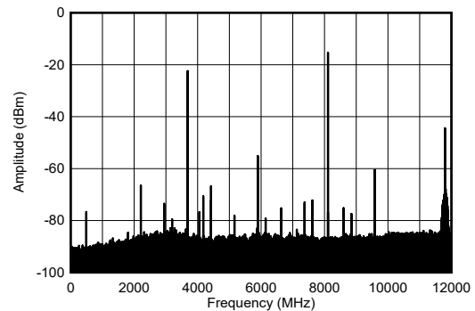
图 4-205. 8.1GHz 条件下 TX 单音输出频谱
