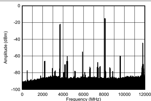
图 4-209. 8.1GHz 条件下 TX 双音输出频谱
