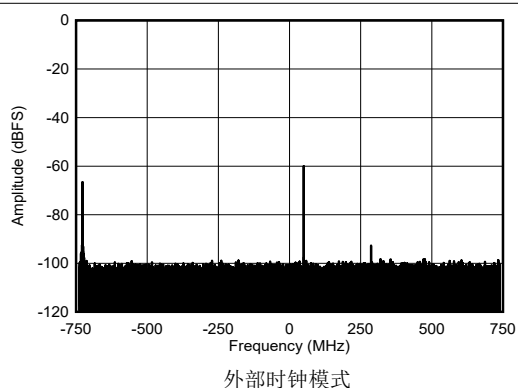
图 4-444. 8.1GHz 条件下 RX 单频输出 FFT, -60dBFS
