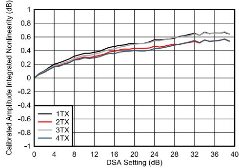
图 4-192. 8.1GHz 条件下 TX DSA 已校准振幅积分非线性
