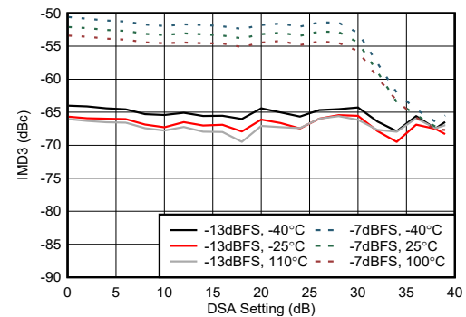
图 4-254. 9.61GHz 条件下 TX IMD3 与 DSA 设置间的关系
