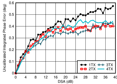
图 4-126. 3.5GHz 条件下 TX 未校准积分相位误差与 DSA 设置和通道间的关系
