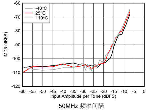
图 4-429. 8.11 GHz 条件下 RX IMD3 与输入振幅间的关系
