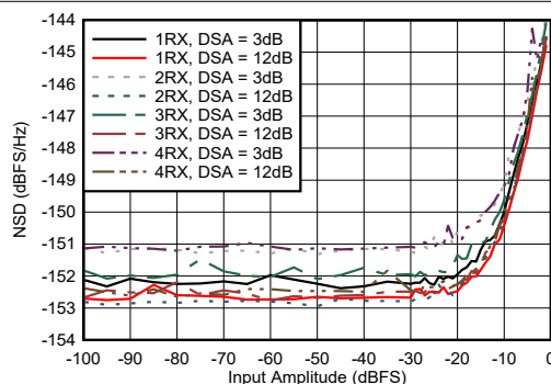
图 4-433. 8.1GHz 条件下 RX NSD 与数字振幅间的关系
