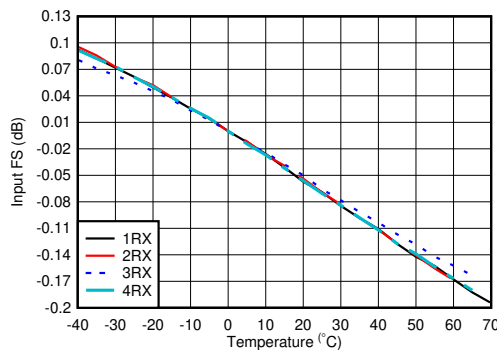
图 4-286. 800MHz 条件下 RX 输入满量程与温度和通道间的关系
