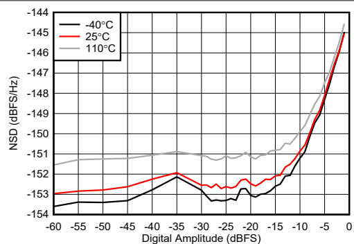
图 4-261. 9.61GHz 条件下 TX NSD 与数字振幅间的关系
