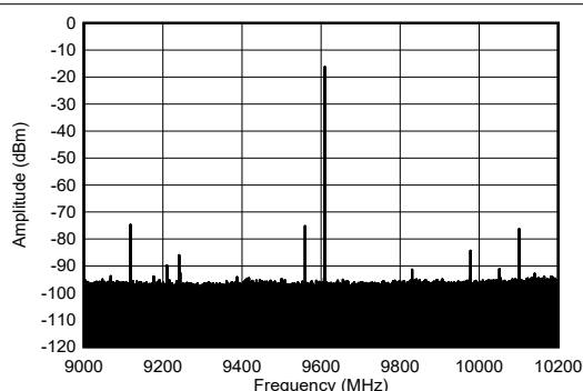
图 4-269. 9.61GHz 和 -6dBFS (1.2GHz 带宽) 条件下的 TX 单音频谱
