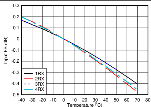
图 4-317. 1.75GHz 条件下 RX 输入满量程与温度和通道间的关系
