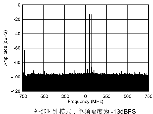
图 4-446. 8.1GHz 条件下 RX 双音输出 FFT
