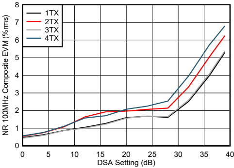
图 4-282. 9.61GHz 条件下 TX NR100MHz EVM 与 DSA 设置间的关系
