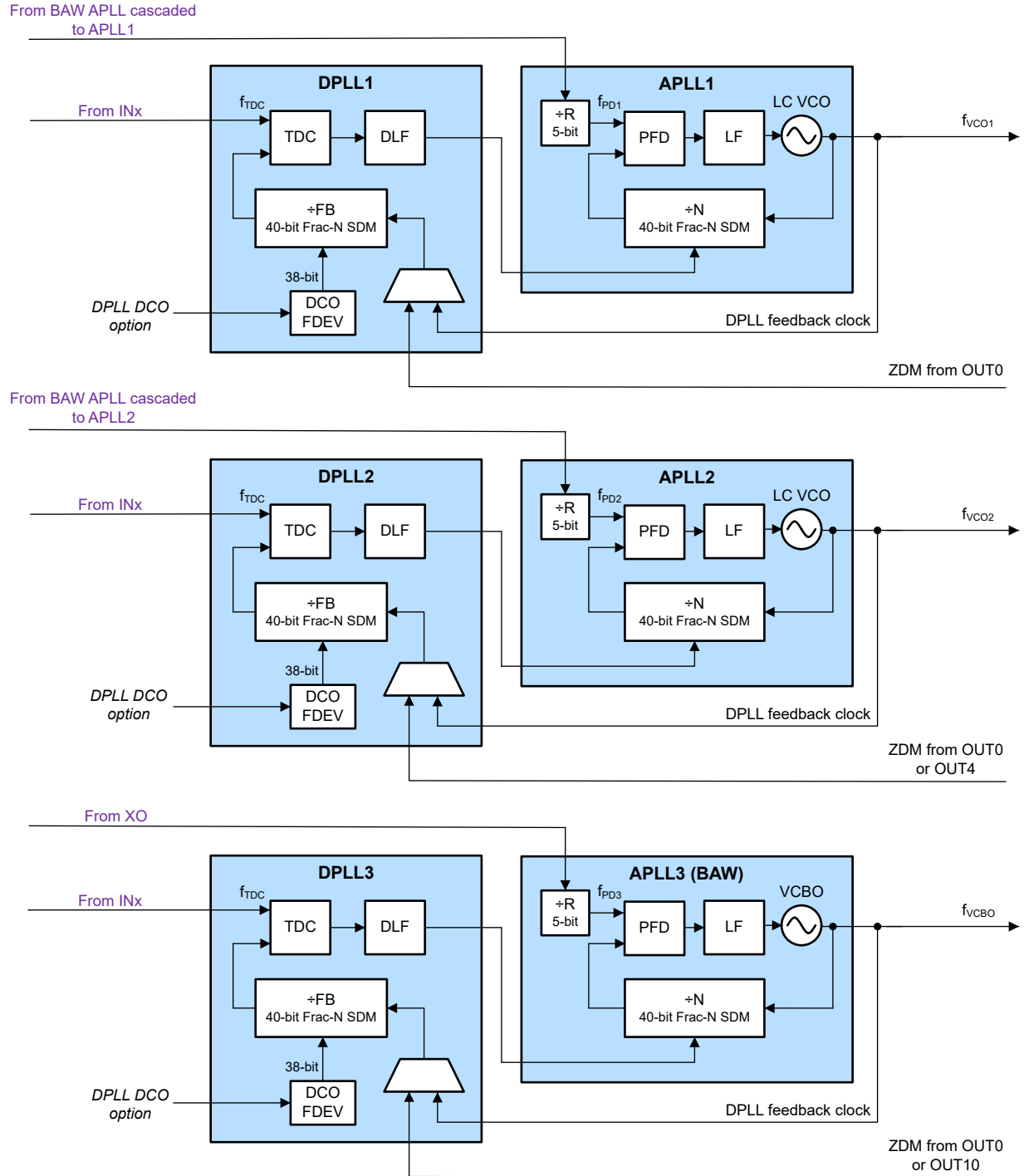
图 8-5. 启用 DPLL 的 APLL 级联示例
