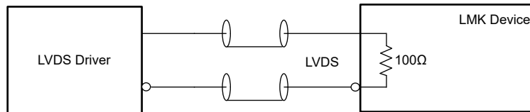
图 8-12. 直流耦合 HSDS/LVDS 至基准 (INx)
