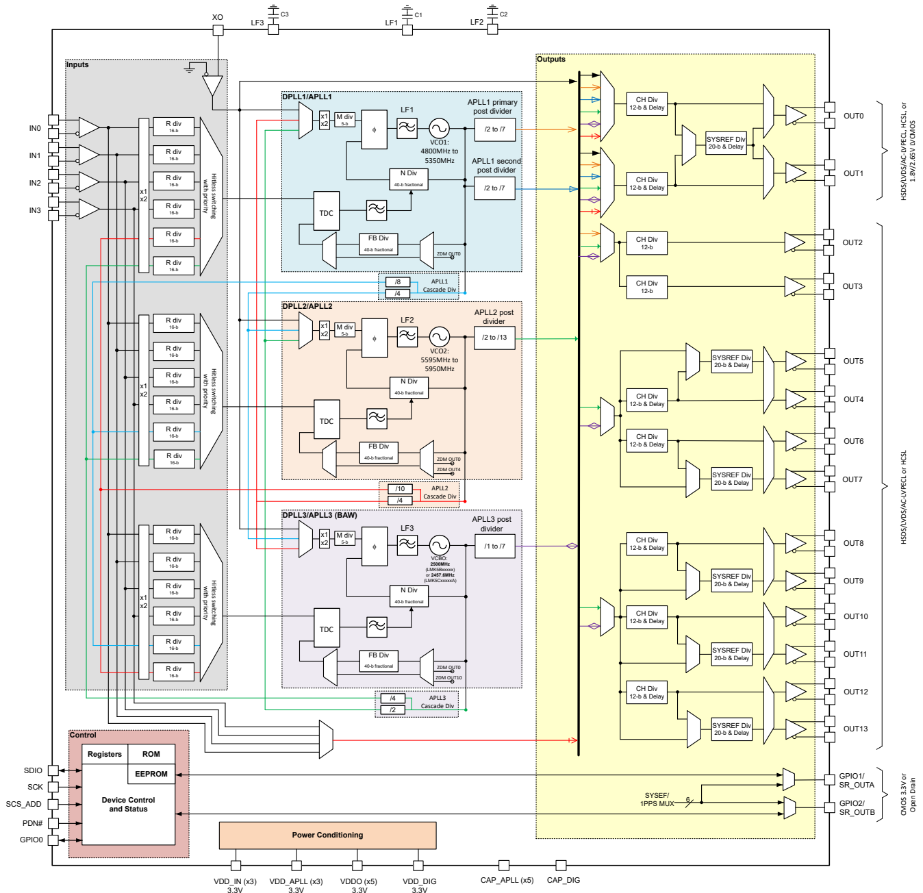
图 8-1. LMK5B33414 顶层方框图
