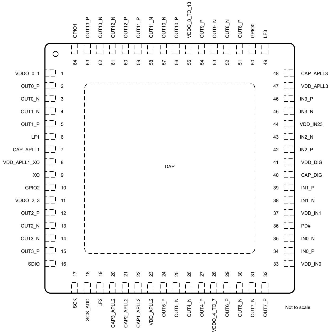
图 5-1. LMK5B33414 RGC 封装 64 引脚 VQFN 顶视图
