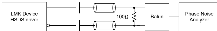
图 7-6. HSDS 输出相域测试配置
