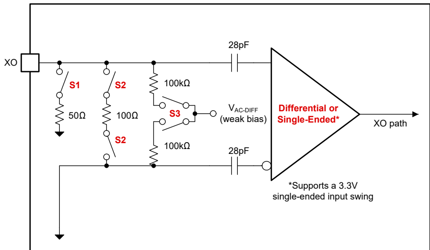
图 8-8. XO 输入缓冲器
