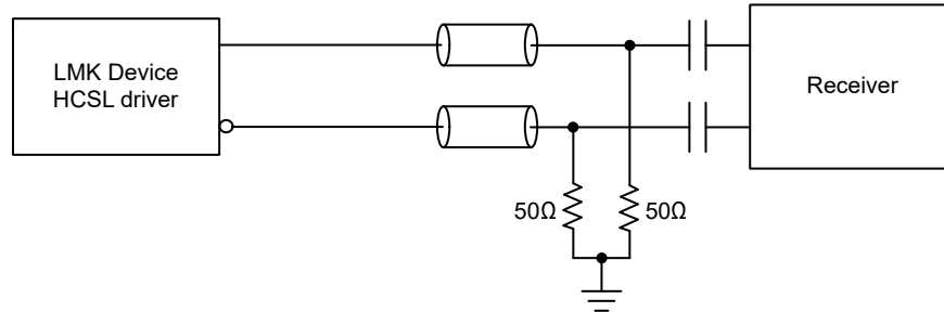
图 8-31. 交流耦合 HCSL 输出端接
