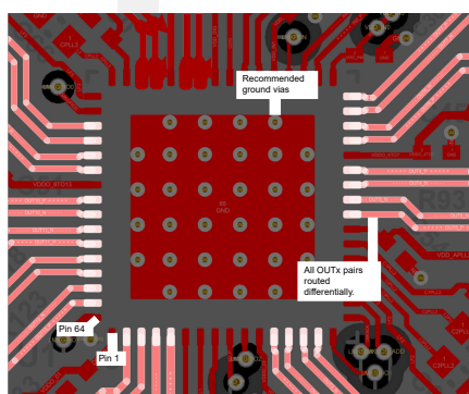
图 9-6. LMK5B33414 的 PCB 布局示例, 顶层
