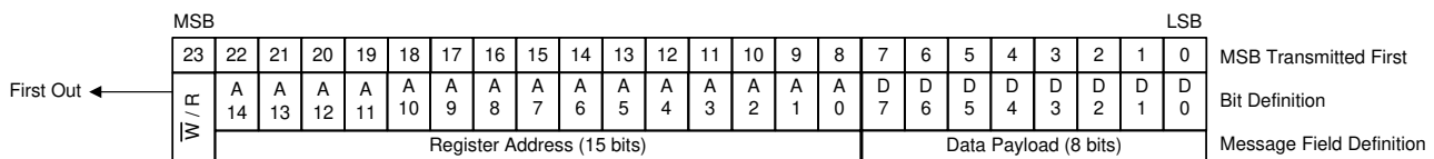
图 8-44. SPI 消息格式
