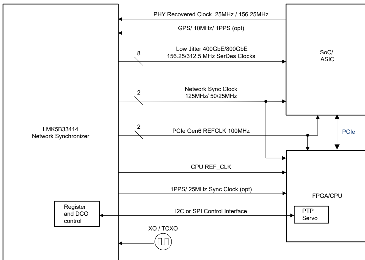
LMK5B33414 典型系统方框图
