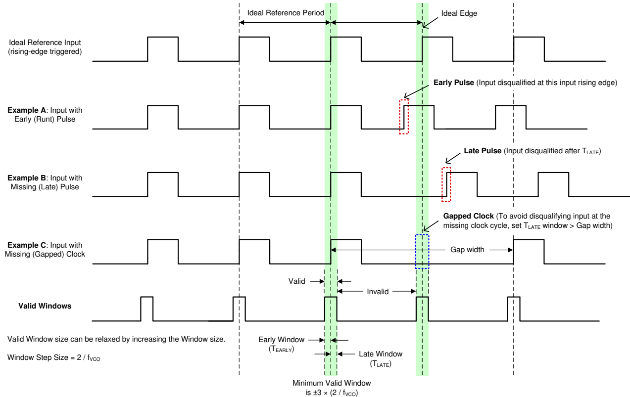
图 8-18. 早期和晚期窗口检测器示例
