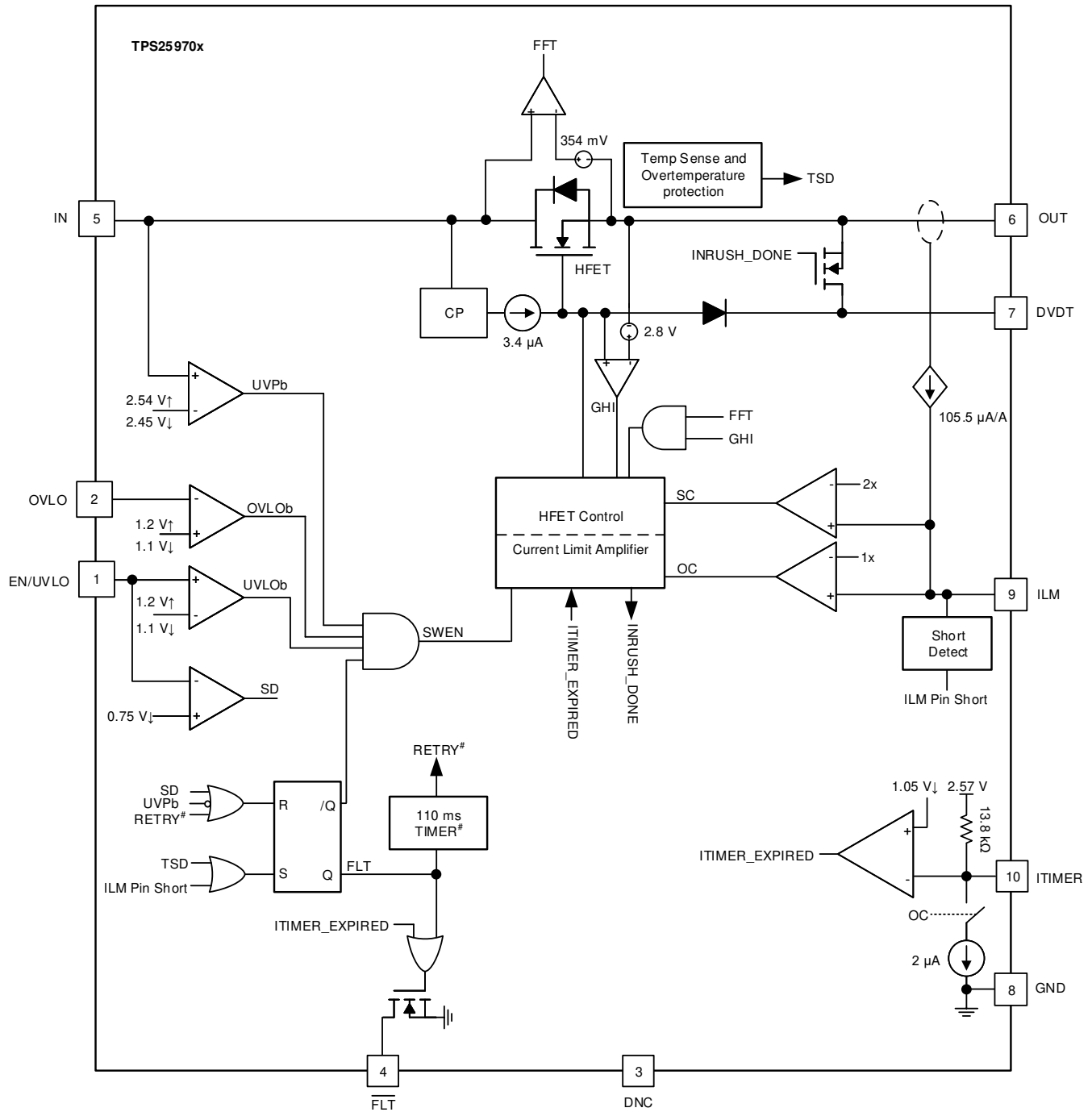
图 7-1. TPS25970x Block Diagram
