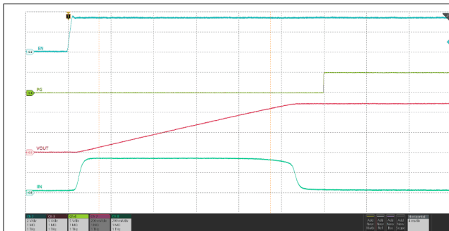
图 8-4. Power Up
