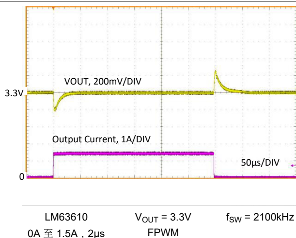
图 8-14. 负载瞬态
