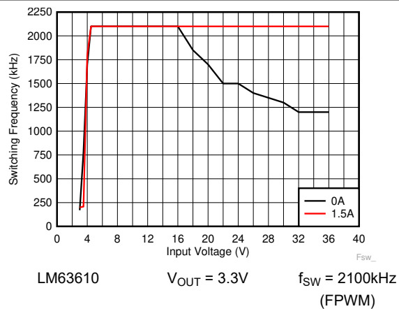
图 8-12. 开关频率与输入电压间的关系
