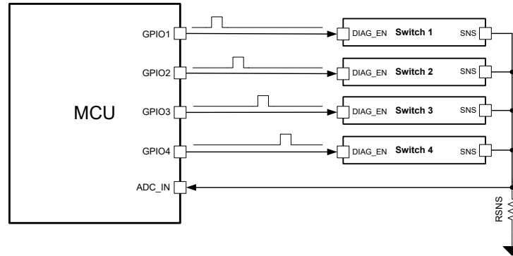
图 8-20. 电阻器共享
