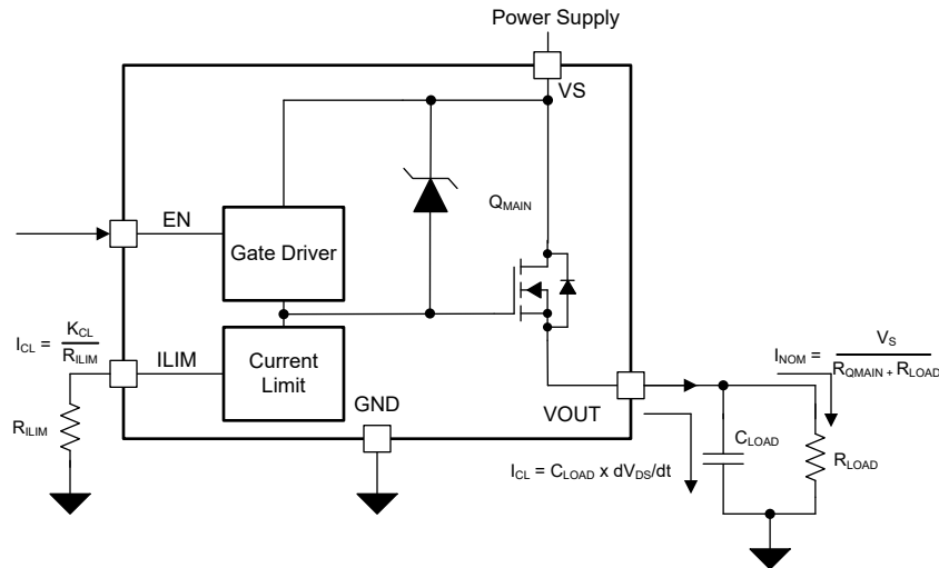
图 8-7. 电容充电电路
