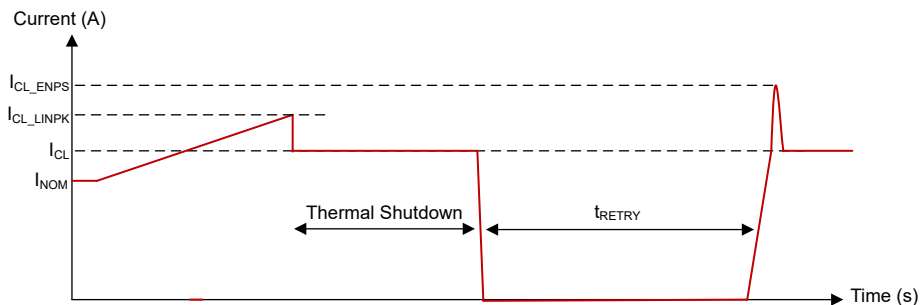
图 8-6. 过载行为
