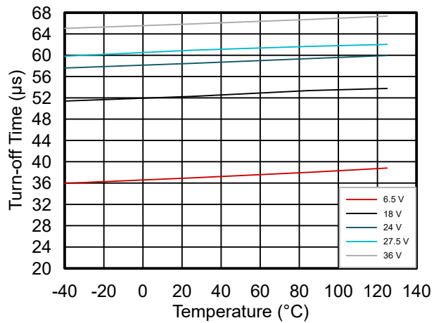
图 6-13. 关断时间 ( t_{\text{OFF}} ) 与温度与 VS 电压间的关系
