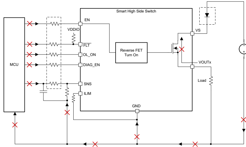
图 8-17. 采用阻断二极管实现反向保护
