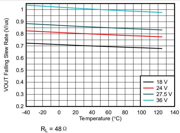
图 6-15. VOUT 下降压摆率 ( \text{SR}_F ) 与温度与 VS 电压间的关系
