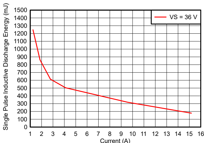
图 8-14. TPS1HTC30 在 125°C 下的电感负载放电能量能力
