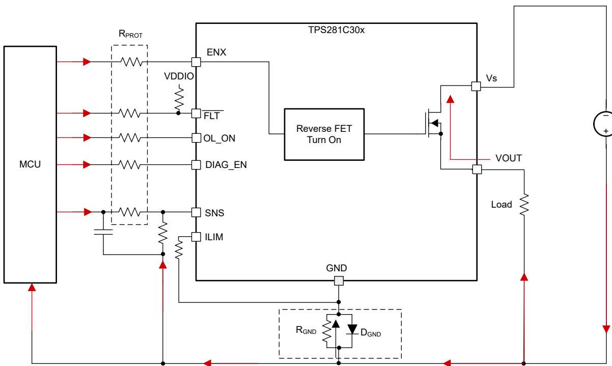
图 8-19. MCU IO 保护
