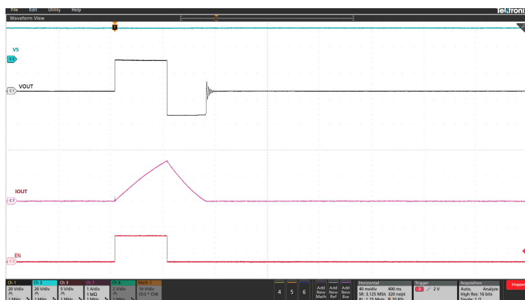
图 8-13. TPS1HTC30 电感放电 (400mH)
