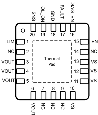
图 5-1. RGW 封装，20 引脚 QFN（顶视图）
