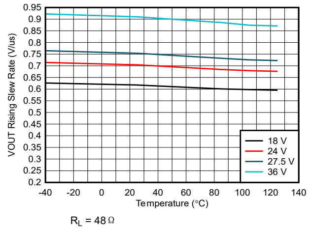
图 6-14. VOUT 上升压摆率 ( \text{SR}_R ) 与温度与 VS 电压间的关系
