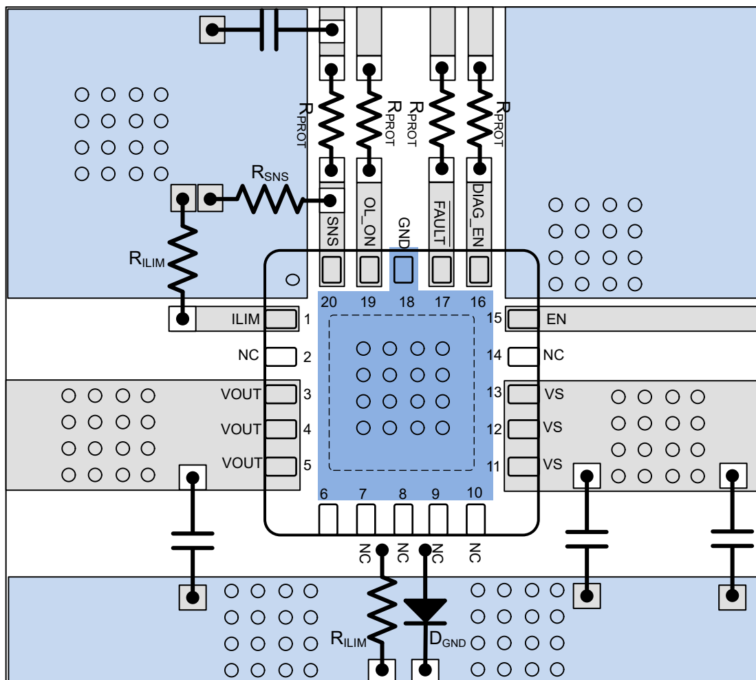
图 9-2. 采用接地网络的 RGW 布局
