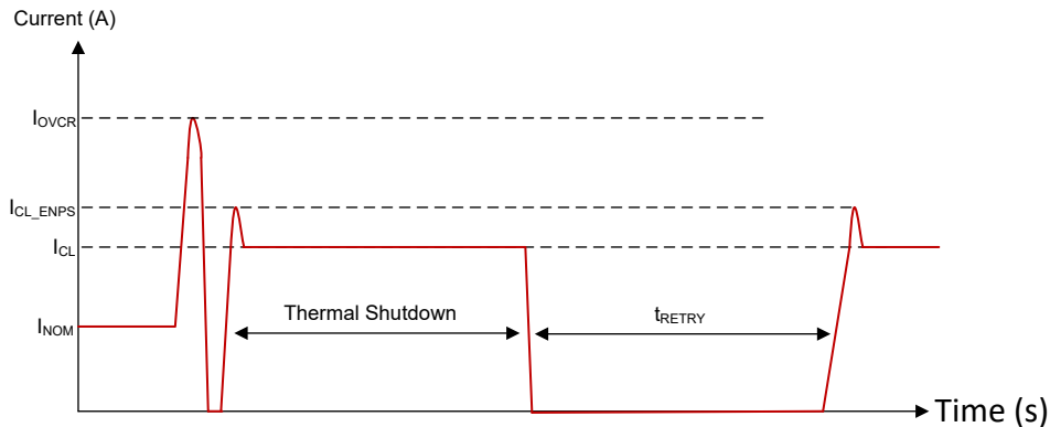
图 8-5. 导通状态短路行为
