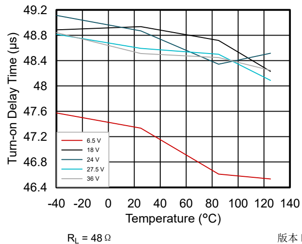
图 6-7. 导通延迟时间 ( t_{DR} ) 与温度与 VS 电压间的关系
