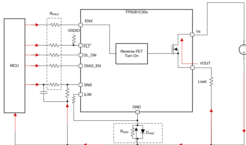
图 8-18. 通过接地网络实现反向保护
