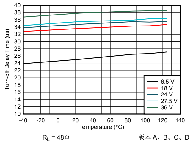
图 6-8. 关断延迟时间 ( t_{DF} ) 与温度与 VS 电压间的关系
