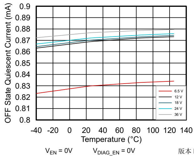
图 6-5. 来自 VS 输入电源的关断状态静态电流 ( I_{Q(OFF)} ) 与温度和 VS 电压间的关系
