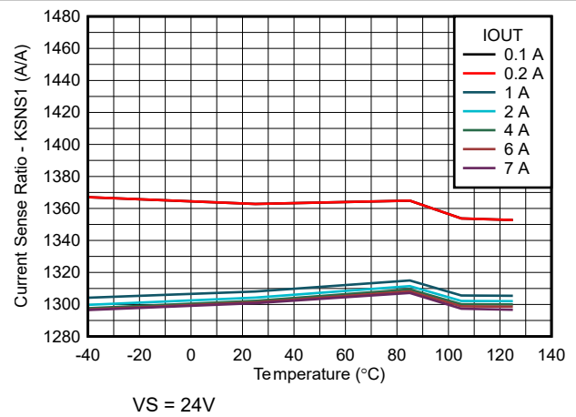
图 6-16. 电流检测比 ( \text{KSNS}_1 ) 与温度与负载电流间的关系
