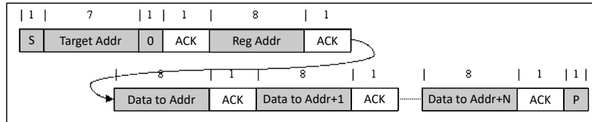
图 7-23. 多重写入
