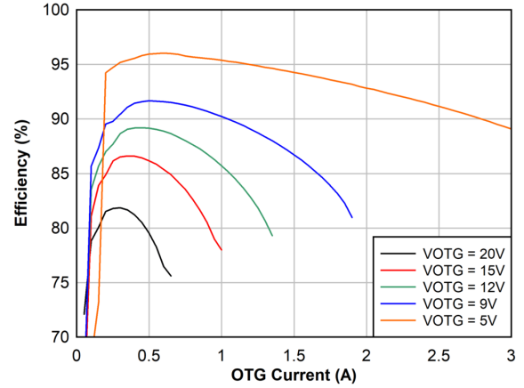
图 6-10. 1 节电池 OTG 效率, 1.5MHz
