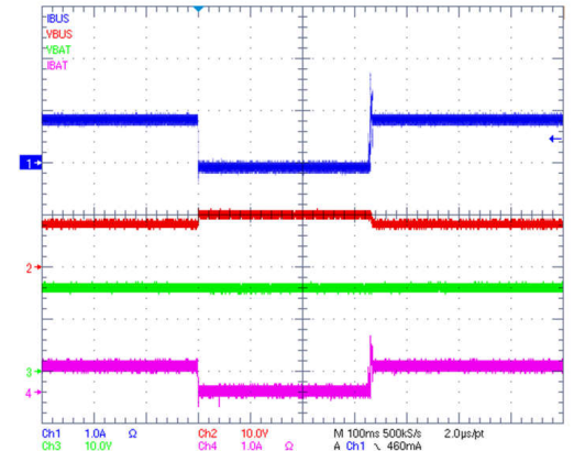
图 8-17. VOTG 负载瞬态响应
