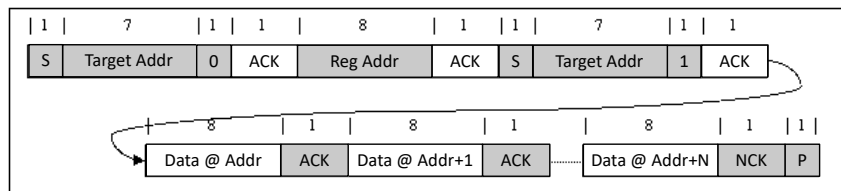
图 7-24. 多重读取
