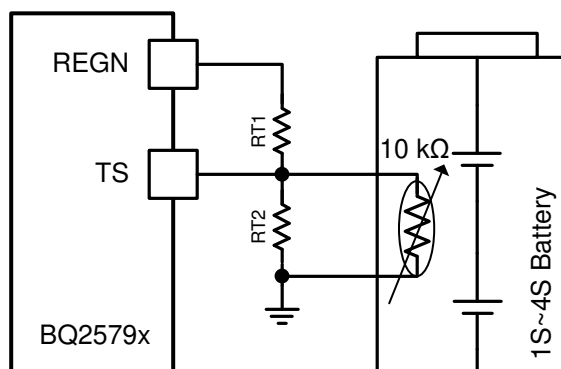
图 7-12. TS 电阻器网络
