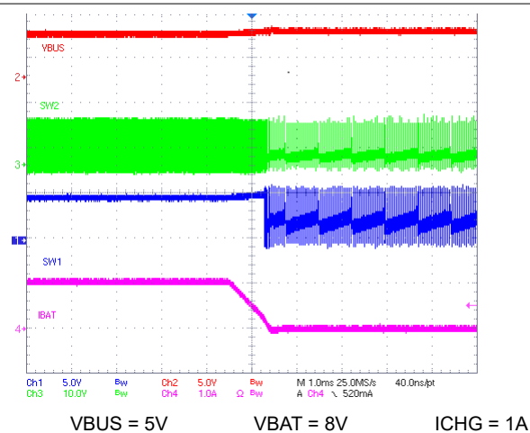
图 8-7. 充电禁用
