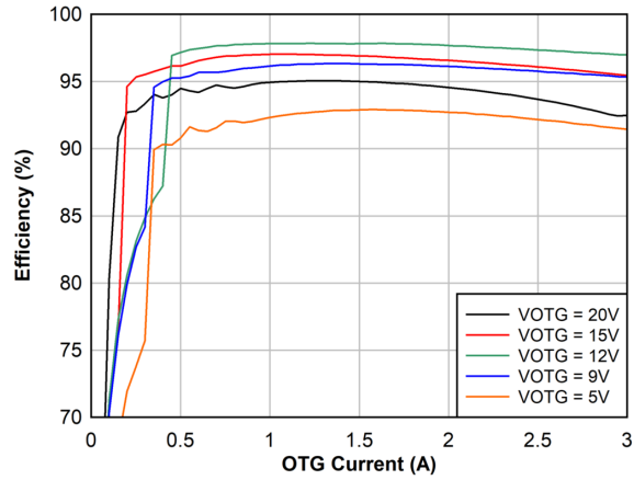
图 6-13. 3s 电池 OTG 效率, 750kHz
