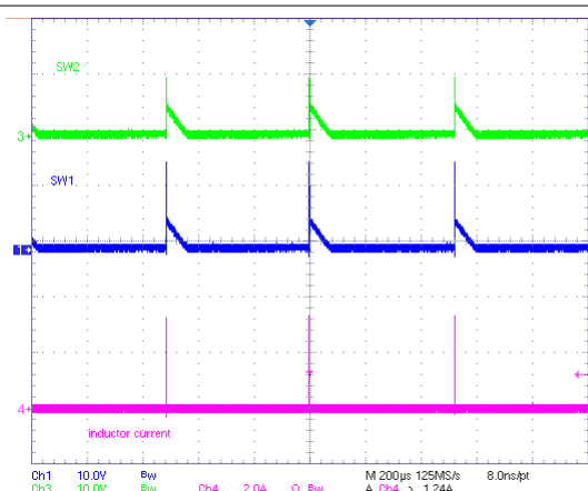
图 8-10. 降压充电模式 PWM 运行
