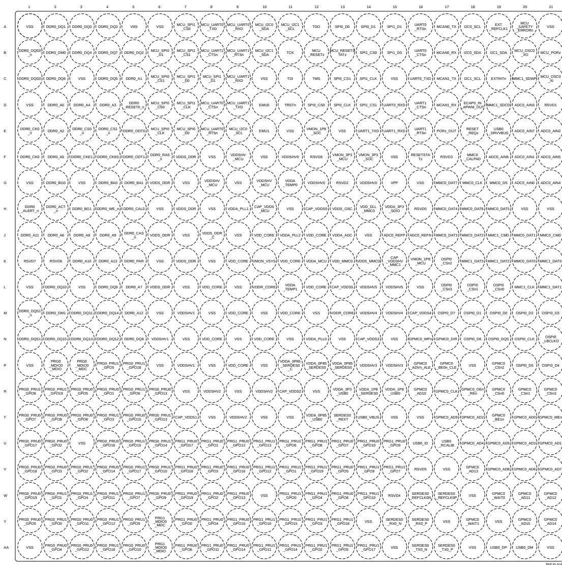
图 5-1. ALV/ANI FCBGA-N441 引脚图 (顶视图)
