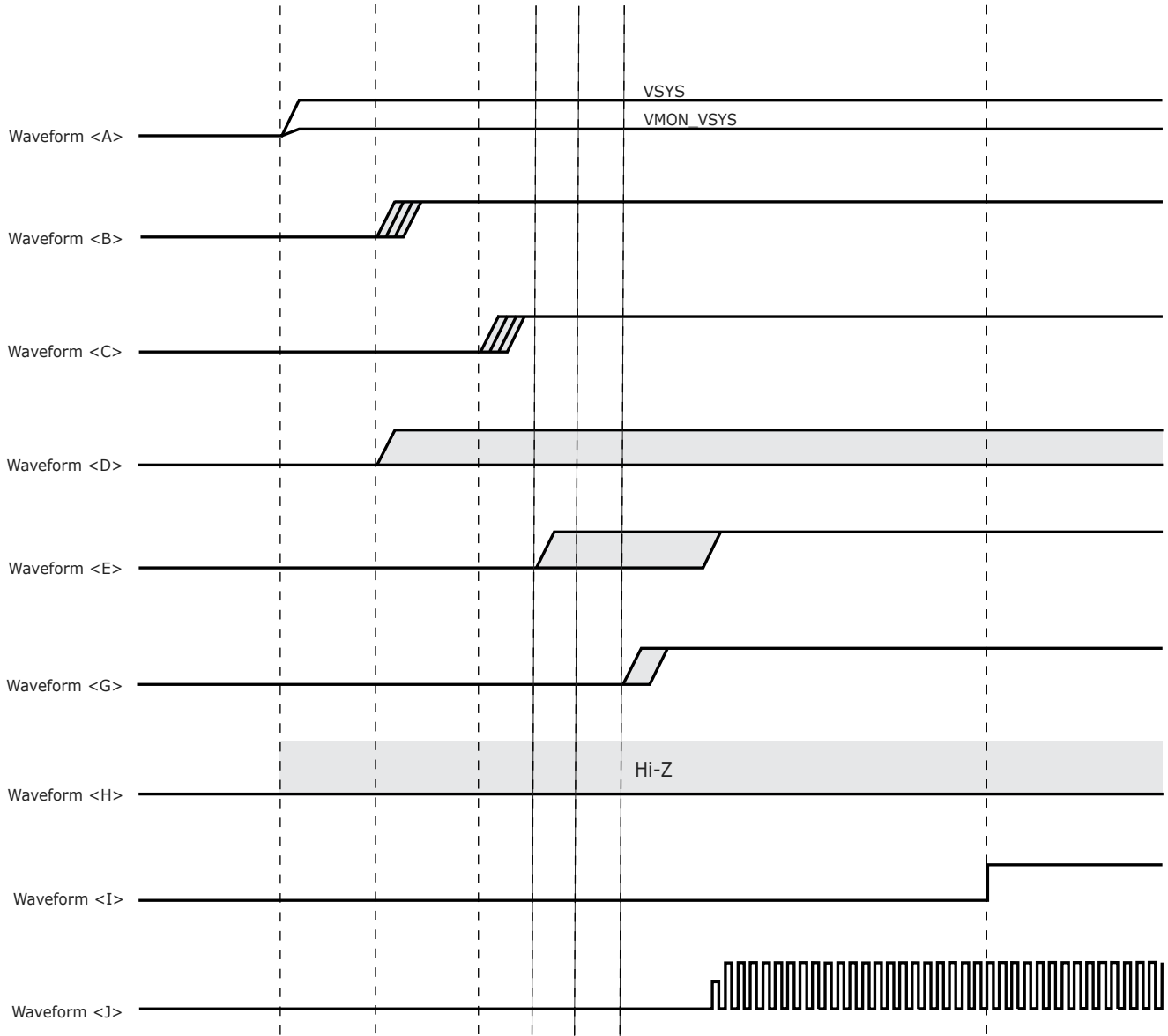
图 6-5. 上电时序
