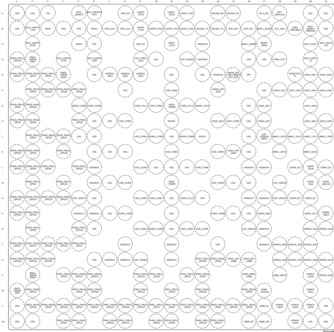
图 5-2. ALX FCBGA-N293 引脚图 (顶视图)
