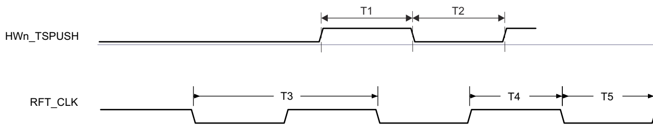
图 6-77. CPTS 时序要求
