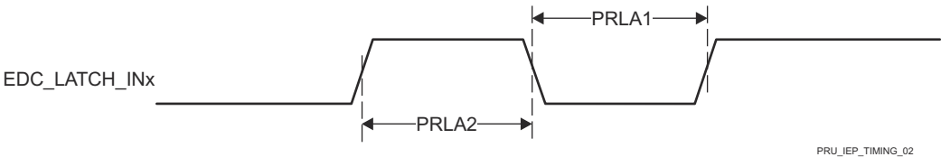
图 6-102. PRU_ICSSG IEP LATCH_INx 时序要求
