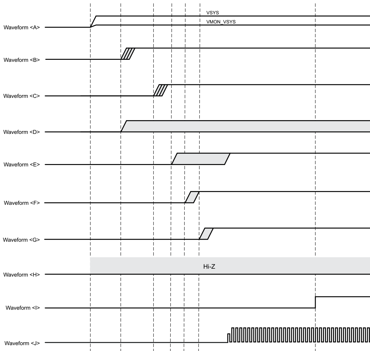
图 6-5. 上电时序
