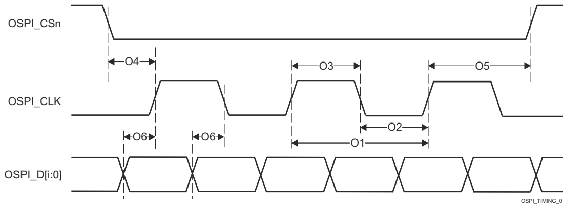
图 6-80. OSPI0 开关特性 - PHY DDR 数据训练
