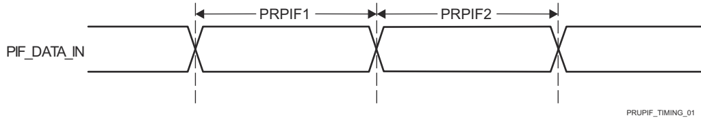
图 6-97. PRU_ICSSG PRU 外设接口时序要求
