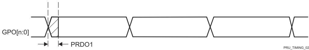
图 6-90. PRU_ICSSG PRU 直接输出时序
