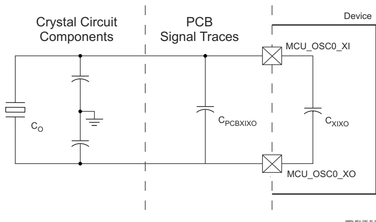
图 6-20. 并联电容
