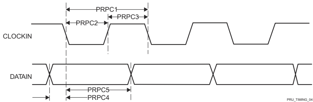
图 6-92. PRU_ICSSG PRU 并行捕获时序要求 - 下降沿模式
