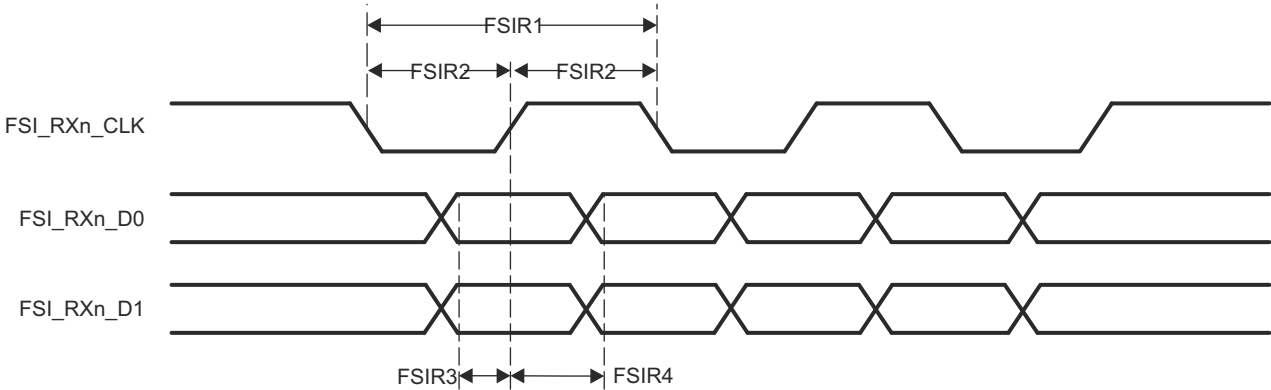
图 6-36. FSI 时序要求
