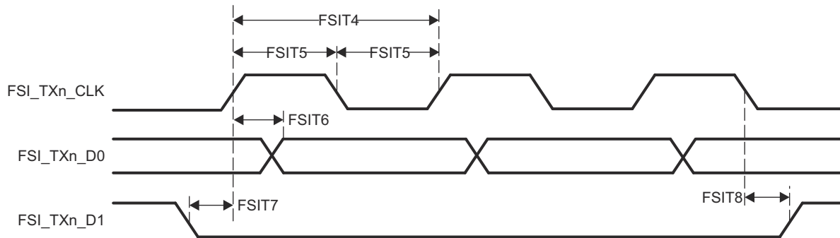
图 6-38. FSI 开关特性 - SPI 模式
