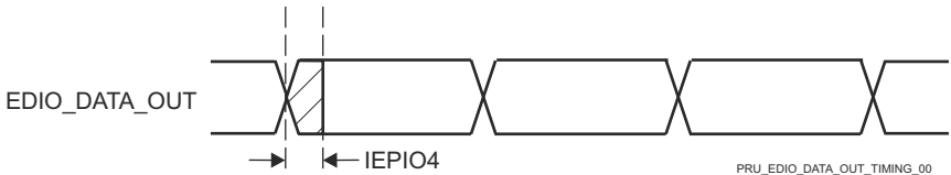
图 6-101. PRU_ICSSG IEP 数字 IO 时序要求
