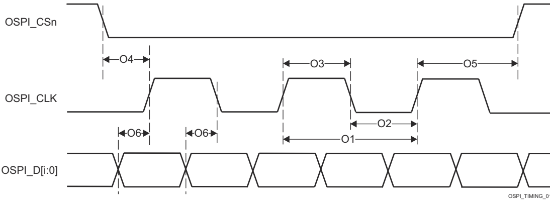
图 6-80. OSPI0 开关特性 - PHY DDR 数据训练
