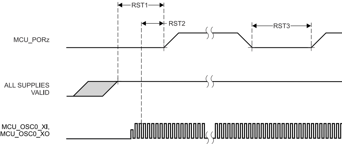
图 6-7. MCU_PORz 时序要求
