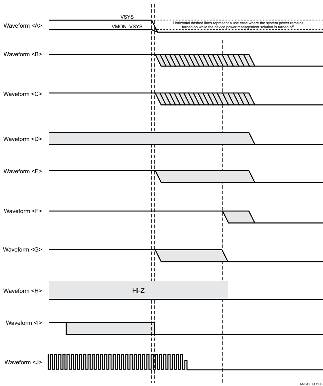
图 6-6. 下电时序
