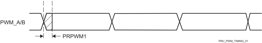
图 6-99. PRU_ICSSG PWM 时序
