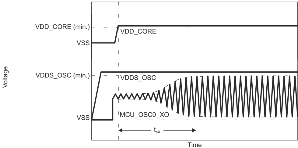
图 6-18. MCU_OSC0 启动时间
