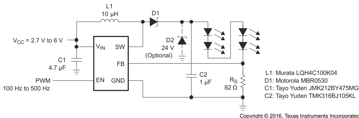
图 7-10. 具有可调亮度控制的白光 LED 电源在使能引脚上使用 PWM 信号，在 V_{IN} = 3V 条件下，效率约等于 86%， I_{LED} = 15mA
