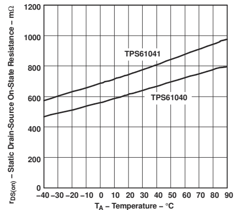
图 5-10. TPS6104x 静态漏源开启状态电阻与自然通风条件下的温度之间的关系
