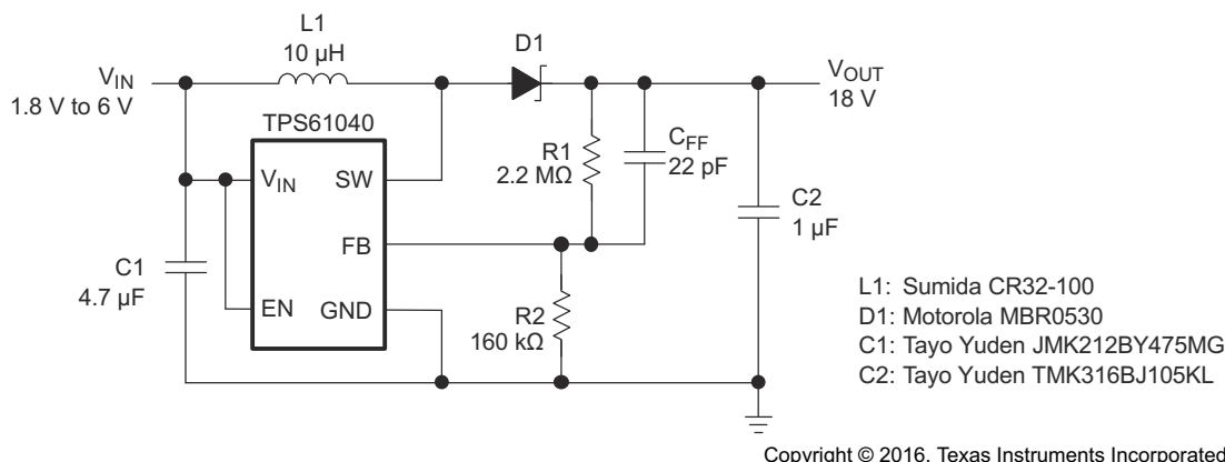
图 7-1. LCD 偏置电源
