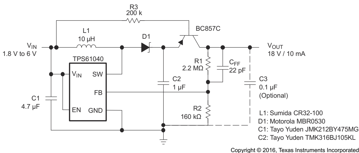
图 7-6. 具有负载断开功能的 LCD 偏置电源
