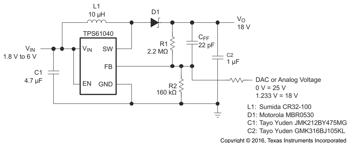
图 7-5. 具有可调输出电压的 LCD 偏置电源
