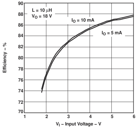
图 5-4. 效率与输入电压之间的关系
