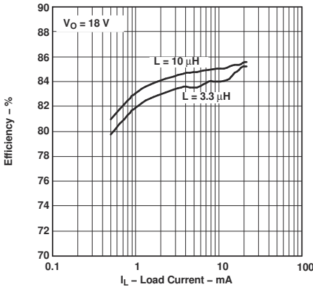
图 5-3. 效率与负载电流之间的关系
