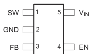
图 4-1. DDC 封装、DBV 封装 SOT 5 引脚 顶视图
