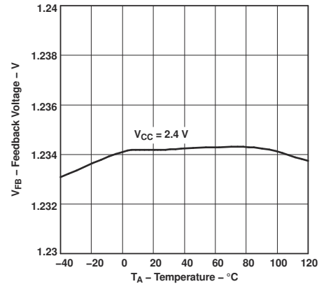
图 5-6. 反馈电压与自然通风条件下的温度之间的关系
