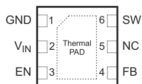
图 4-2. DRV 封装 WSON 6 引脚 透明顶视图
