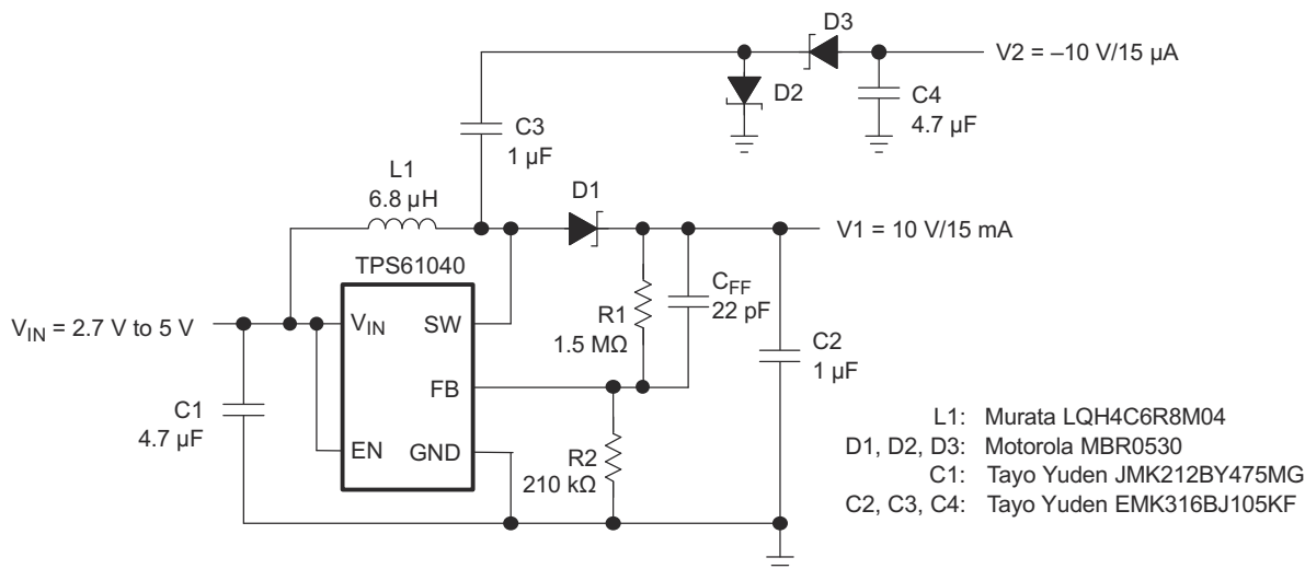
图 7-7. 正负输出 LCD 偏置电源
