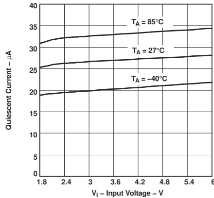
图 5-5. TPS61040 静态电流与输入电压之间的关系
