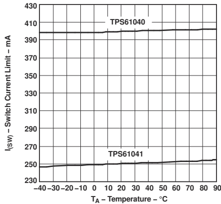
图 5-7. TPS6104x 开关电流限值与自然通风条件下的温度之间的关系
