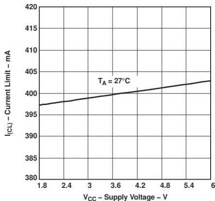
图 5-9. TPS61040 电流限值与电源电压之间的关系
