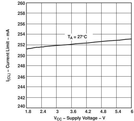
图 5-8. TPS61041 电流限值与电源电压之间的关系
