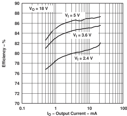
图 5-1. 效率与输出电流之间的关系
