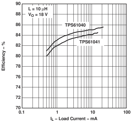
图 5-2. 效率与负载电流之间的关系
