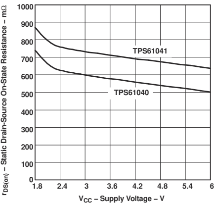
图 5-11. TPS6104x 静态漏源开启状态电阻与电压之间的关系
