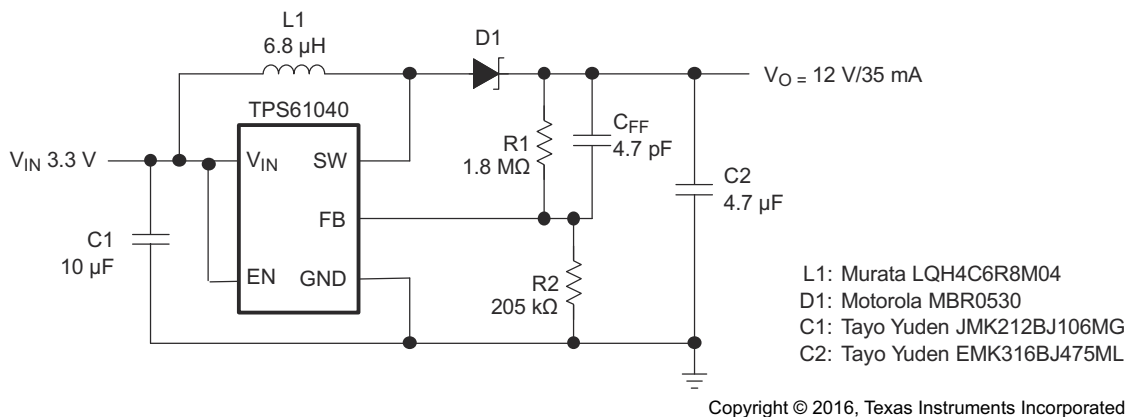
图 7-8. 标准 3.3V 至 12V 电源
