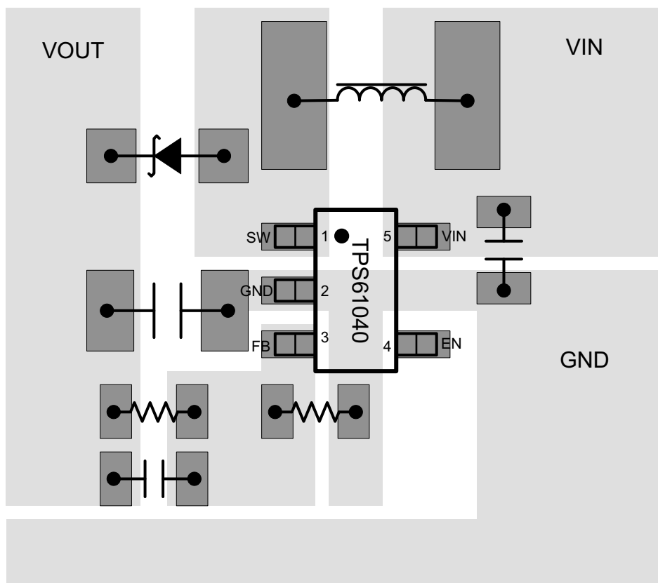
图 7-12. 布局图
