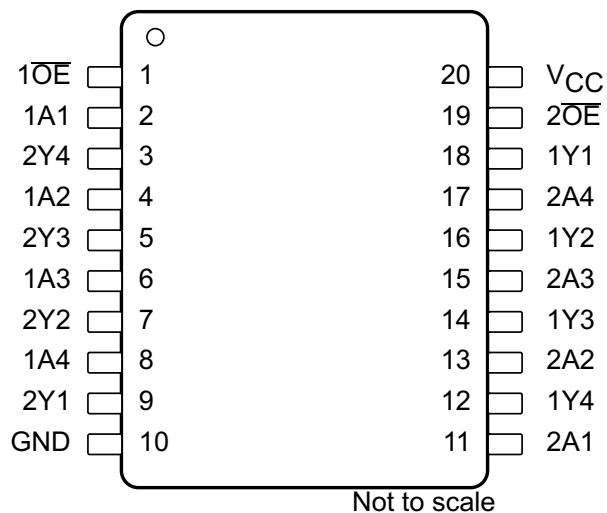
图 4-2. DB、DGV、DW、N、NS、DGS 和 PW 封装 20 引脚 SSOP、TVSOP、SOIC、PDIP、SO、VSSOP 和 TSSOP 前视图
