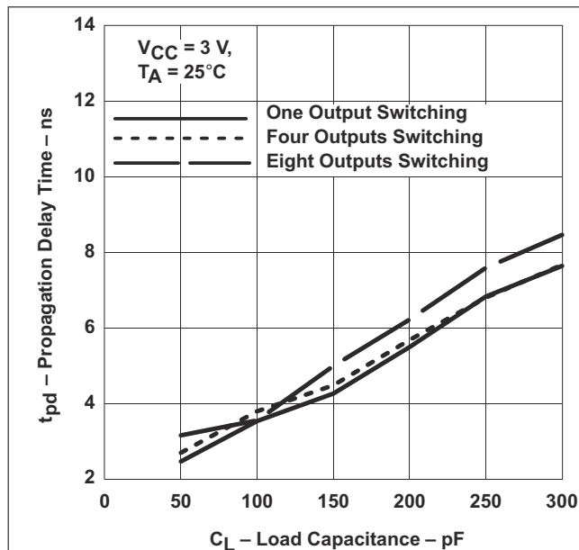
图 5-1. 传播延迟 (低电平至高电平转换) 与负载电容间的关系
