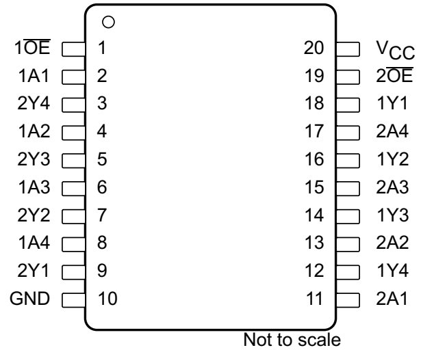
图 4-2. DB、DGV、DW、N、NS、DGS 和 PW 封装 20 引脚 SSOP、TVSOP、SOIC、PDIP、SO、VSSOP 和 TSSOP 前视图
