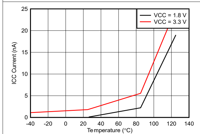
图 5-3. 睡眠模式 ICC 与温度间的关系
