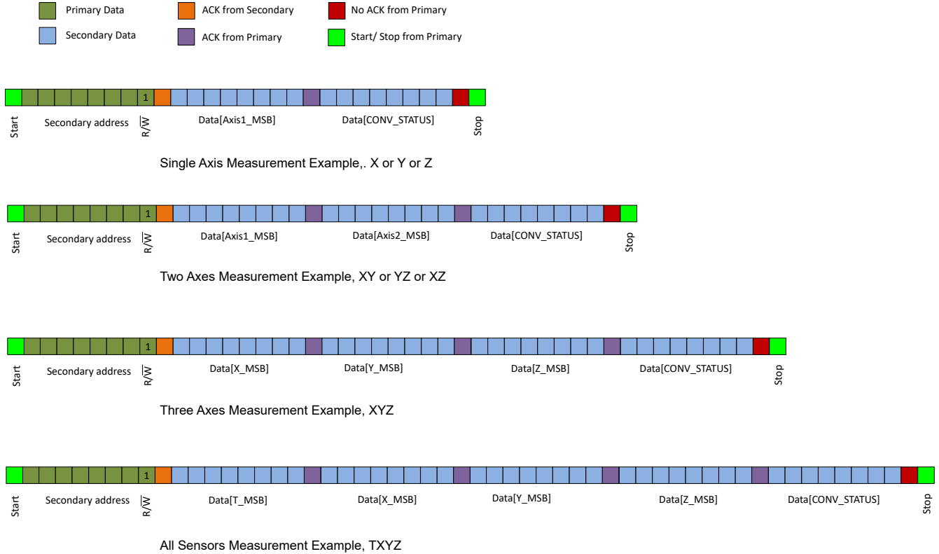
图 6-13. CRC 禁用且 CRC_EN = 0b 时 8 位数据的 1 字节 I 2 C 读取命令
