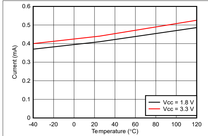
图 5-1. 待机模式 ICC 与温度间的关系
